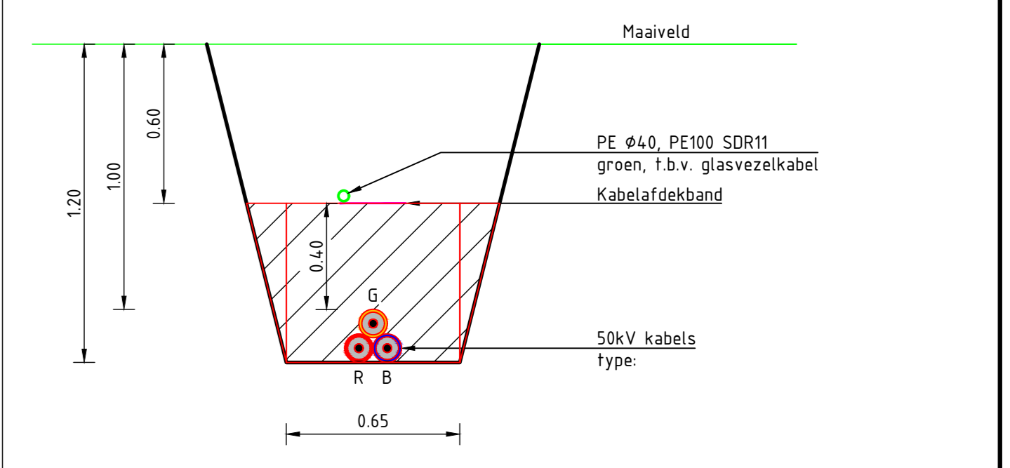
DWARSPROFIEL A-A SCHAAL 1 : 20
