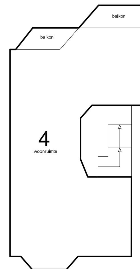
Derde verdieping schaal 1:100
