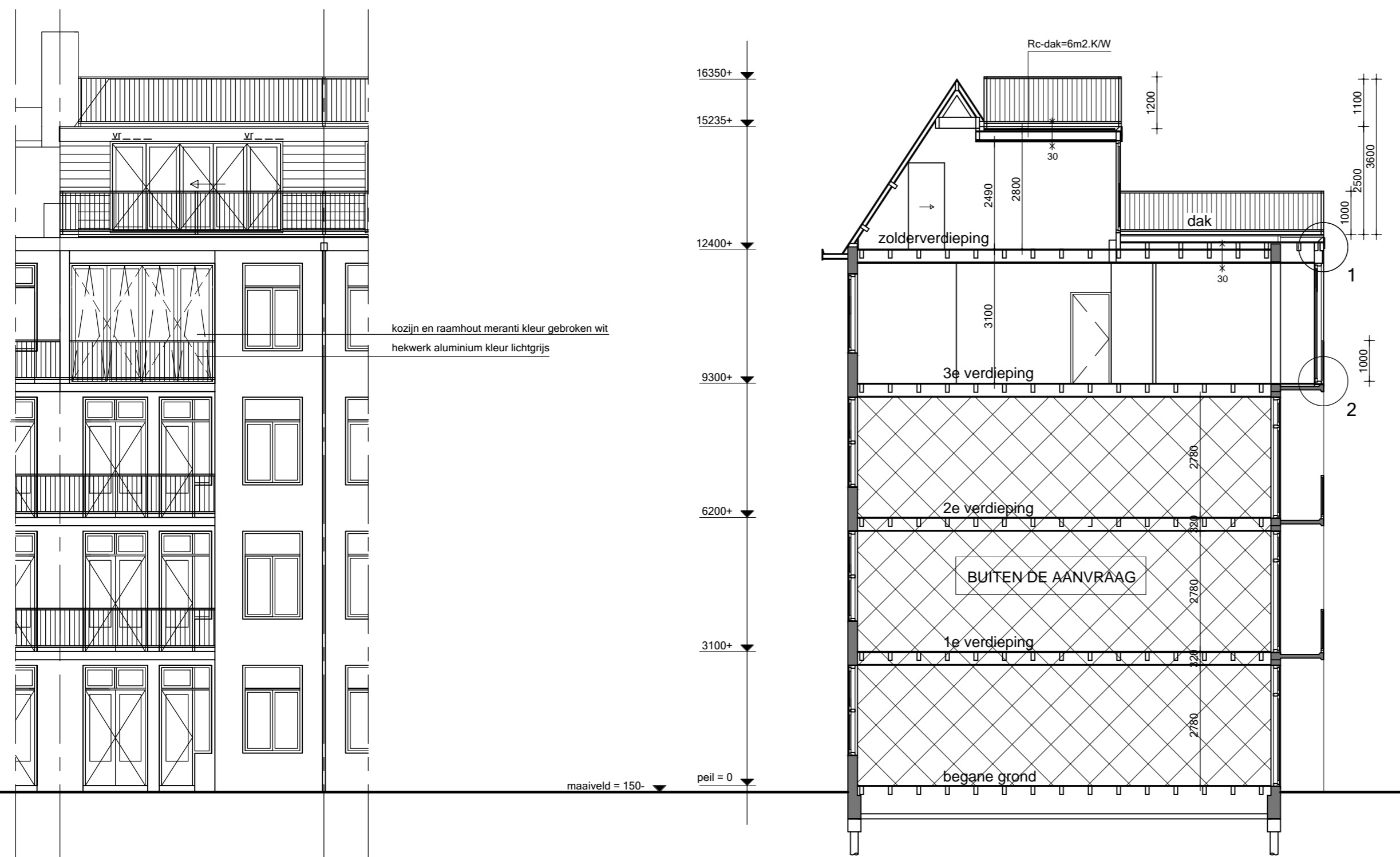
achtergevel
