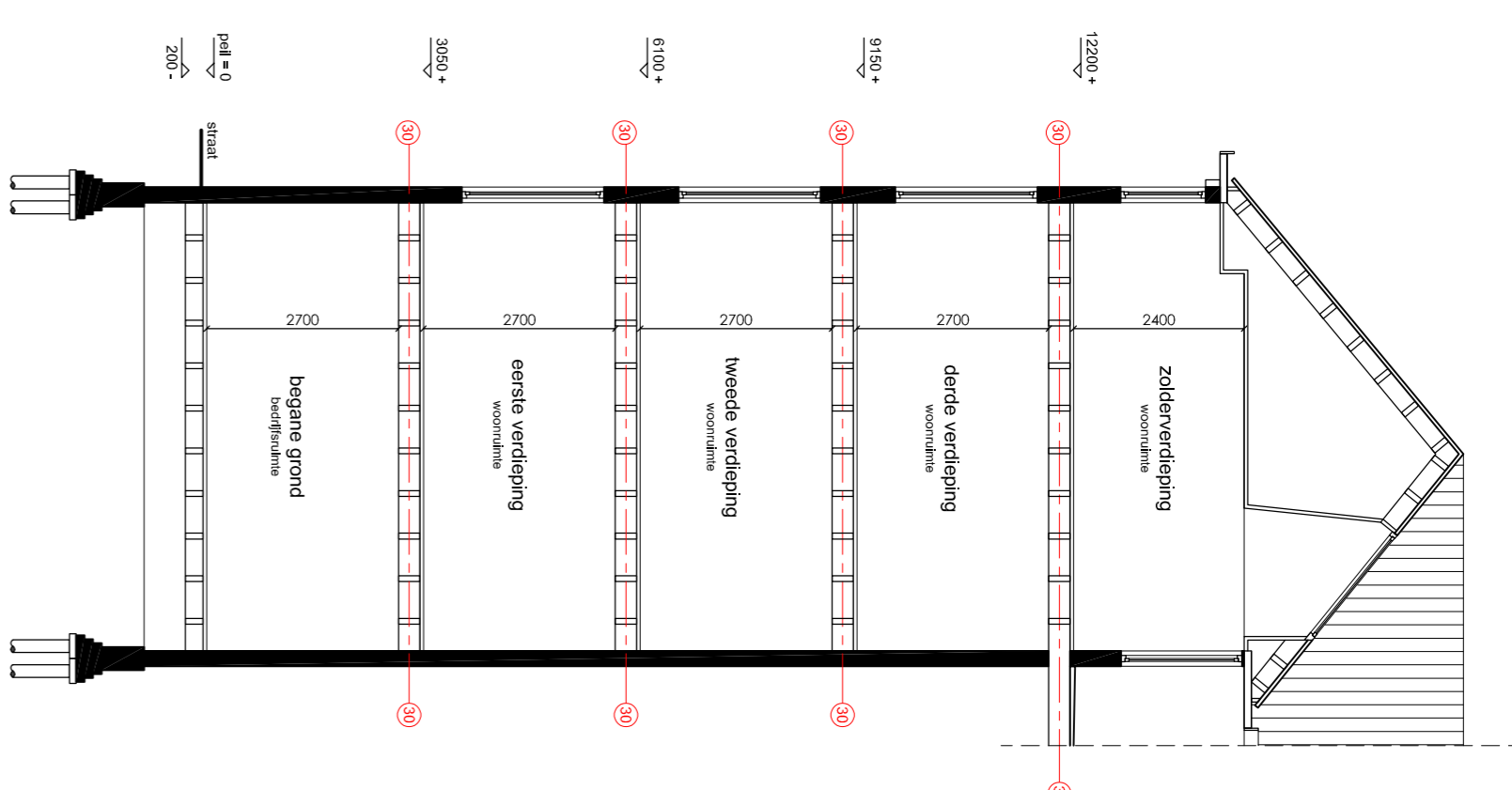
Doorsnede A-A
