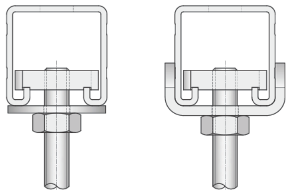
Afbeelding 4: Vergroot de stijfheid bij belasting onder de rail door gebruik te maken van U-vormige onderlegplaten (rechter afbeelding) in plaats van standaard platte onderlegplaten (linker afbeelding)
