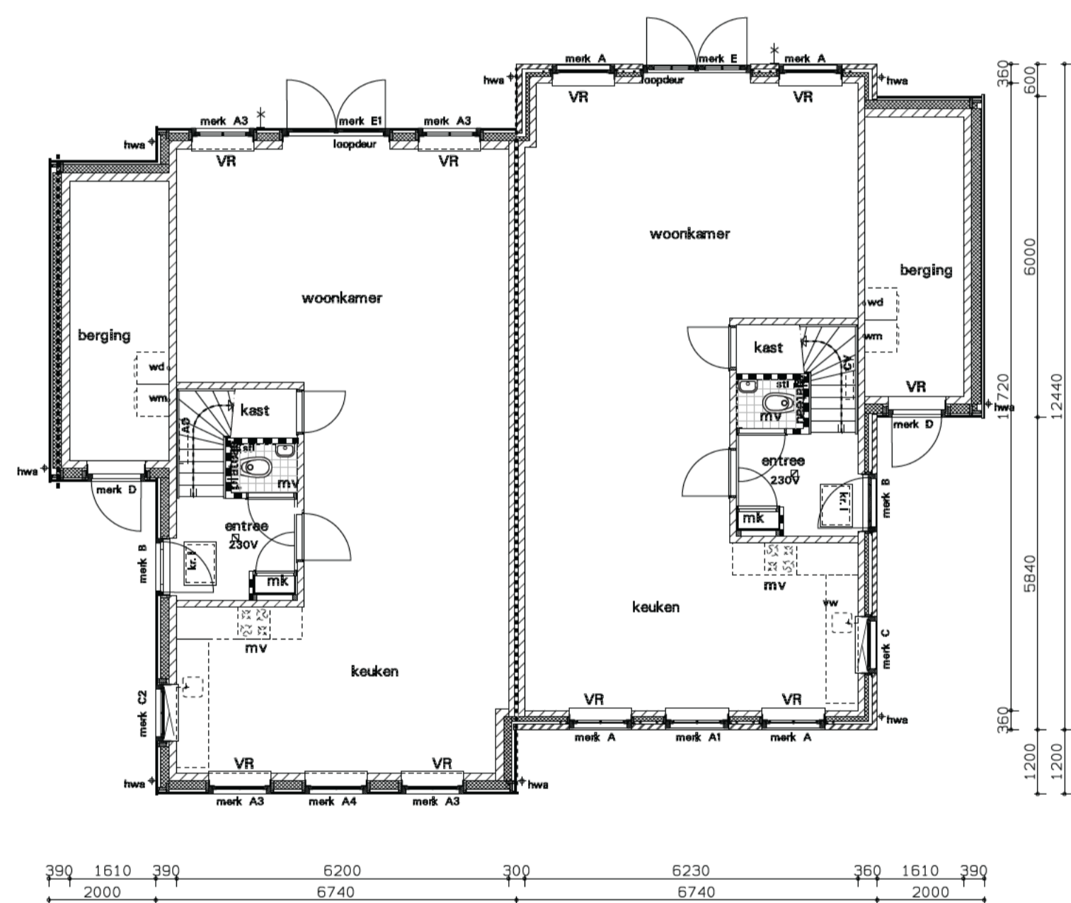
begane grond
