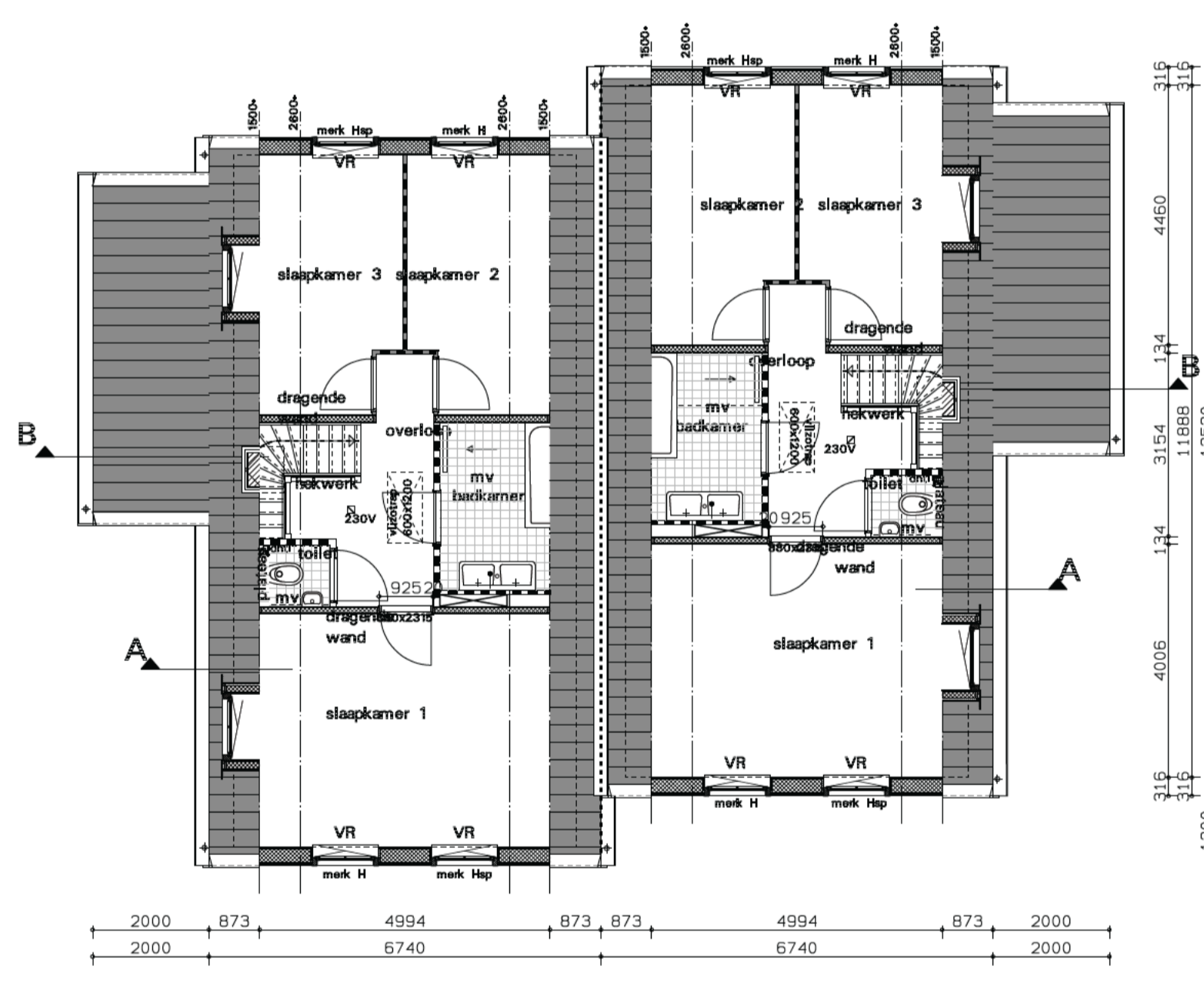
verdieping
