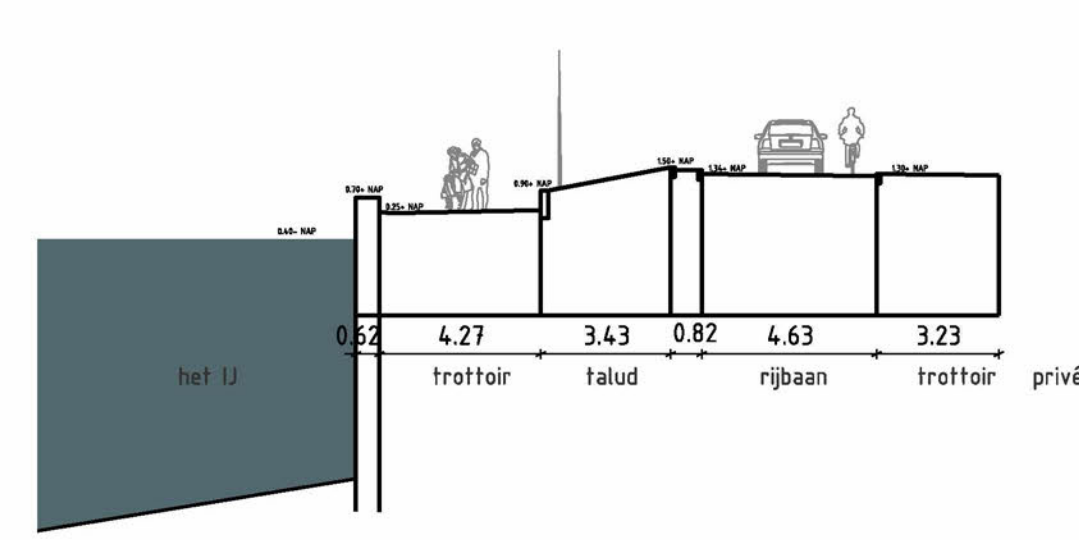
Profiel A
