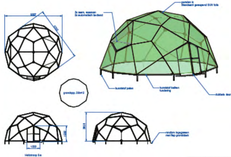
Tekening Kas
