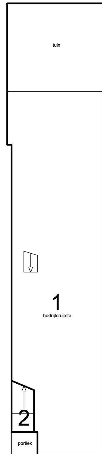
Begane grond schaal 1:100
