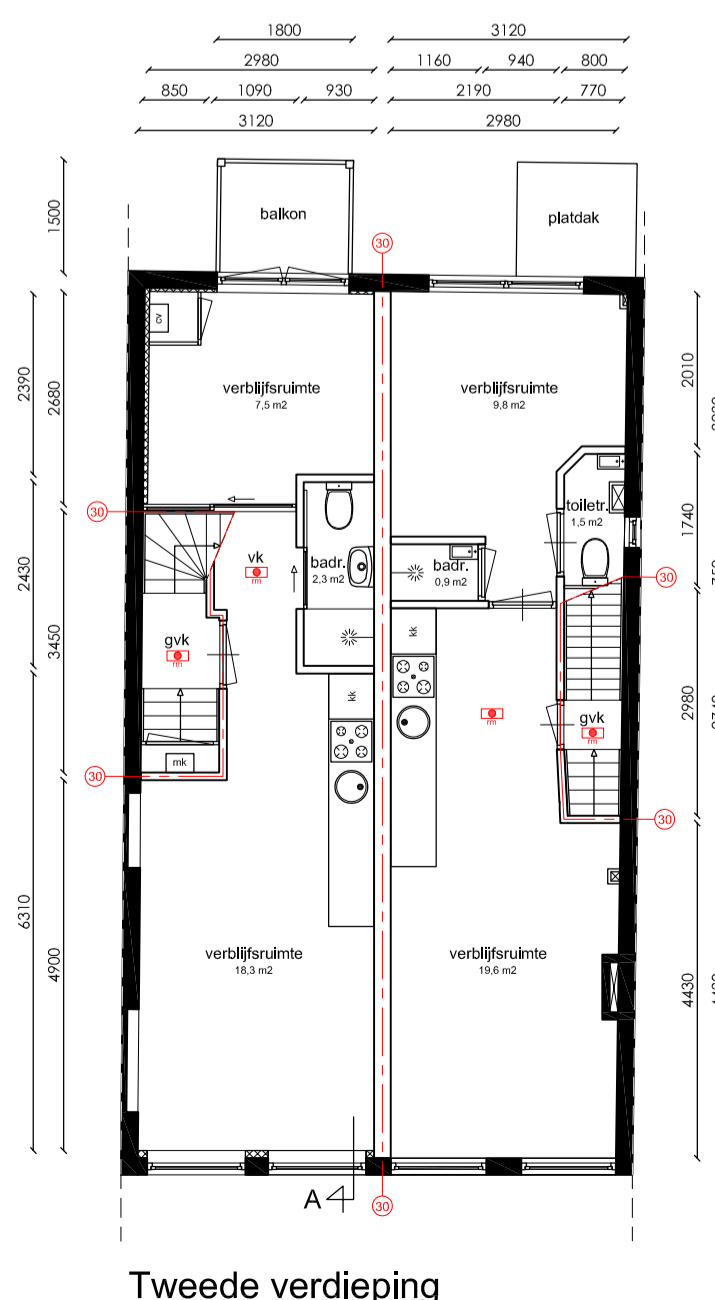
Tweede verdieping
