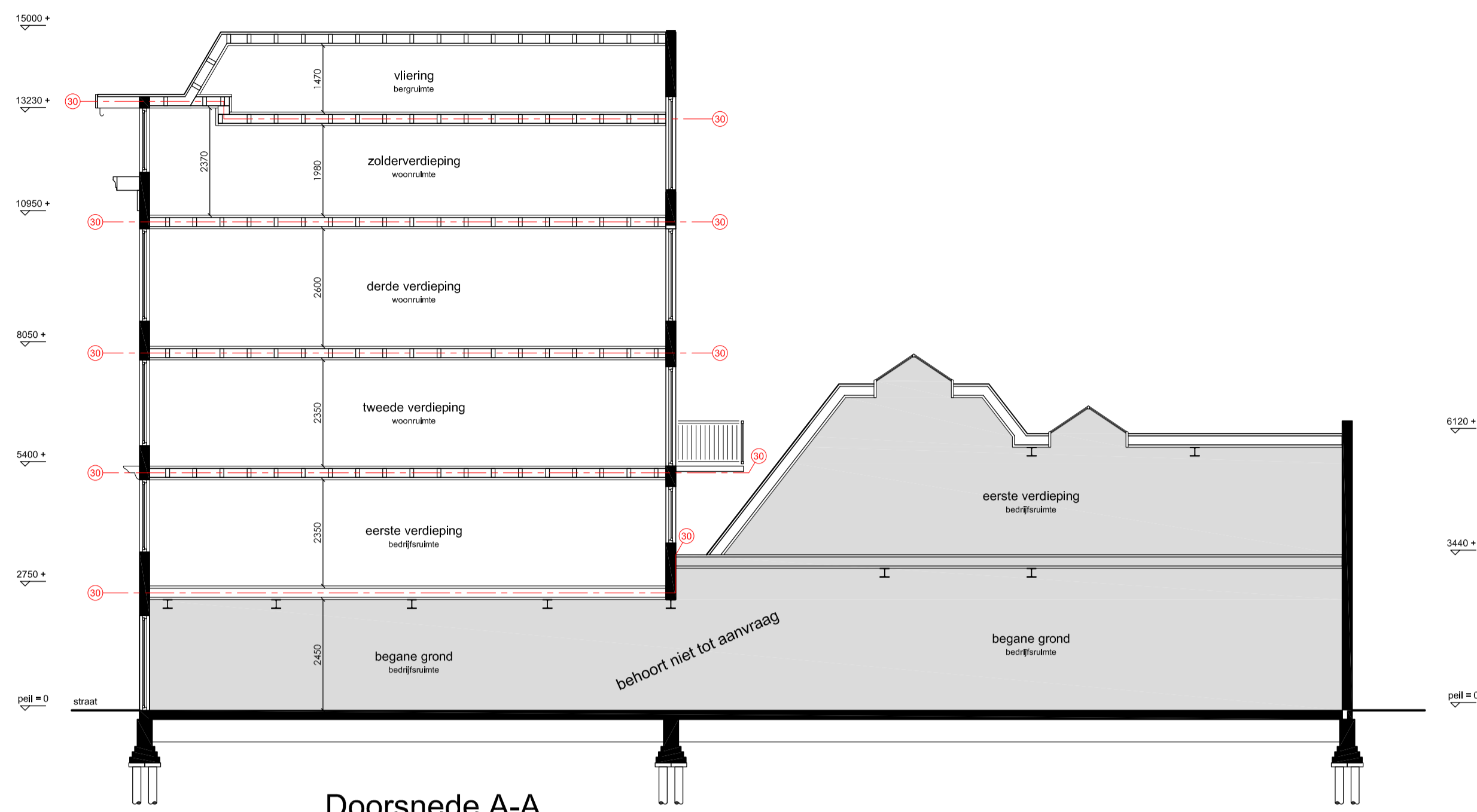
Doorsnede A-A
