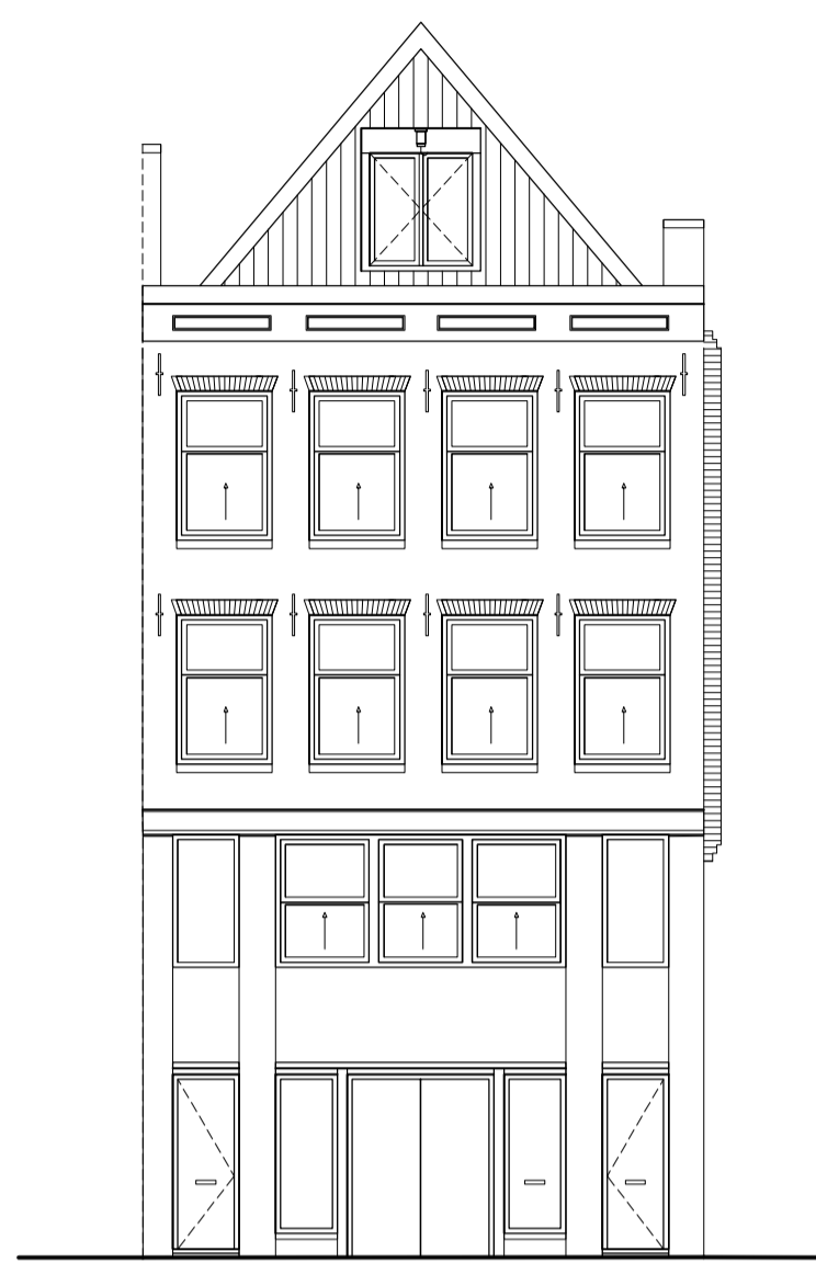
Voorgevel
