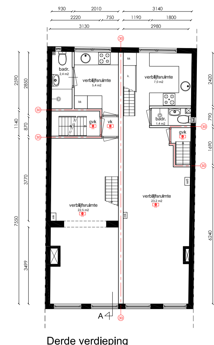
Derde verdieping
