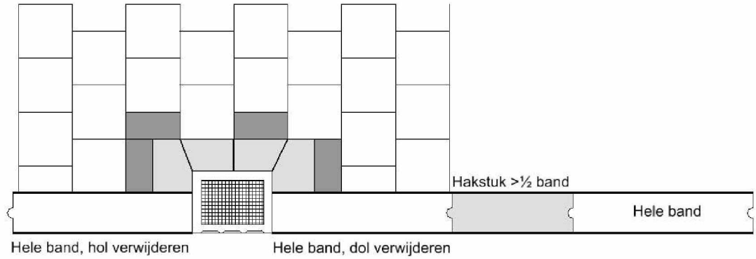
Detail hakwerk rond kolk
