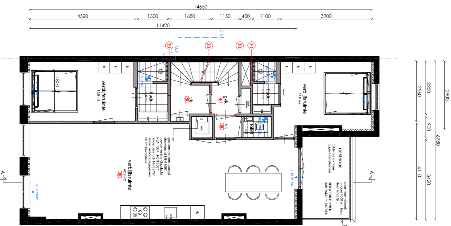
Derde verdieping Woonruimte GO = 77 m 2 / VG = 64 m 2
