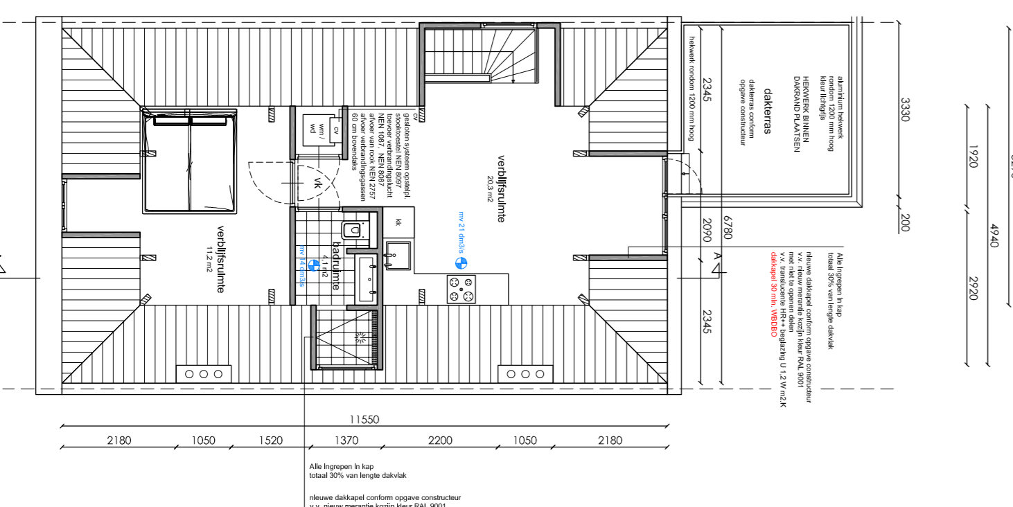
Zolderverdieping Woonruimte GO = 43 m 2 / VG = 32 m 2
