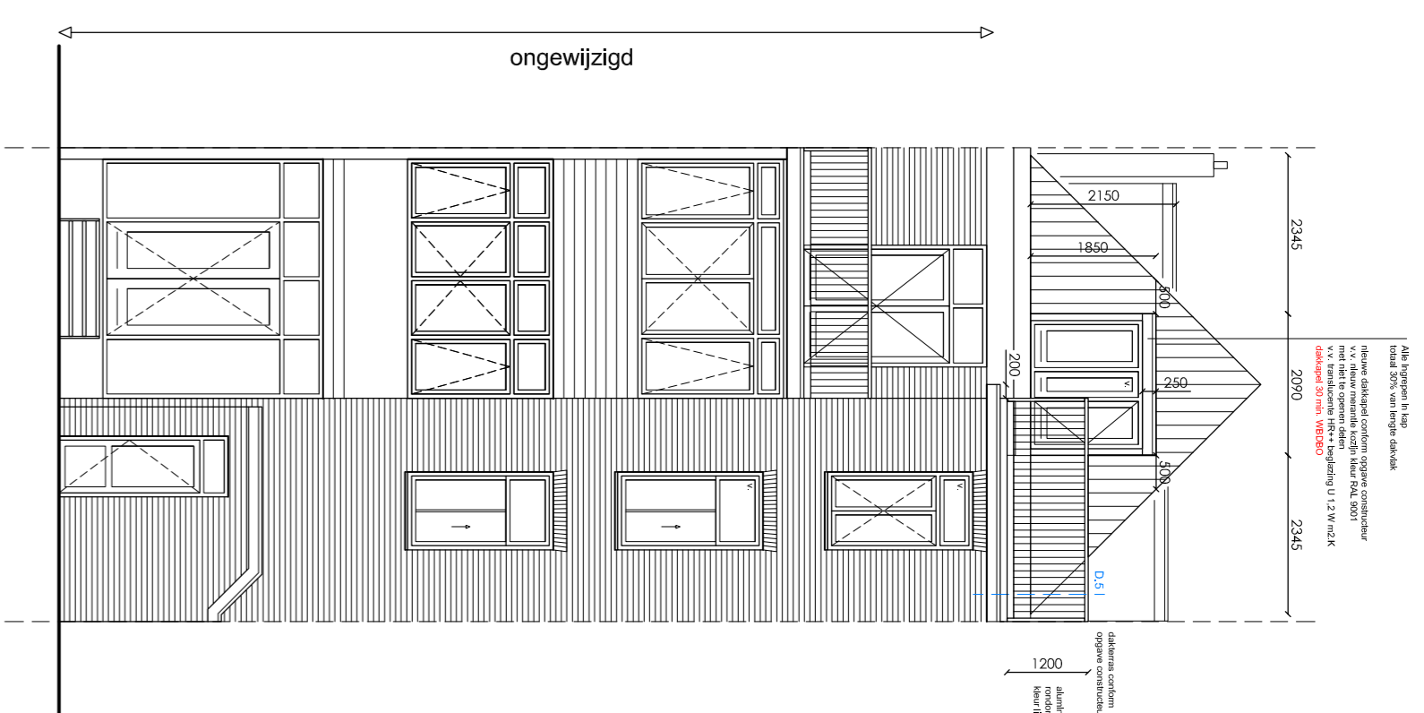
Achtergevel
