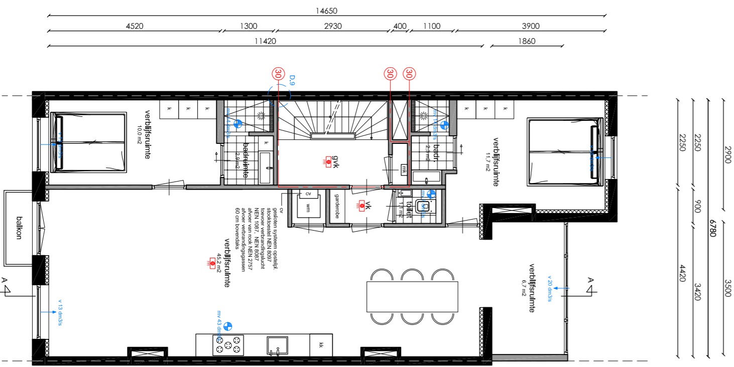
Tweede verdieping Woonruimte GO = 87 m 2 / VG = 71 m 2
