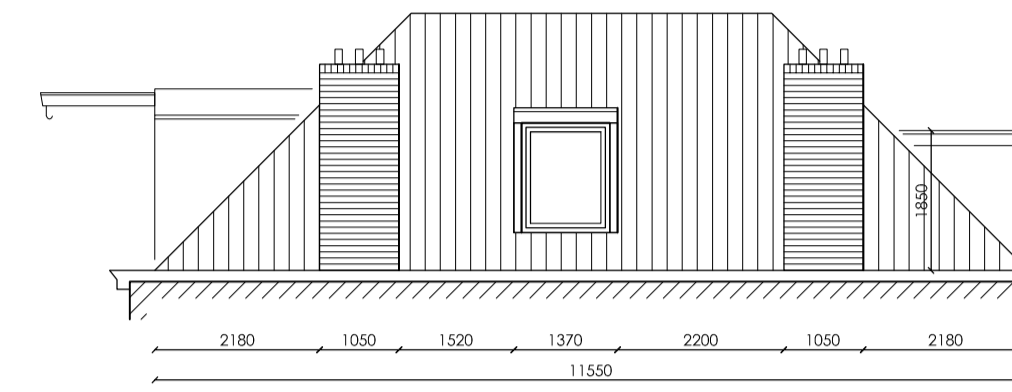
Rechter zijgevel
