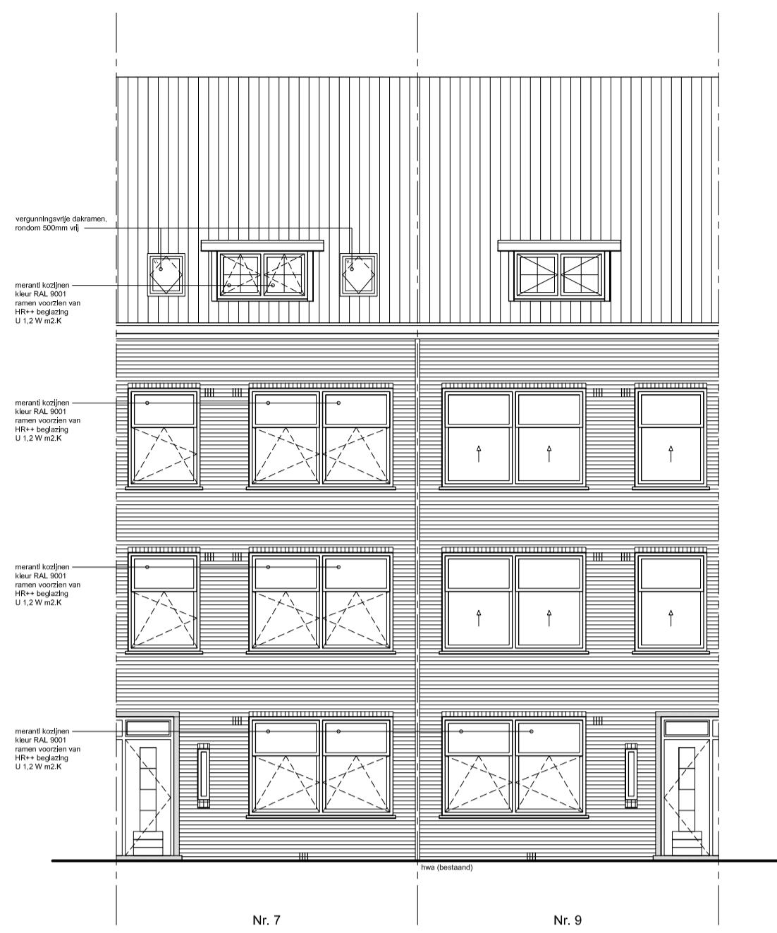
Voorgevel
