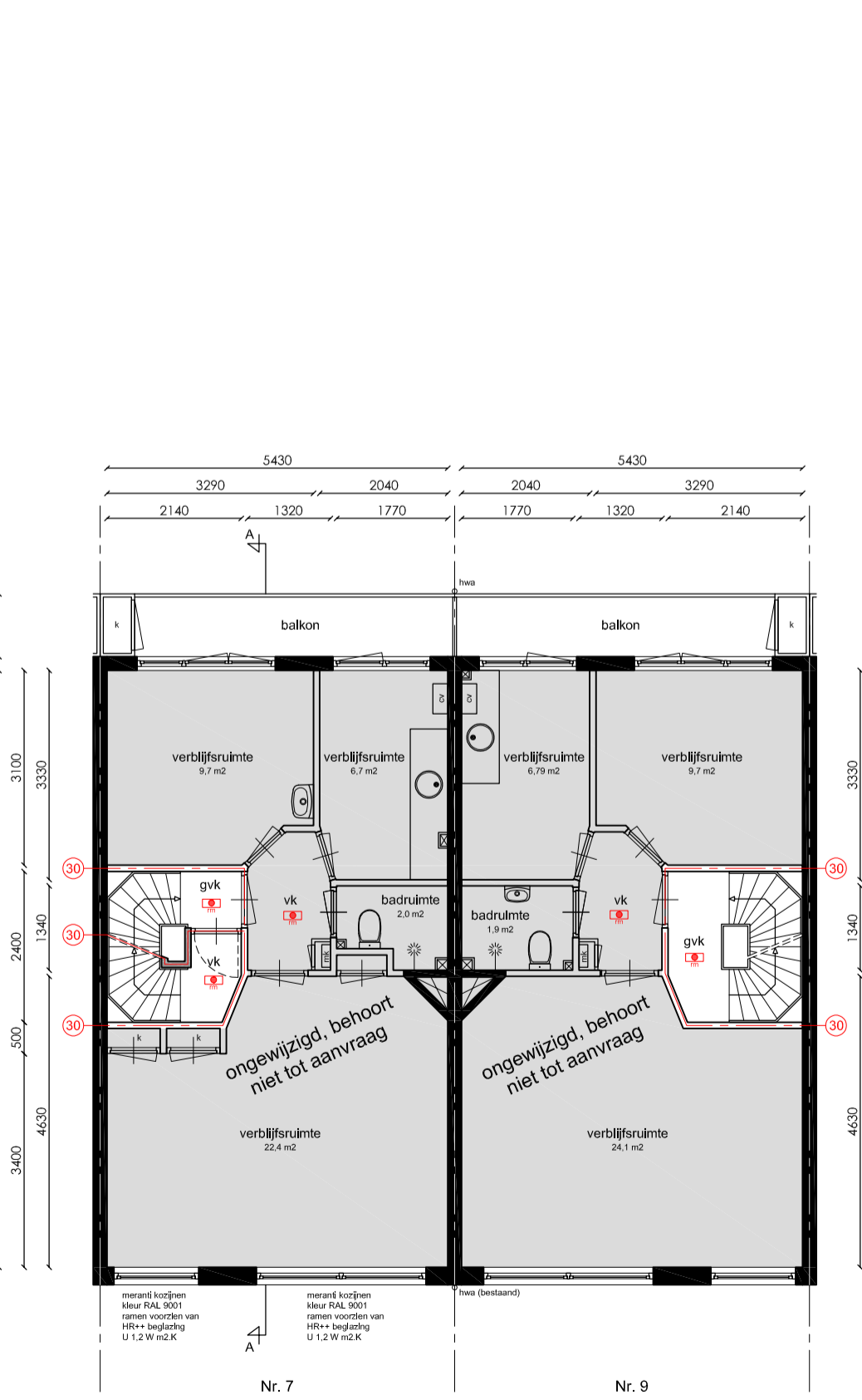
Tweede verdieping
