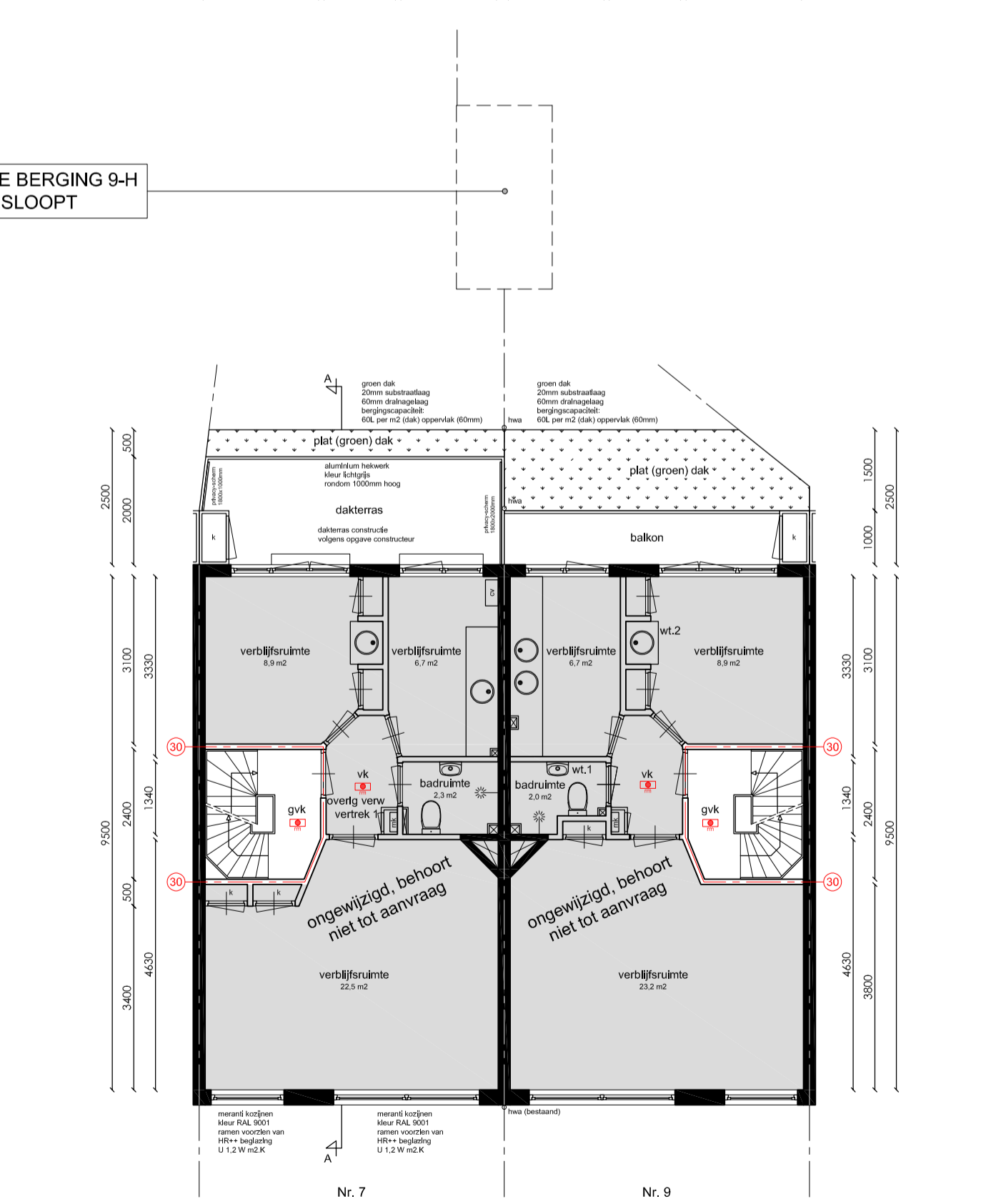
Eerste verdieping
