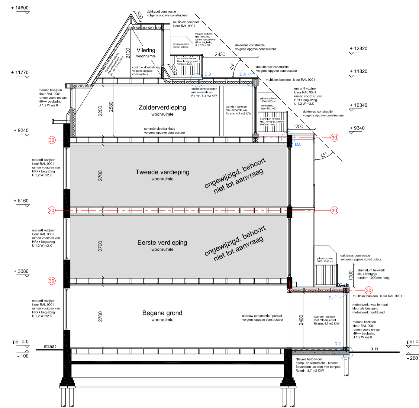
Doorsnede A-A
