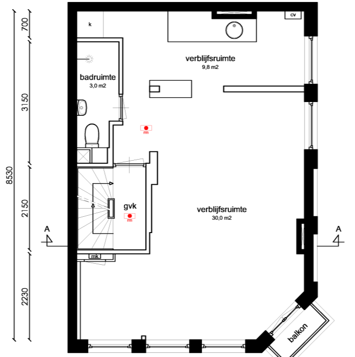
Eerste verdieping
