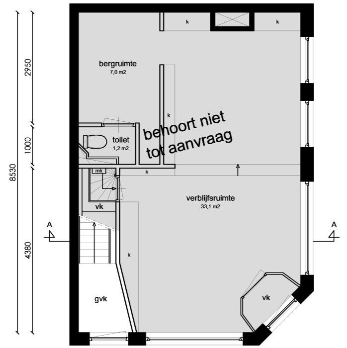
Begane grond
