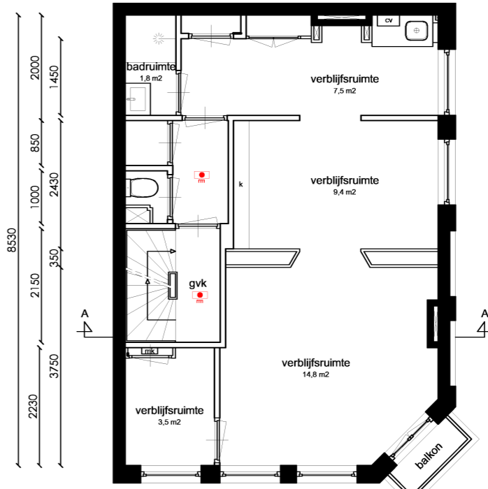
Derde verdieping
