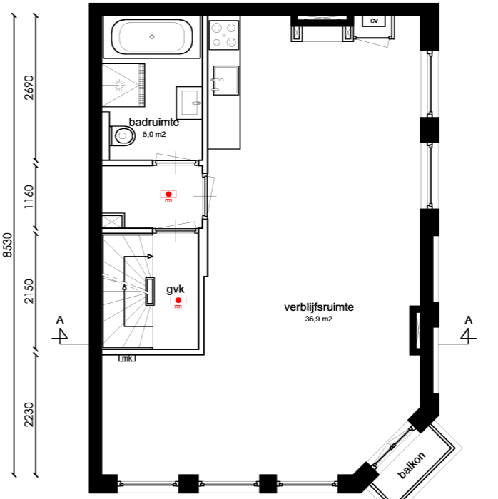
Tweede verdieping
