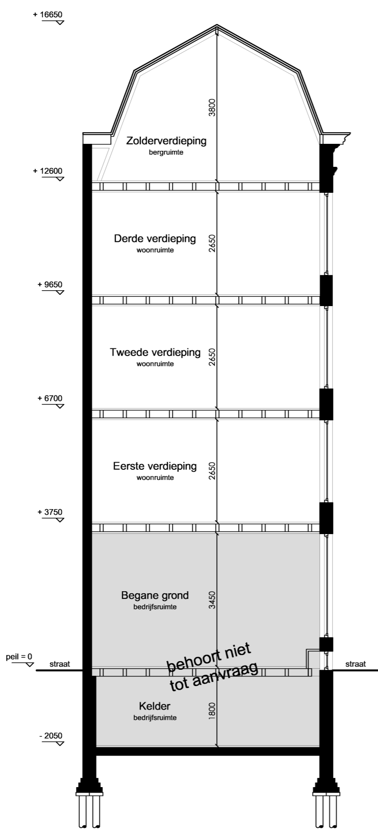
Doorsnede A-A
