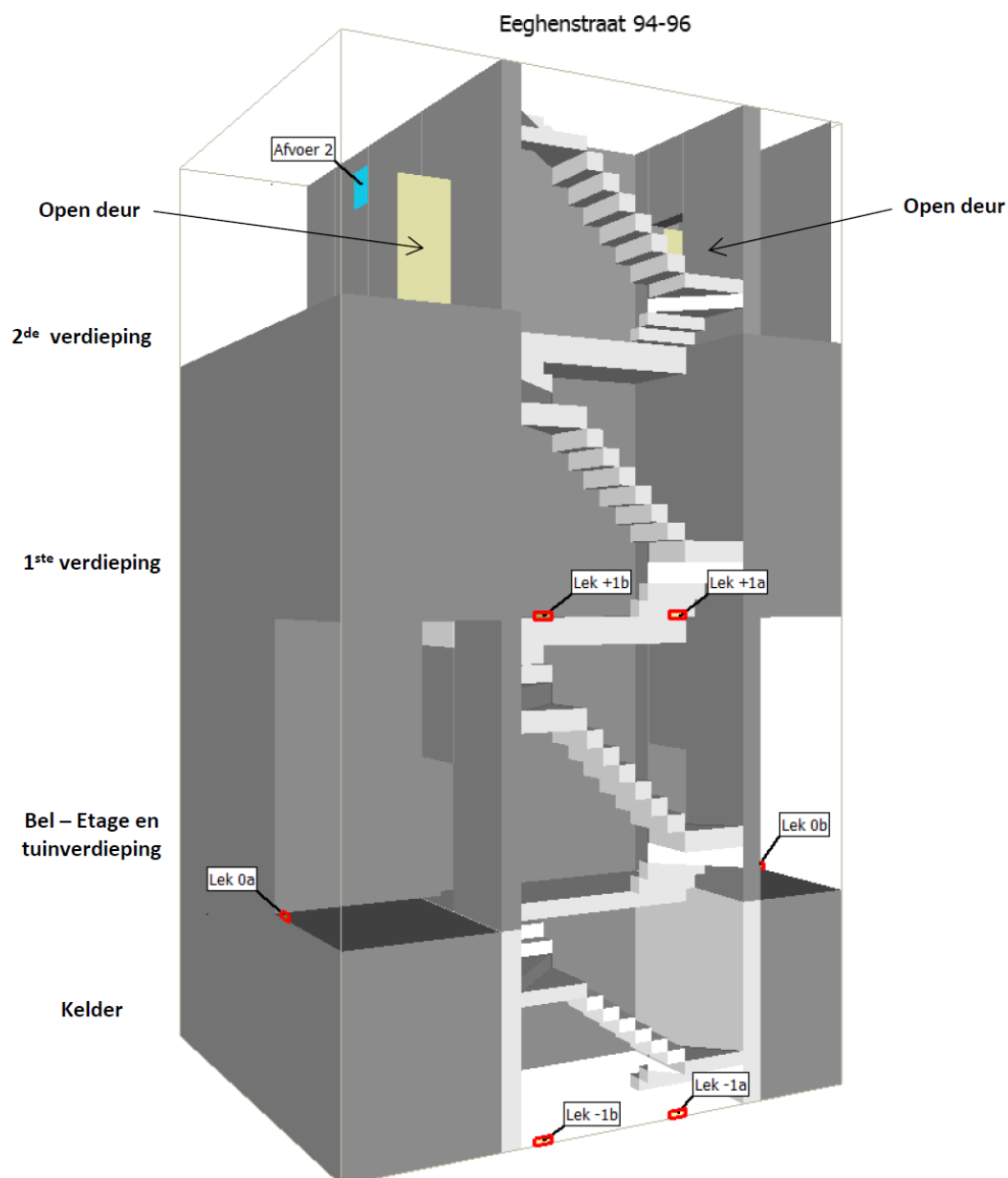
Figuur 2 – CFD-model
