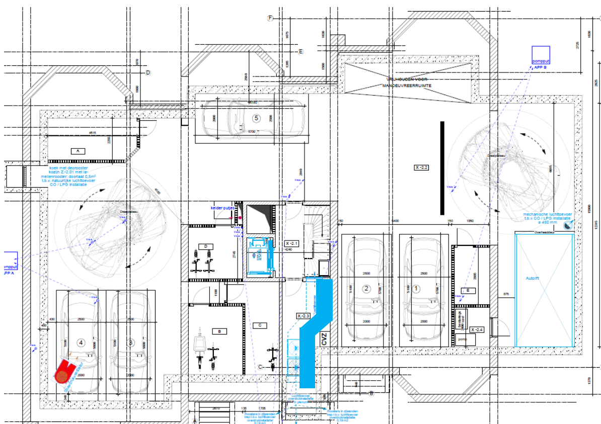
Schematische weergave luchttoevoervoorziening
