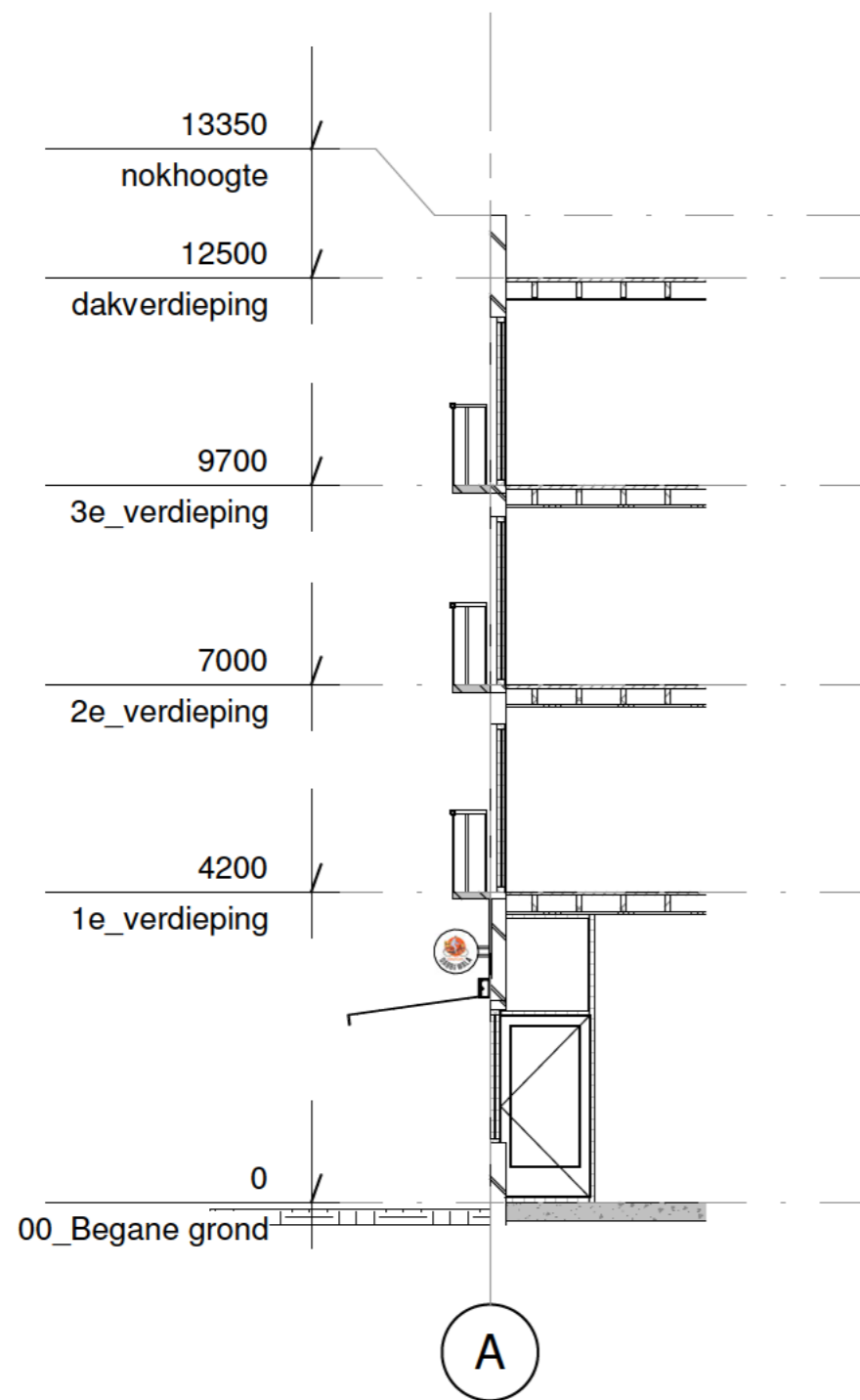
DWARS DOORSNEDE A-A(n)
