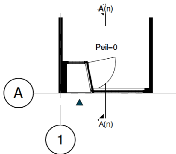
FRAGMENT PLATTEGROND BG
