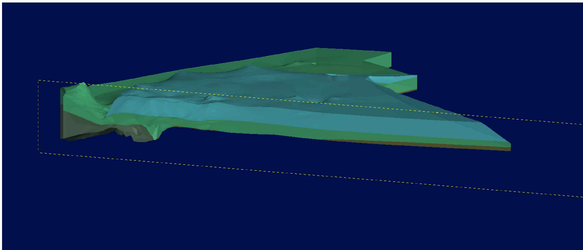
Figuur 4-7: Overzicht uit het 3D model (sluisbuurt doorsnede) met alle zettingsgevoelige lagen. De sliblaag is in het blauw weergegeven, gevolgd door de oude zeeklei en de hydrobia klei. Linksonder is de Oergeul in het donkergroen zichtbaar.
