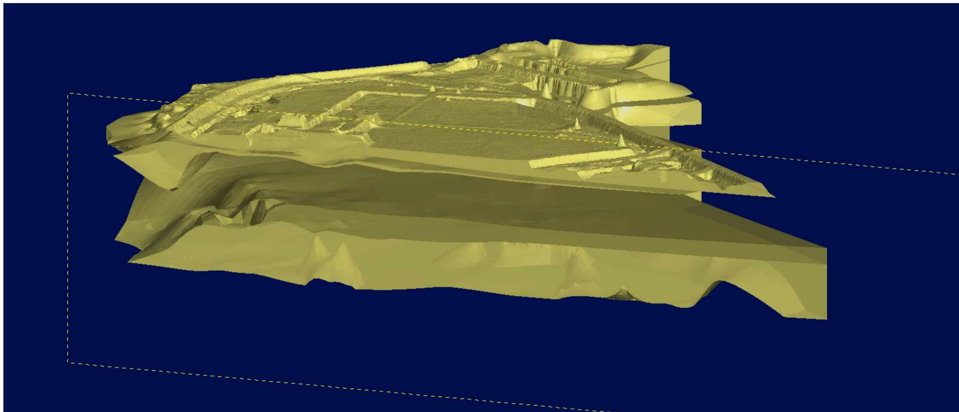
Figuur 4-6: Overzicht uit het 3D model (sluisbuurt doorsnede) met alle zandlagen weergegeven. (De opgehoogde zandlaag, de zandlaag van de oude ophoging, de 1 ste zandlaag en de 2 de zandlaag) De 2 de zandlaag is over het algemeen geschikt als funderingsniveau. Bij de Oergeul locatie ontbreekt deze laag lokaal volledig.
