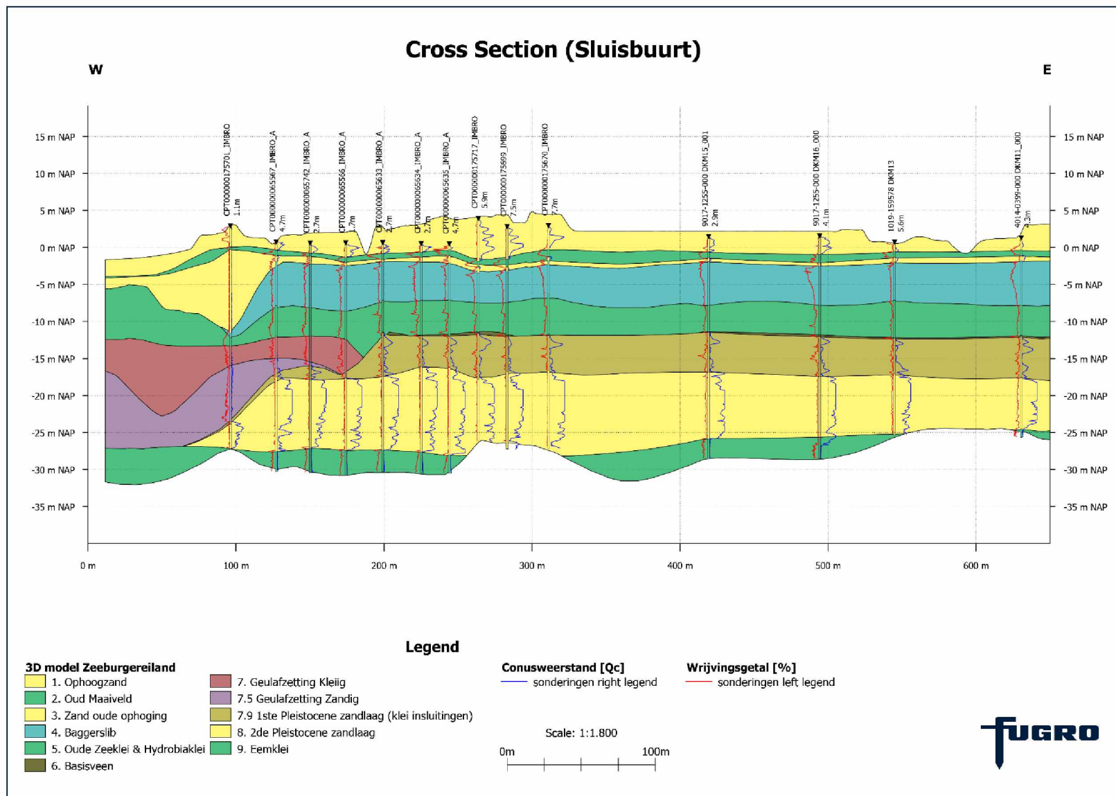
Figuur 4-4: Doorsnede (Sluisbuurt) met daarin verschillende sondeerpunten (binnen 10 m van de doorsnedelij) met conusweerstand en toegekende grondlagen.
