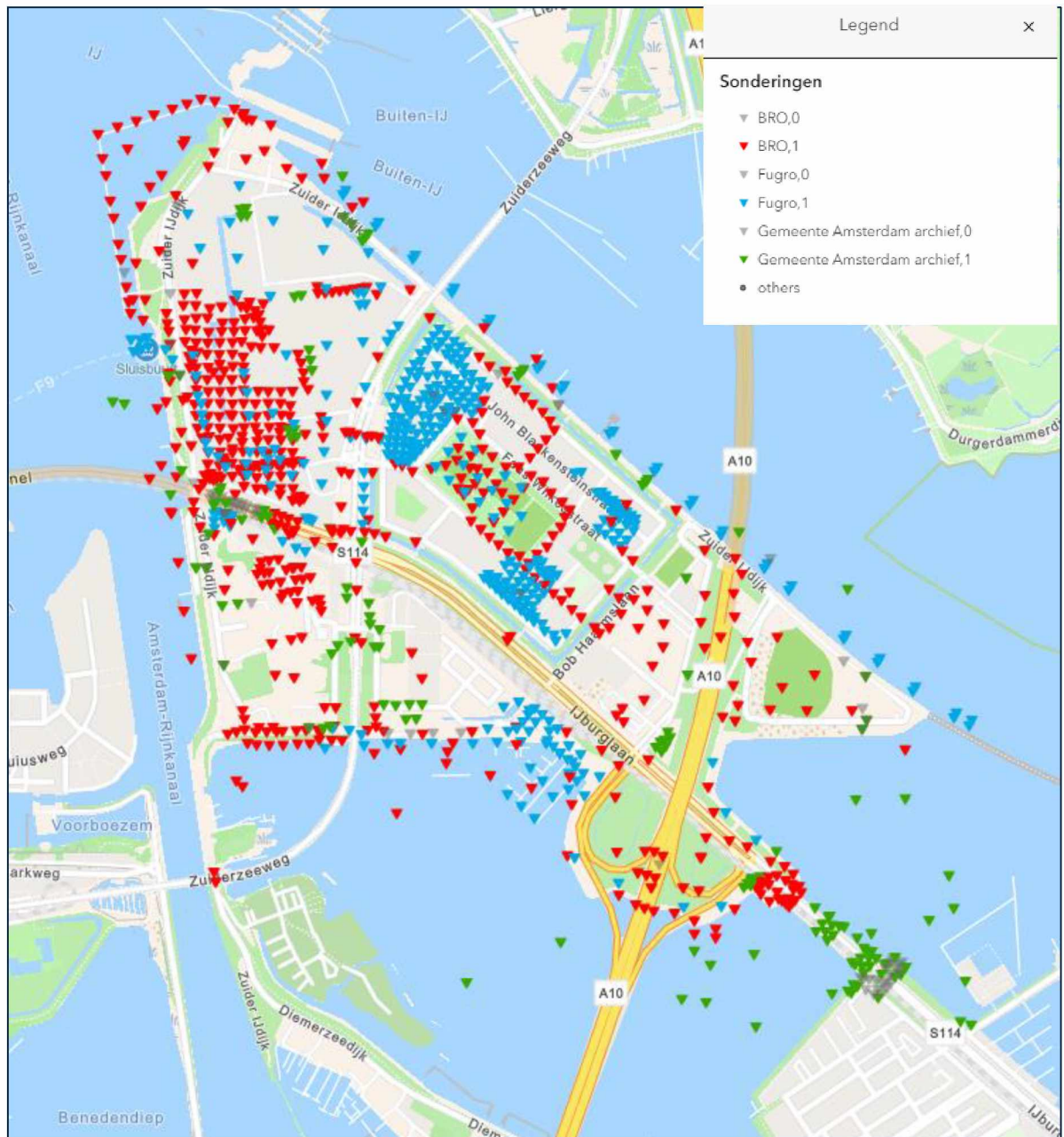
Figuur 3-2: Overzicht gebruikte sonderingen uit openbare archief BRO (rood), archief Fugro (blauw) en archief gemeente Amsterdam (groen)
