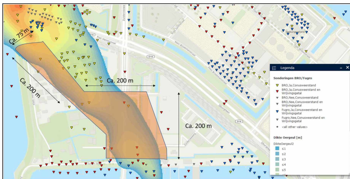
Figuur 6-3: Zoom-in Baai buurten met een indicatie van te onderzoeken oppervlakte van de Oergeul voor het maken van inschatting aanvullende sonderingen.
