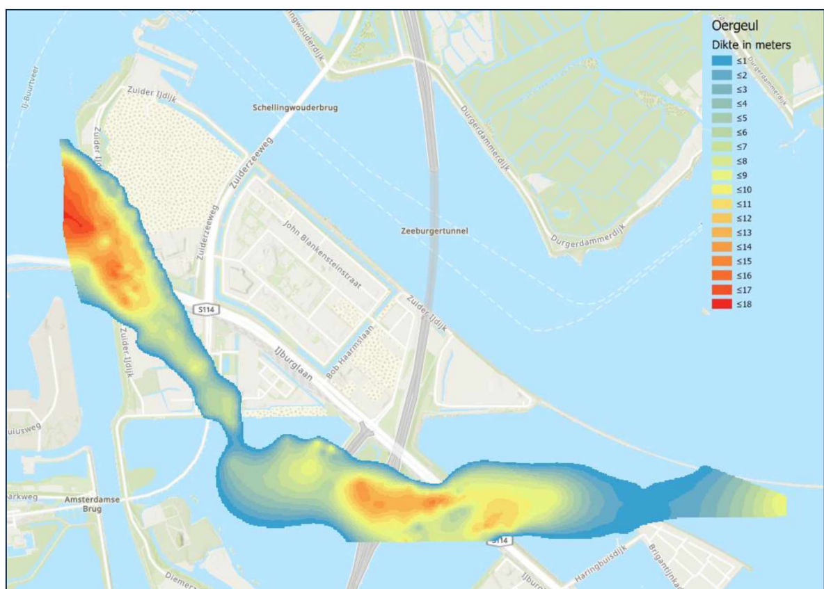
Figuur 5-1: Locatie en dikte Oergeulafzettingen in meters
