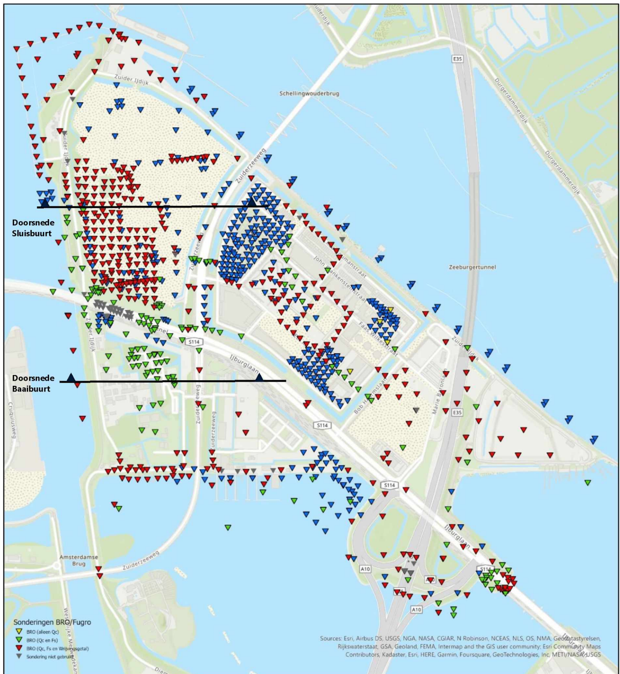
Figuur 4-3: Overzicht Zeeburgereiland, sondeerlocaties (rode punten zijn sonderingen uit BRO-loket en blauwe sonderingen zijn sonderingen uit Fugro archief.), en ondergrond doorsneden van de Sluis- en Baibuurt. Zie Figuur 4-4 en Figuur 4-5
