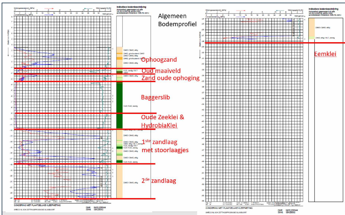
Figuur 3-4: Algemeen bodemprofiel Zeeburgereiland (Sluisbuurt) buiten de Oergeul
