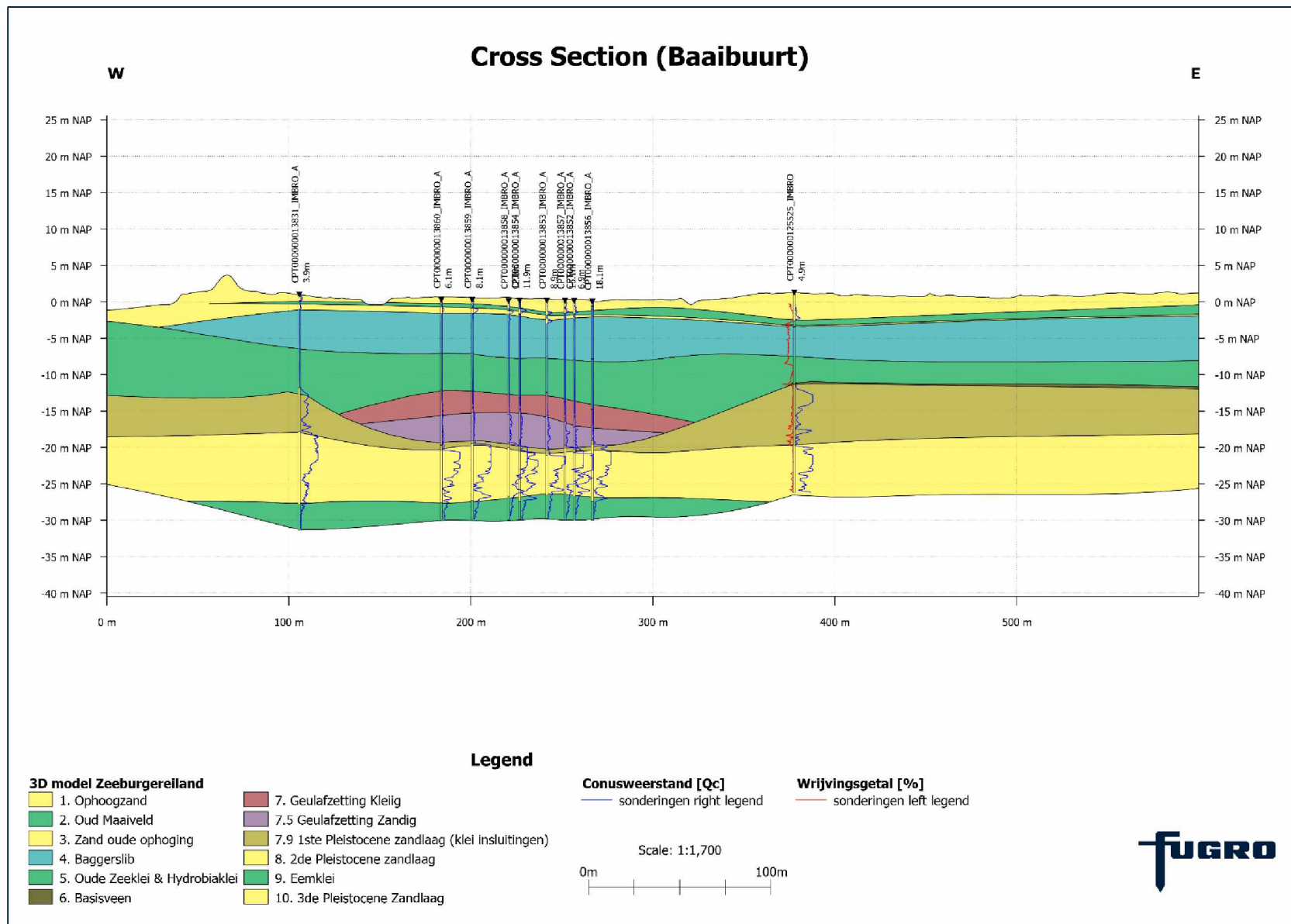
Figuur 4-5: Doorsnede (Baibuurt) met daarin verschillende sondeerpunten (binnen 50 m van de doorsnedelij) met conusweerstand en toegekende grondlagen
