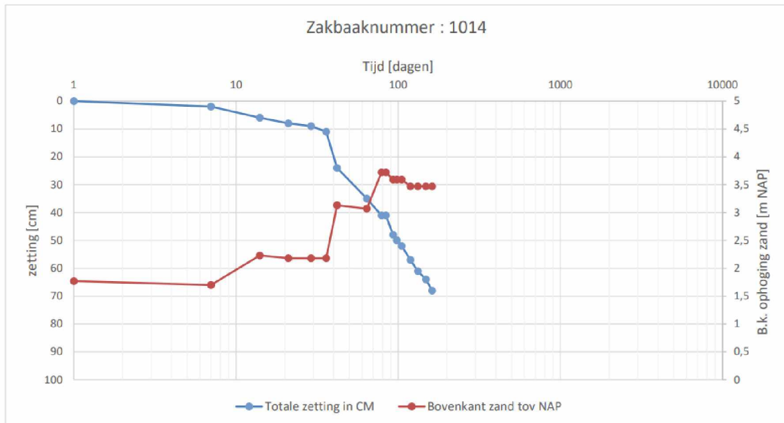
Figuur 5-3: Voorbeeld monitoringsdata van zakbaak 1014 (Sluisbuurt te bouwcluster 5)
