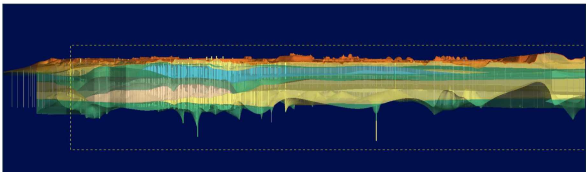
Figuur 4-2: Doorsnede 3D model ZBE met onderzoeklocaties en interpolatie van ondergrondlagen
