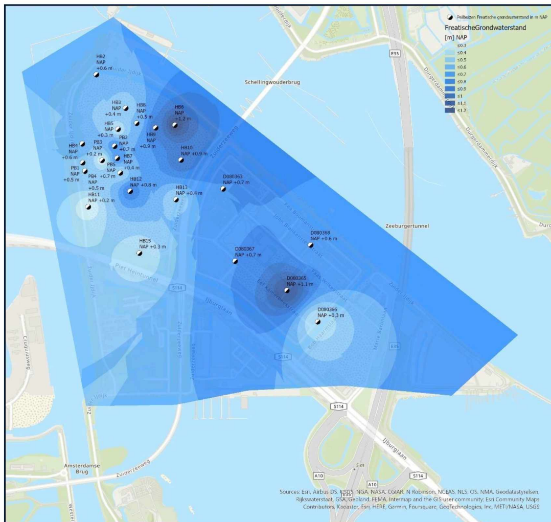
Figuur 3-6: Overzicht freatische grondwaterstand Zeeburgereiland.
