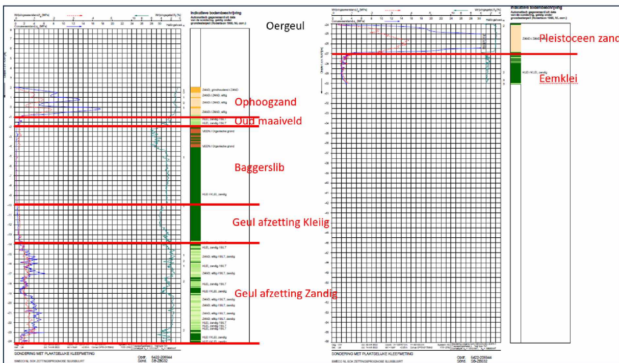
Figuur 3-5: Bodemprofiel (Sluisbuurt) binnen de Oergeul.
