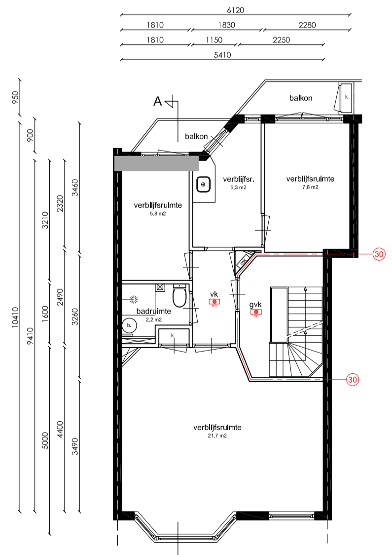
Tweede verdieping
