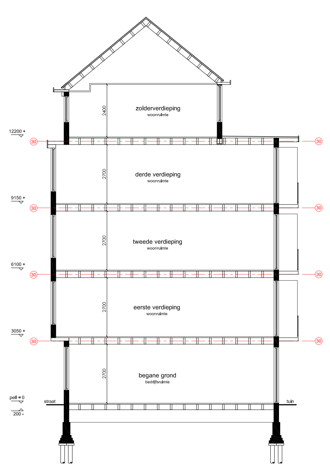
Doorsnede A-A
