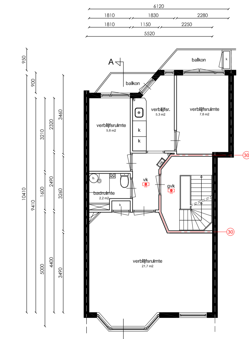
Derde verdieping
