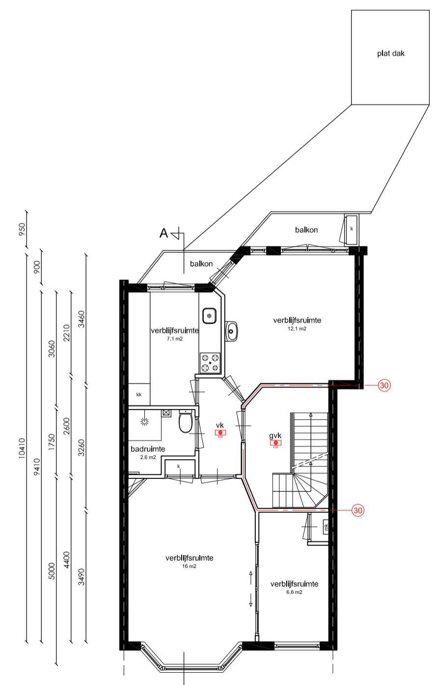
Eerste verdieping
