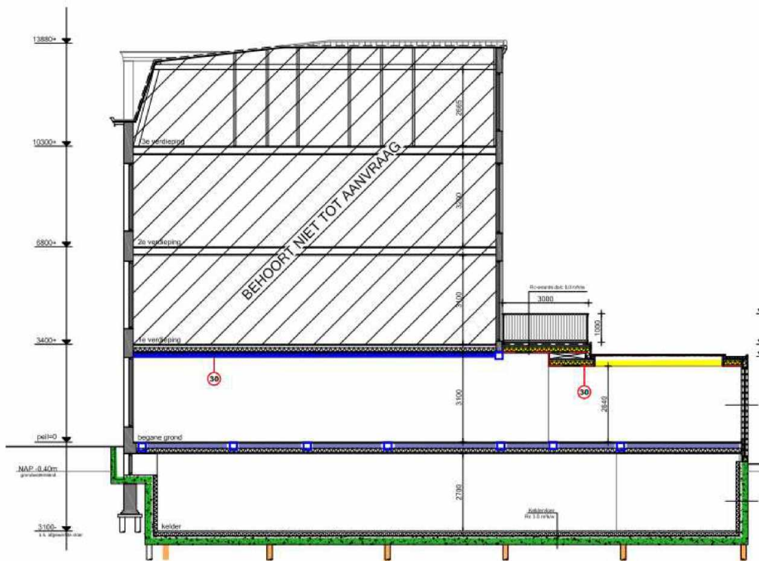
Doorsnede B-B
