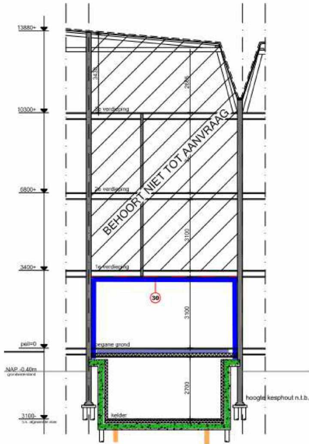
Doorsnede A-A
