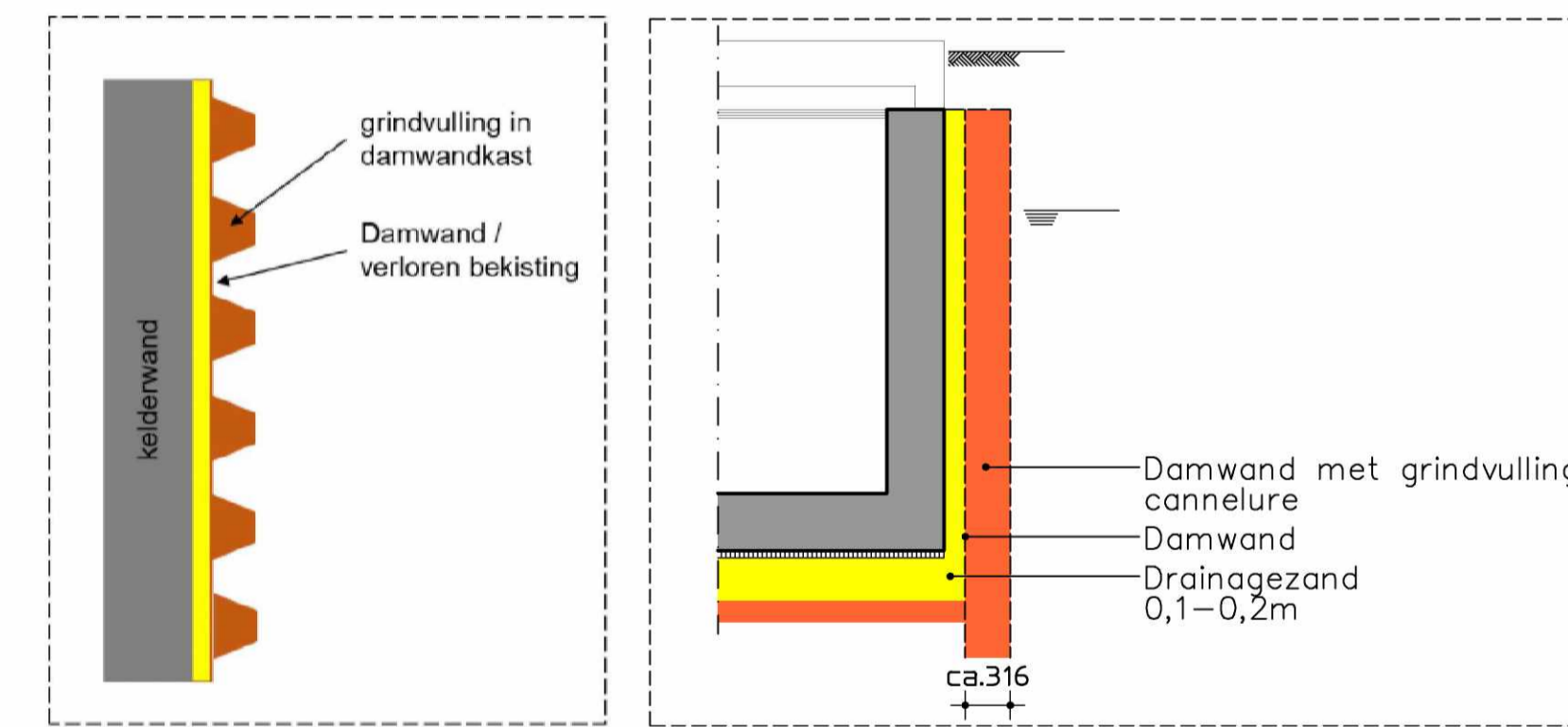
schematisch bovenaanzicht maatregel opvulling cannelures
