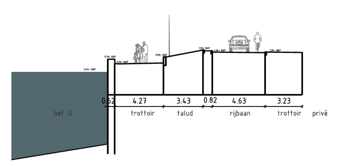
Profiel A
