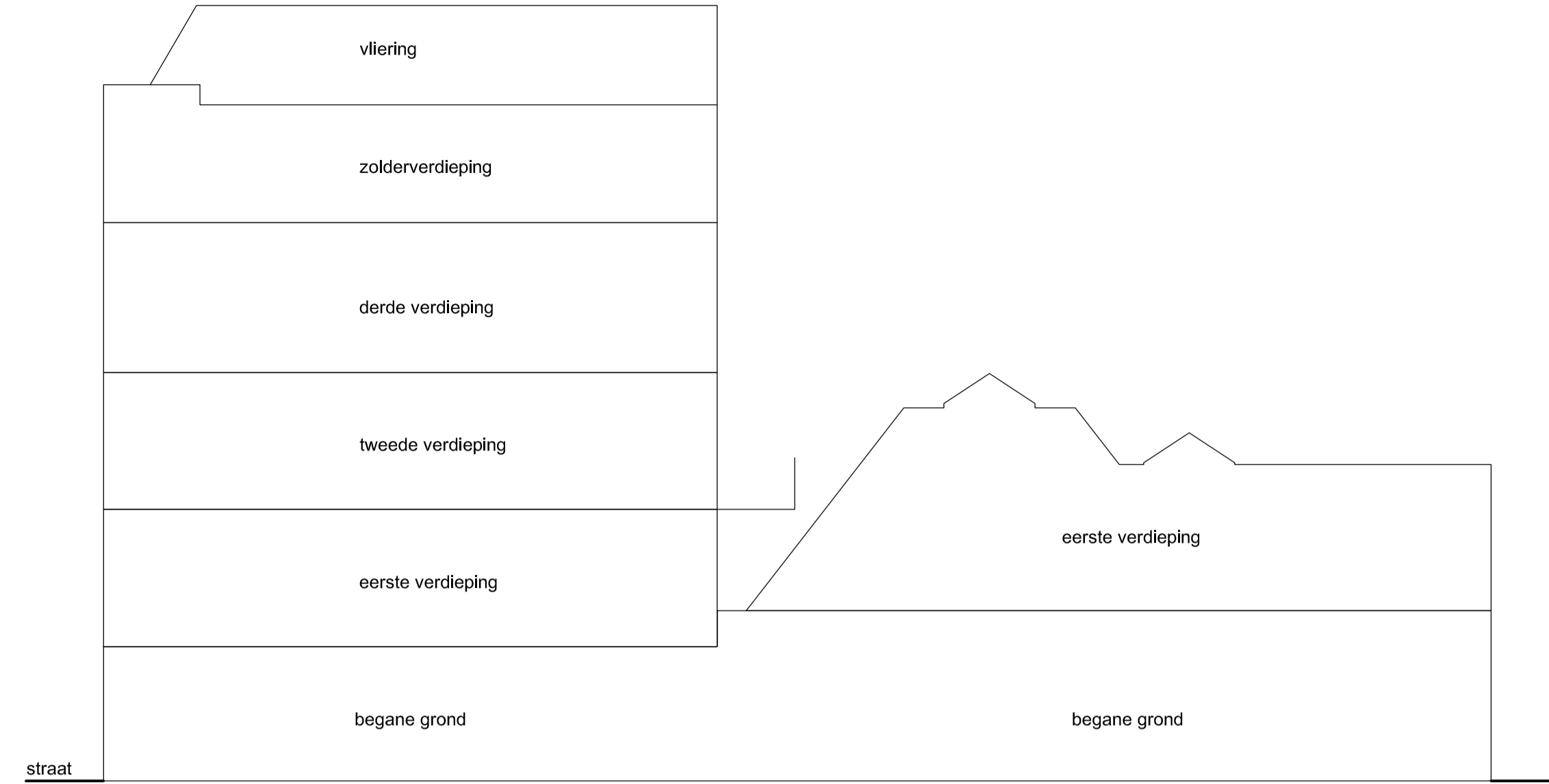
Doorsnede schaal 1:100
