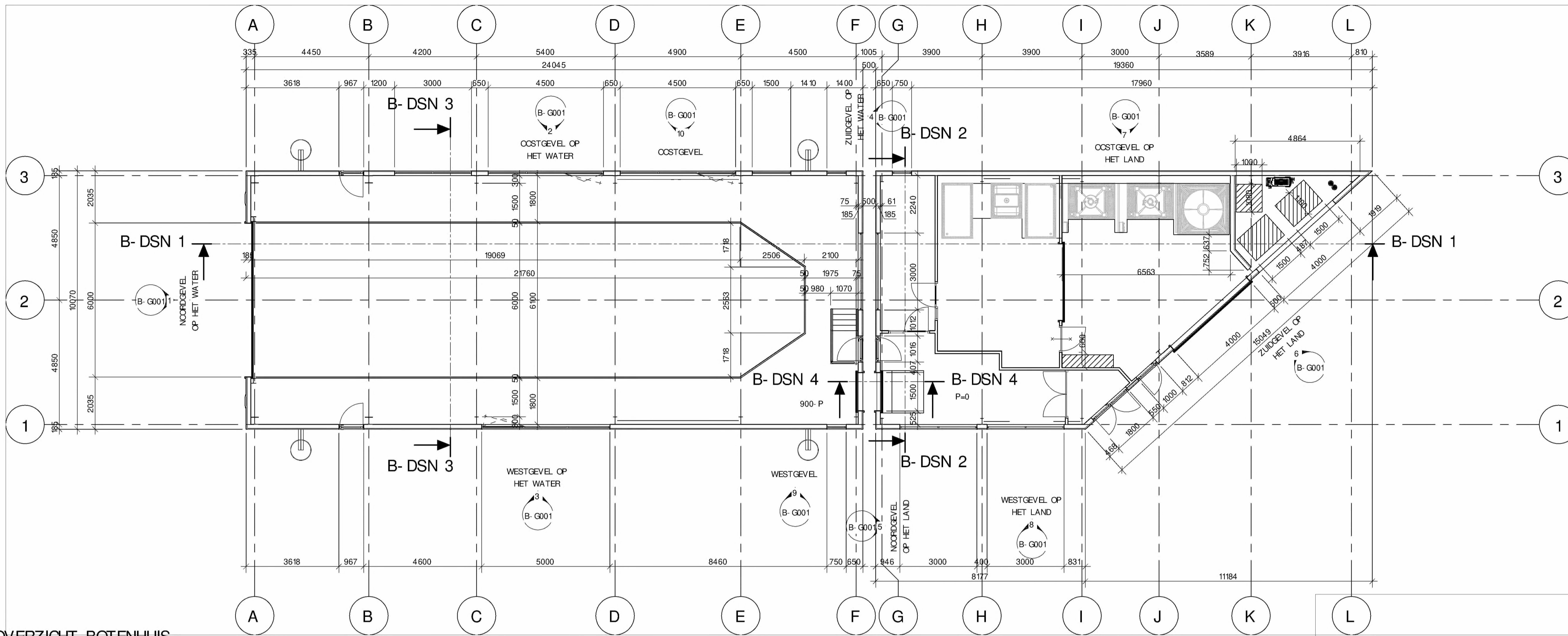
OVERZICHT BOTENHUIS schaal: 1 : 100
