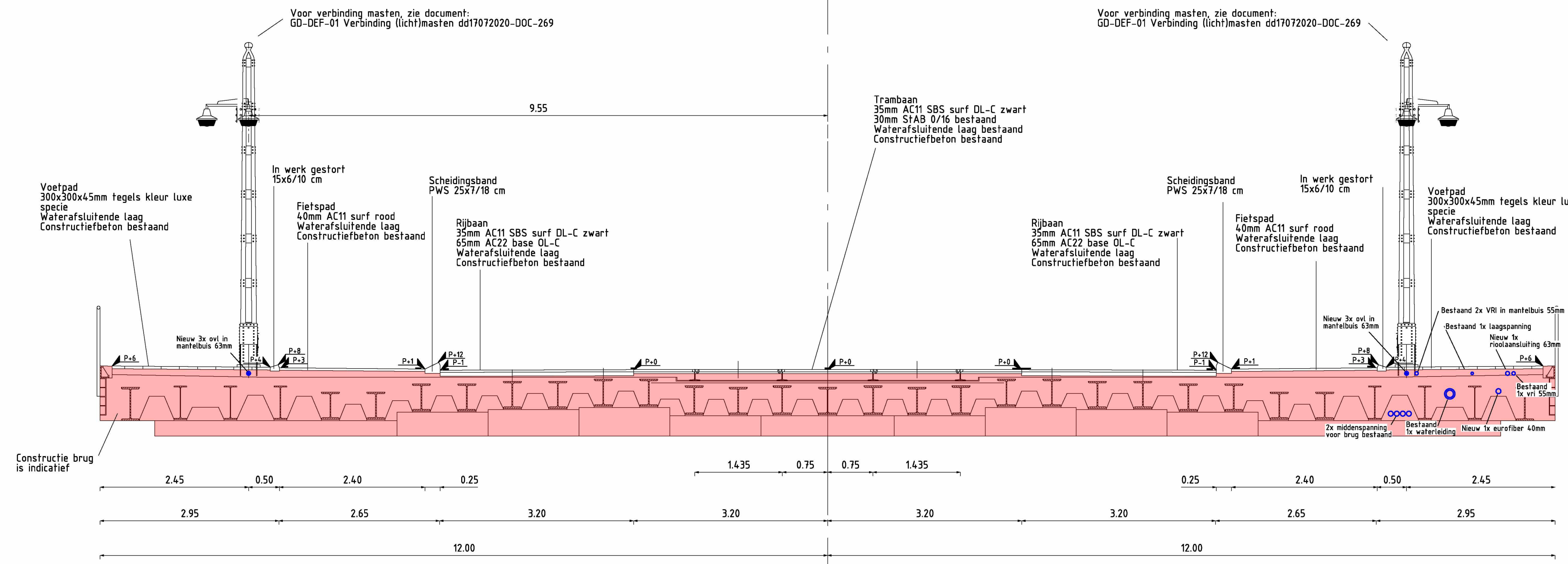
Dwarsprofiel A-A op aanbrug Nieuwe situatie schaal 1:50
