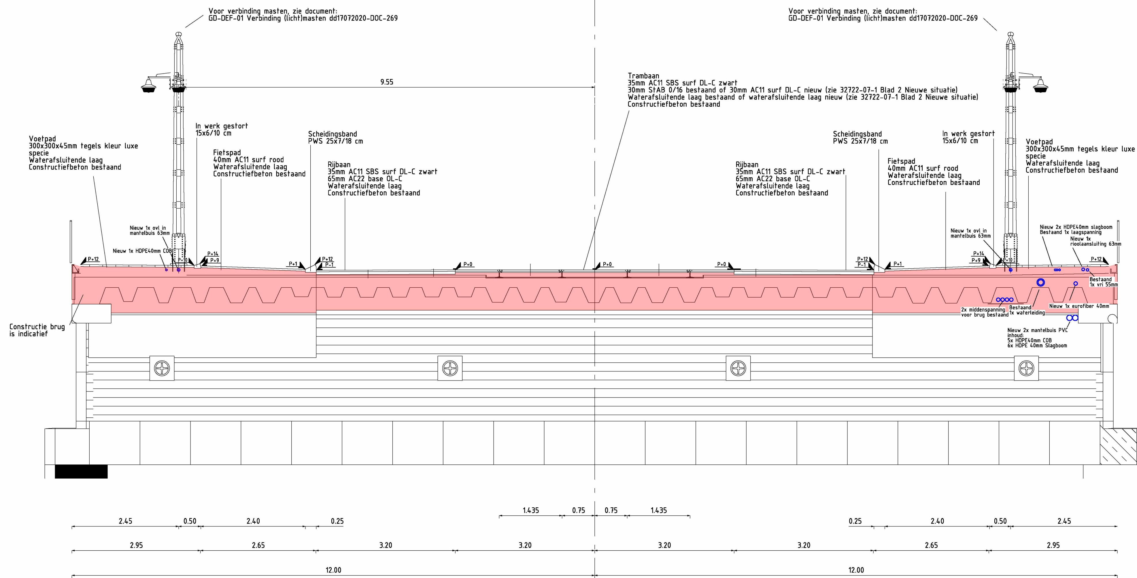
Dwarsprofiel C-C op aanbrug Nieuwe situatie schaal 1:50
