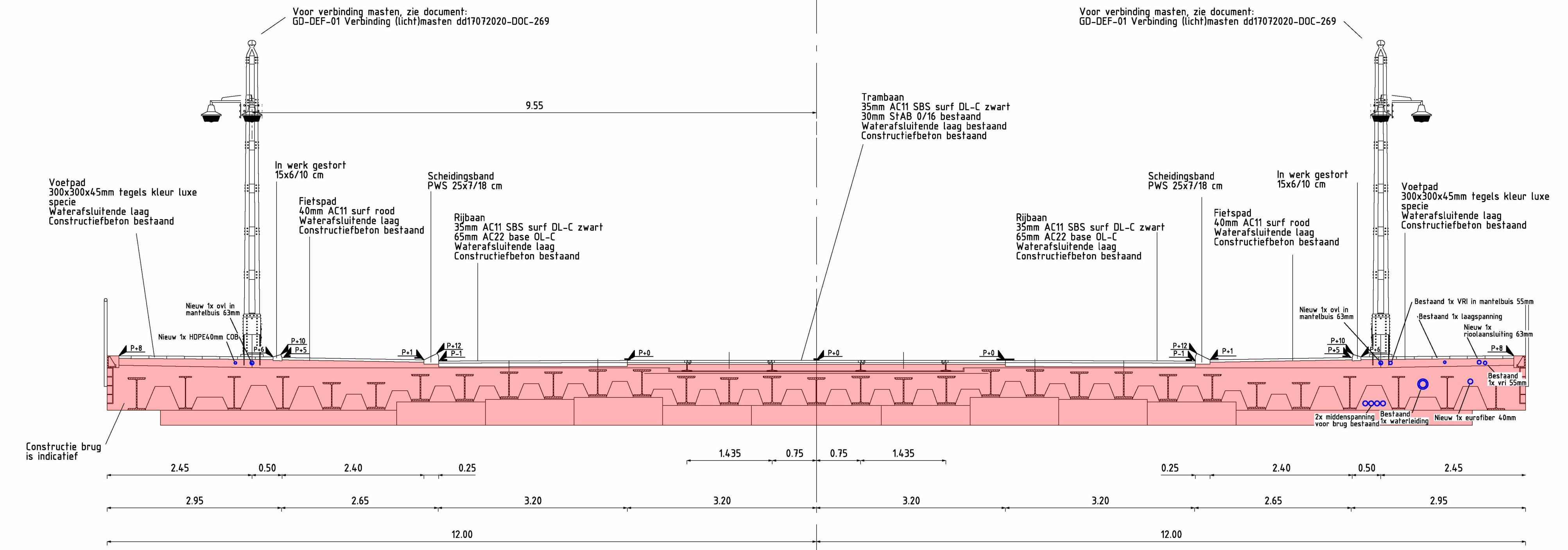
Dwarsprofiel B-B op aanbrug Nieuwe situatie schaal 1:50
