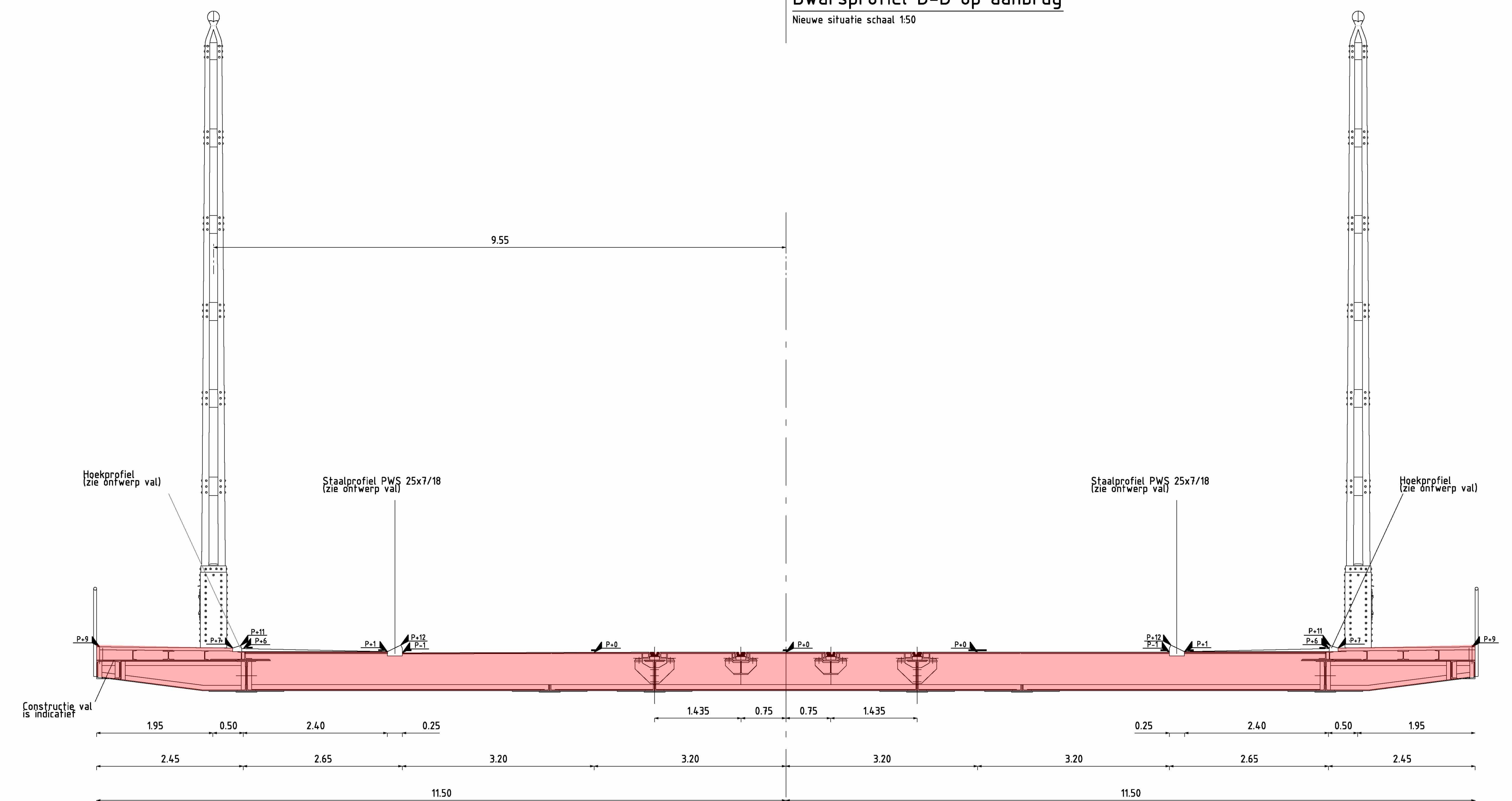
Dwarsprofiel D-D op het val Nieuwe situatie schaal 1:50
