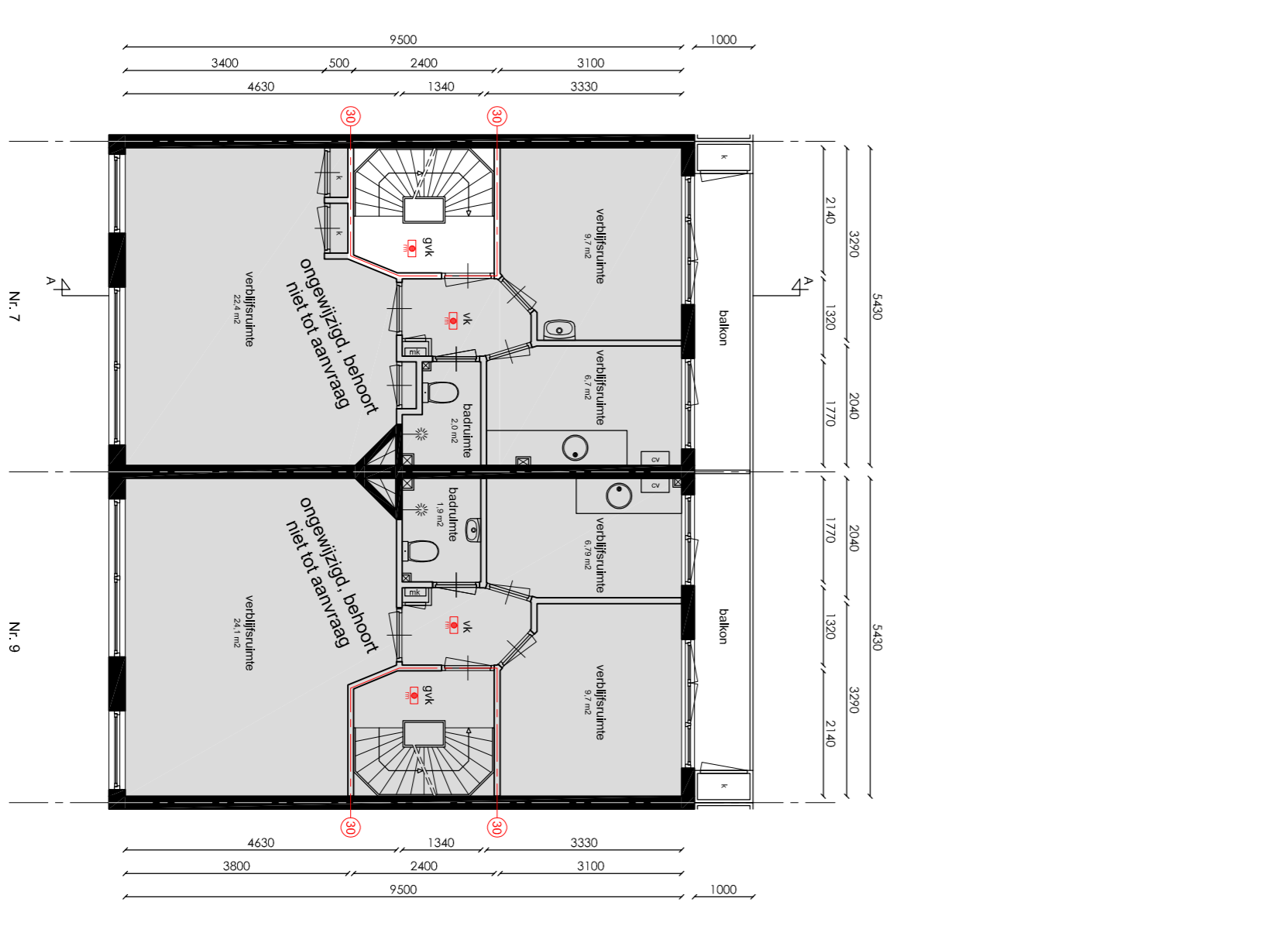
Tweede verdieping
