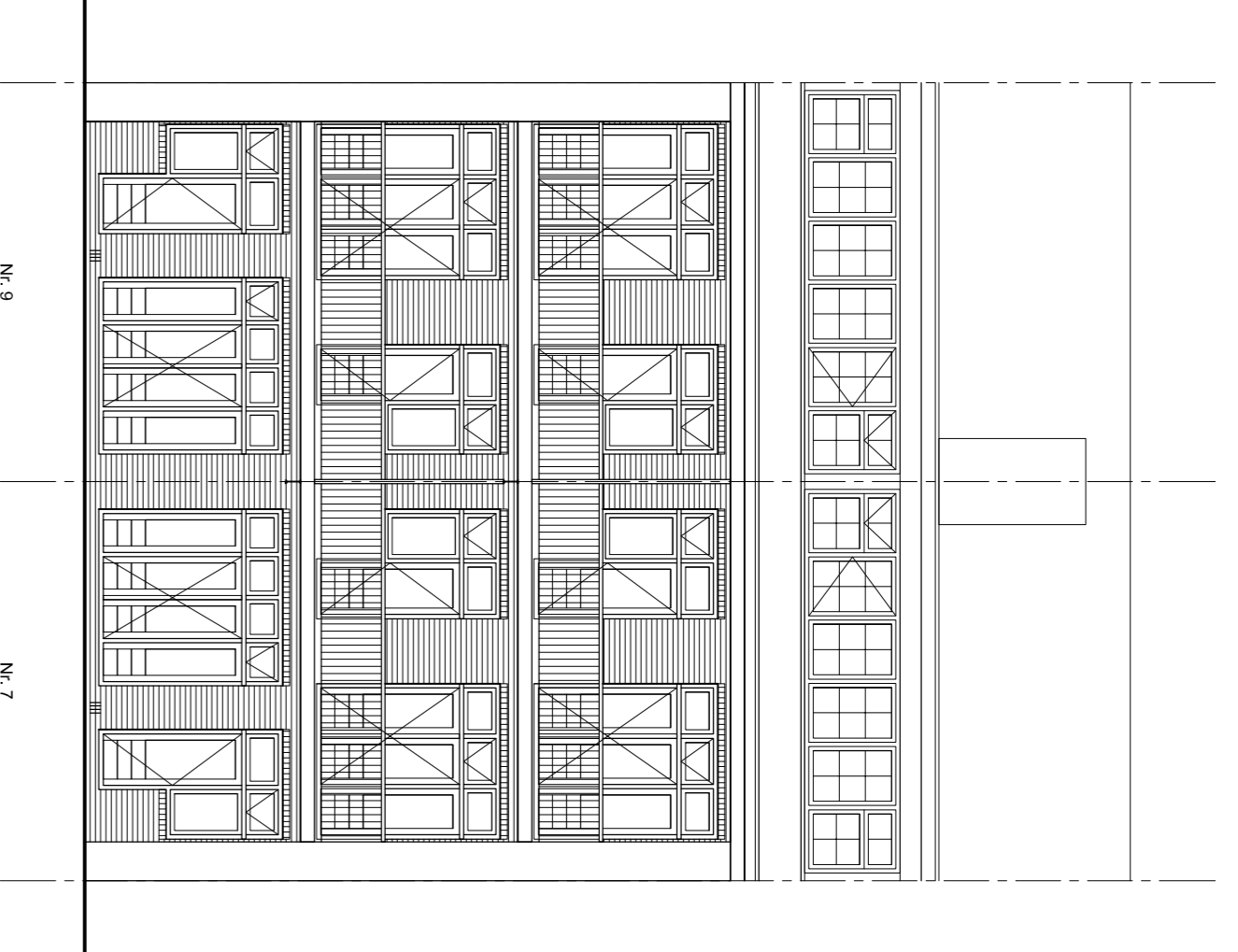
Achtergevel
