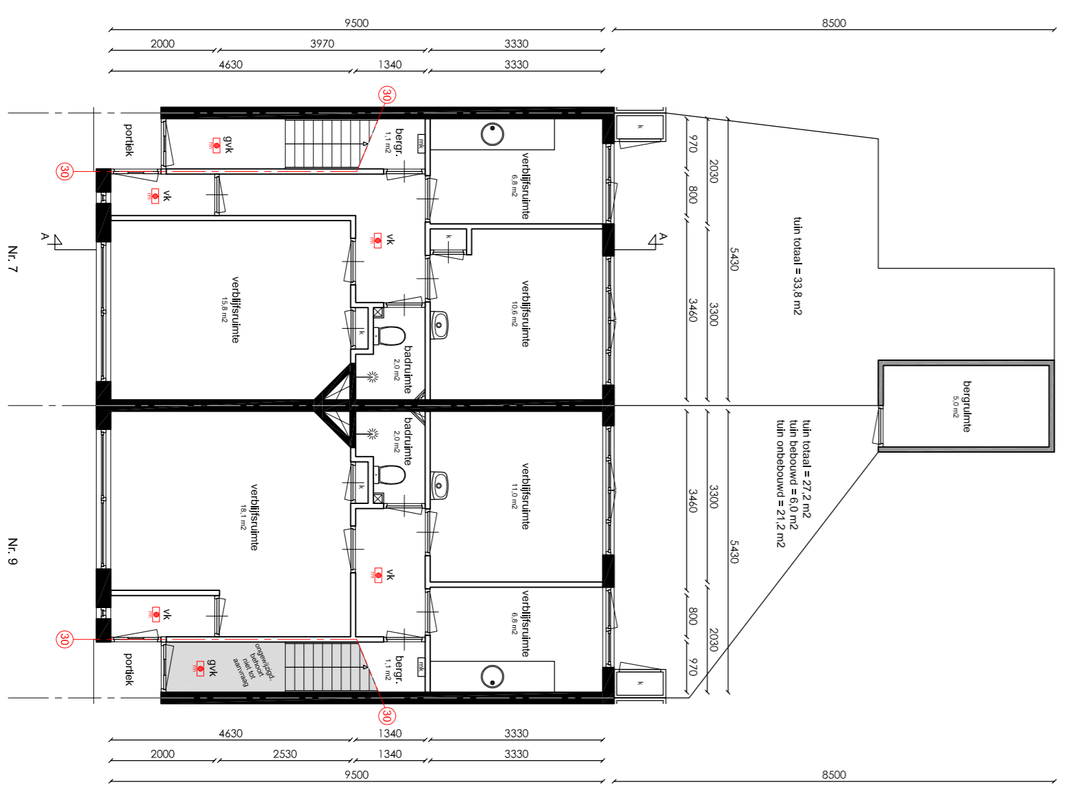
Begane grond
