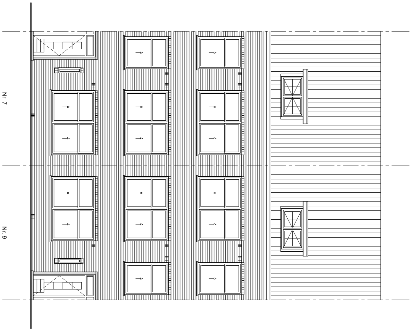
Voorgevel
