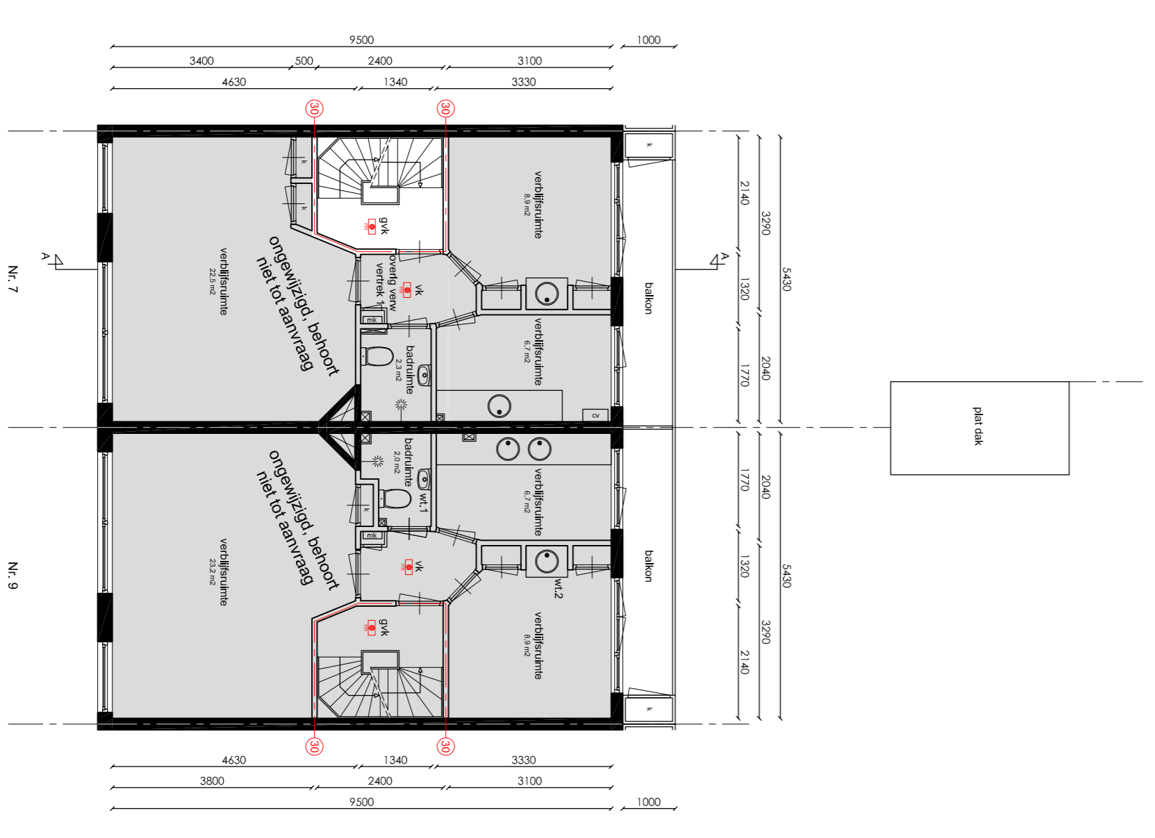
Eerste verdieping
