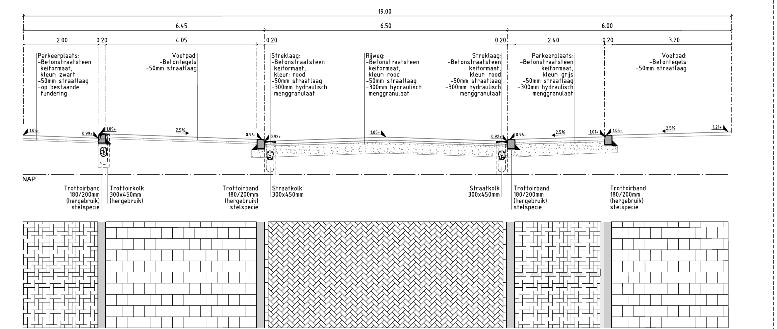
DOORSNEDE A-A SCHAAL 1 : 50
