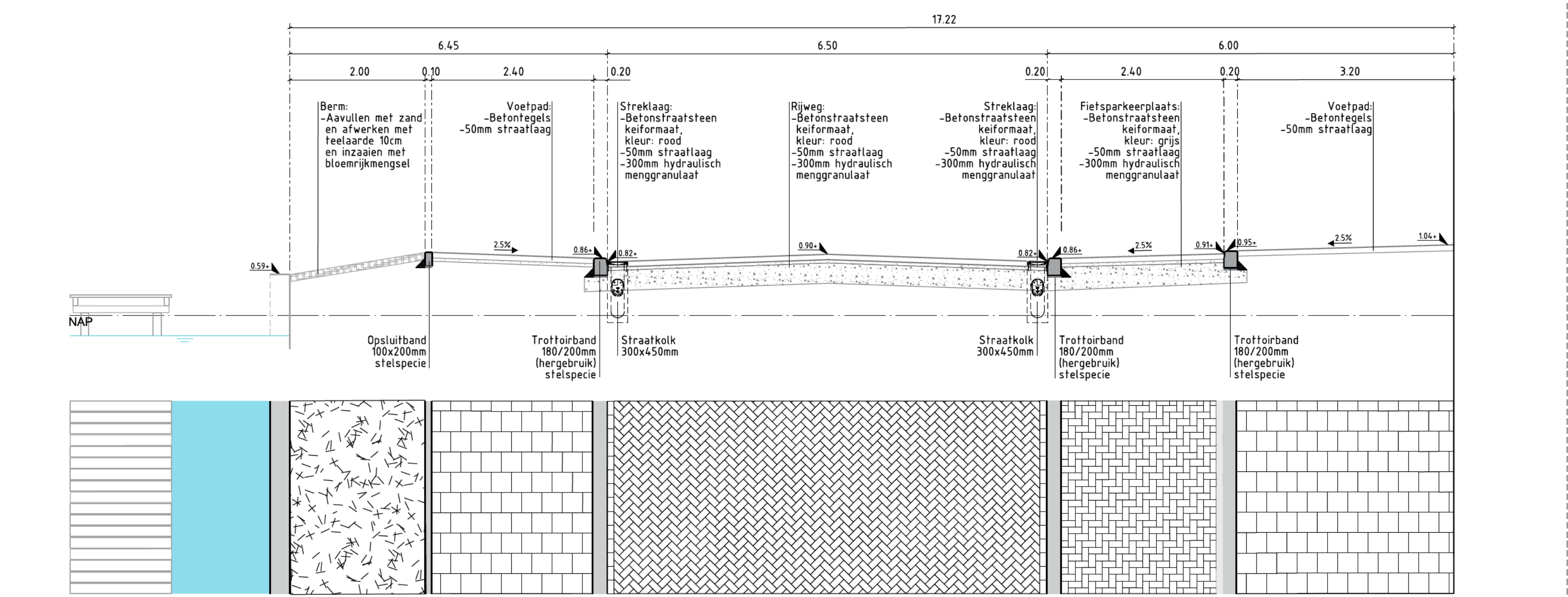
DOORSNEDE B-B SCHAAL 1 : 50
