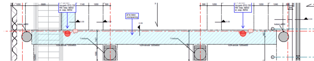
Voorgespannen balk begane grond
