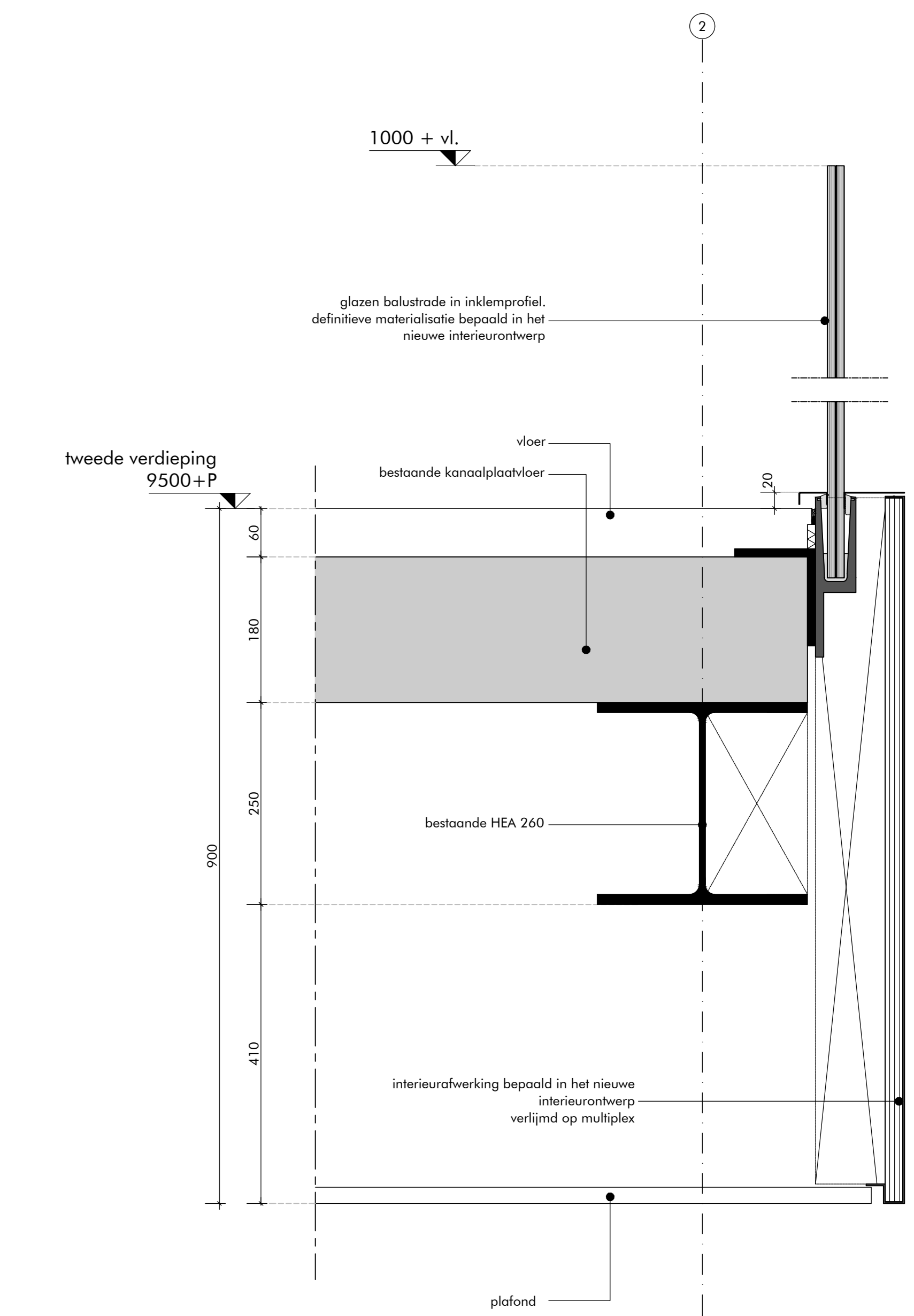
detail V-01 - vloerand 1:5
