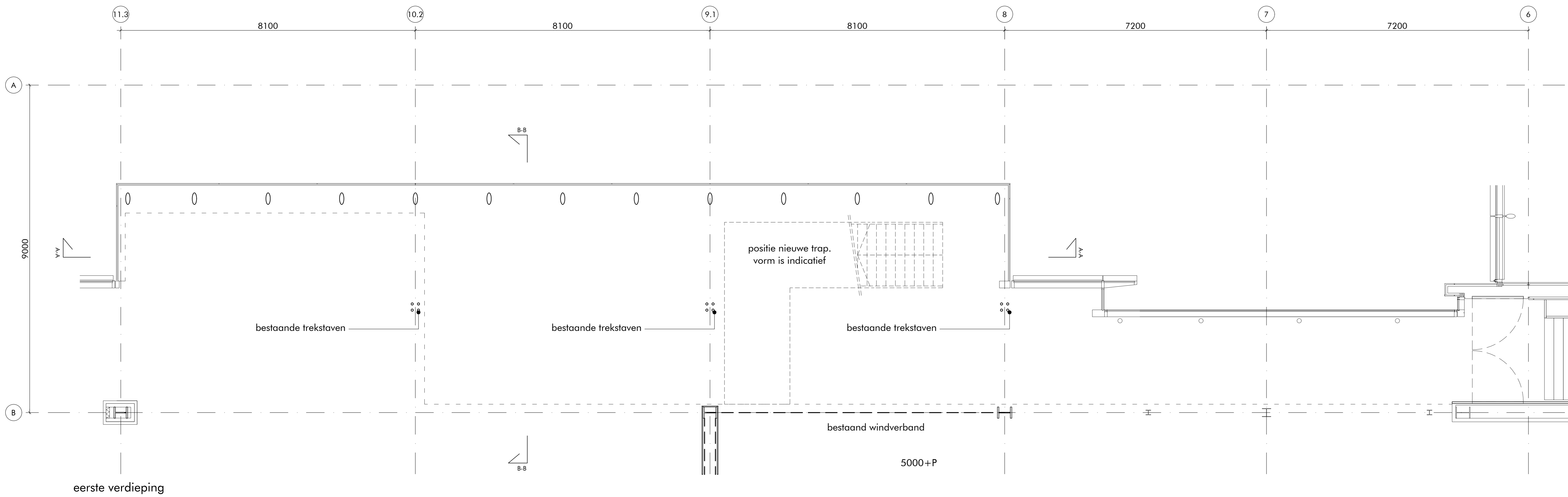
eerste verdieping
