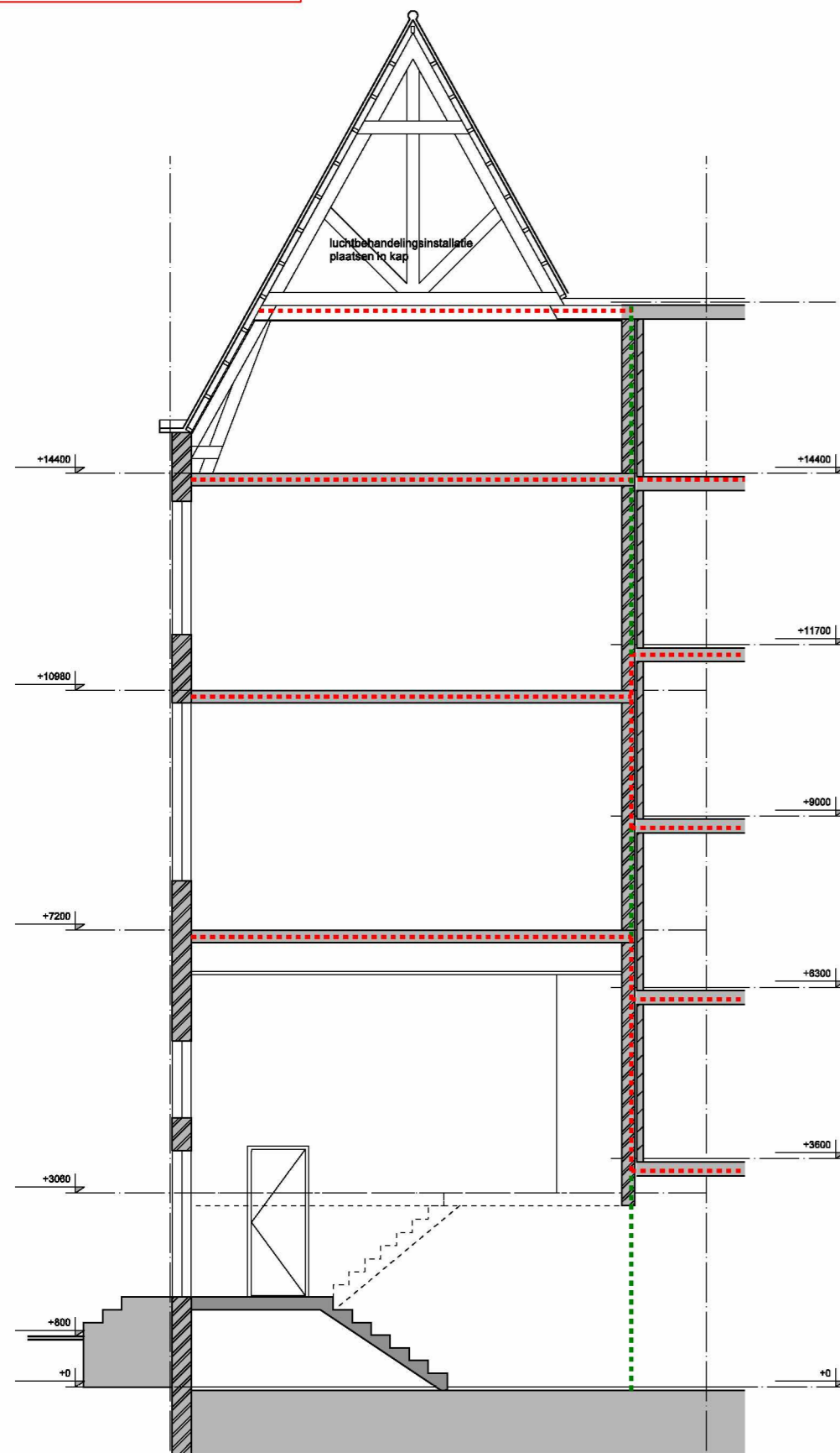
DOORSNEDE CC 1
