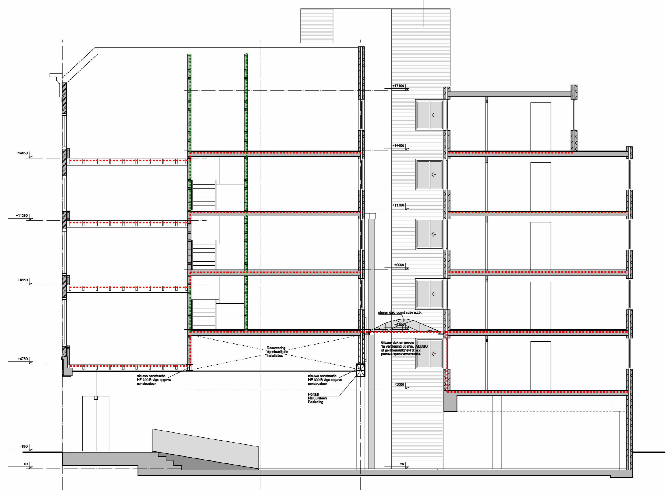
DOORSNEDE AA
