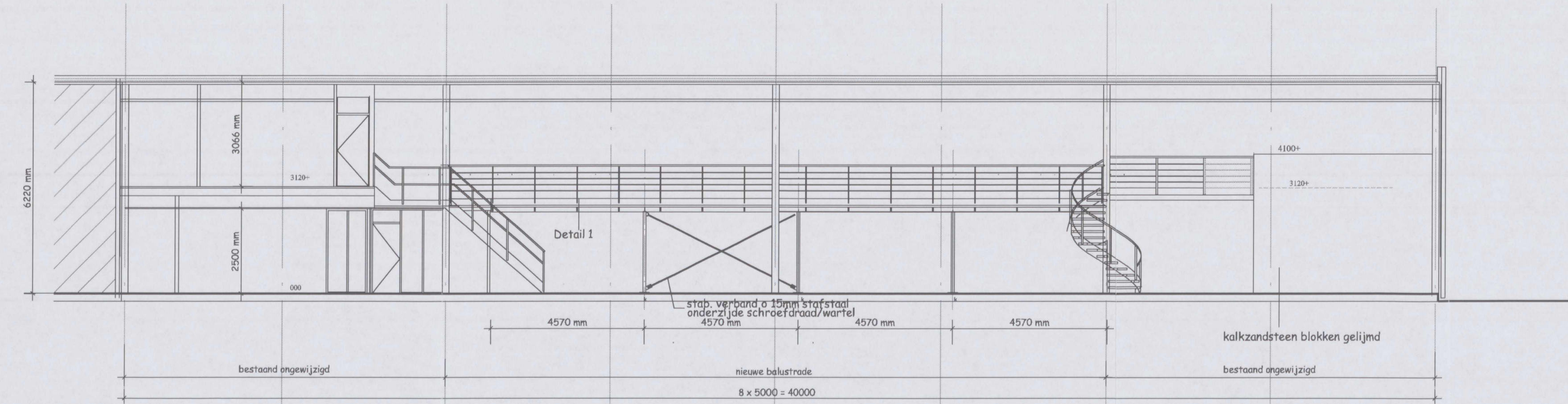
doorsnede nieuw
