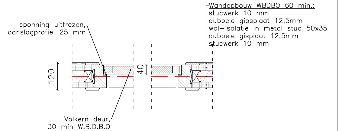
Detail P4 deur horizontaal
