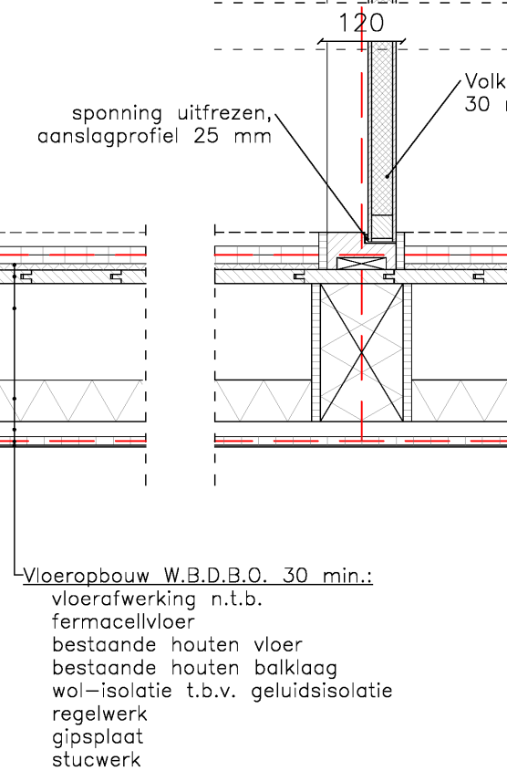
Detail P2 onderaansluiting niet dragende woningscheidende wand
