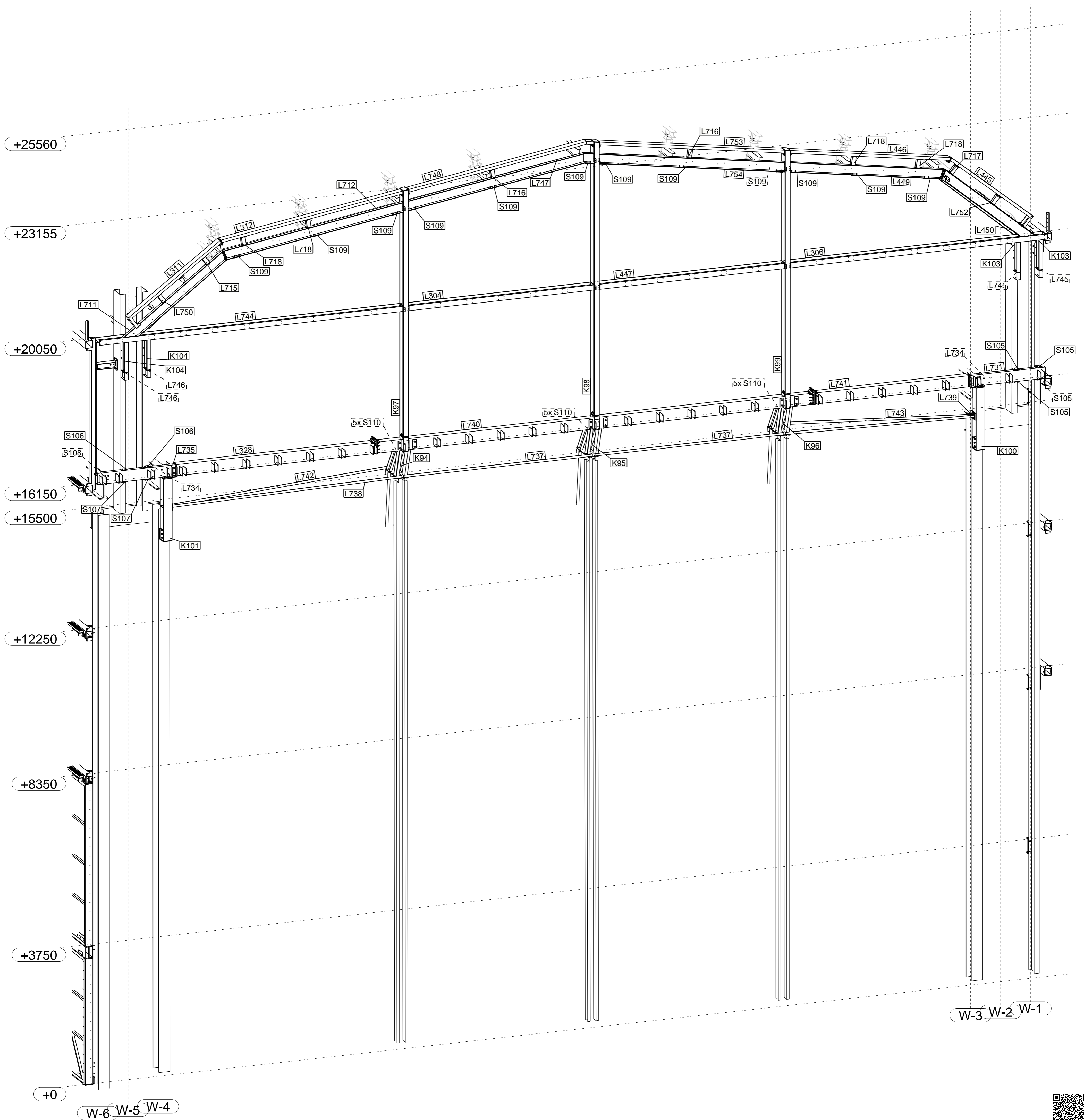
Aanzicht as W-B 1:50
