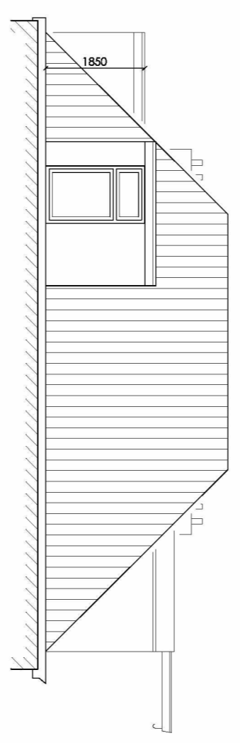
Linker zijgevel
