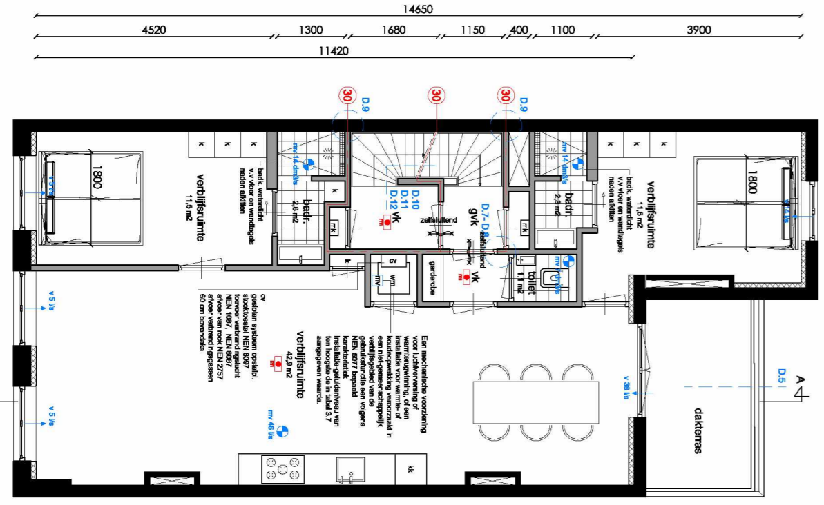
Derde verdieping
