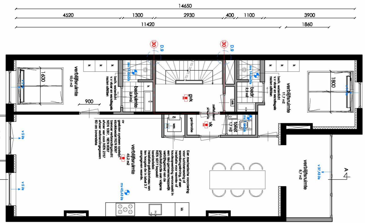
Tweede verdieping
