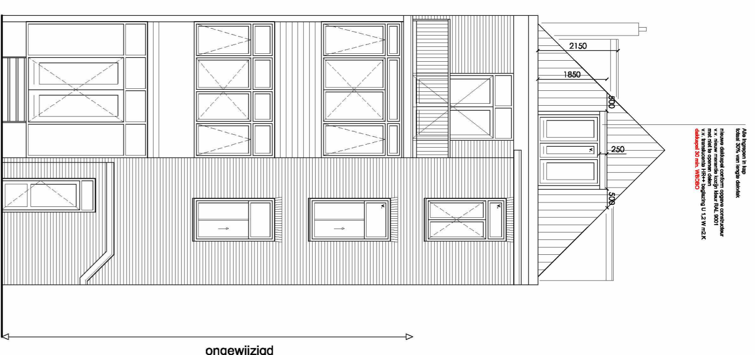
Achterevel
