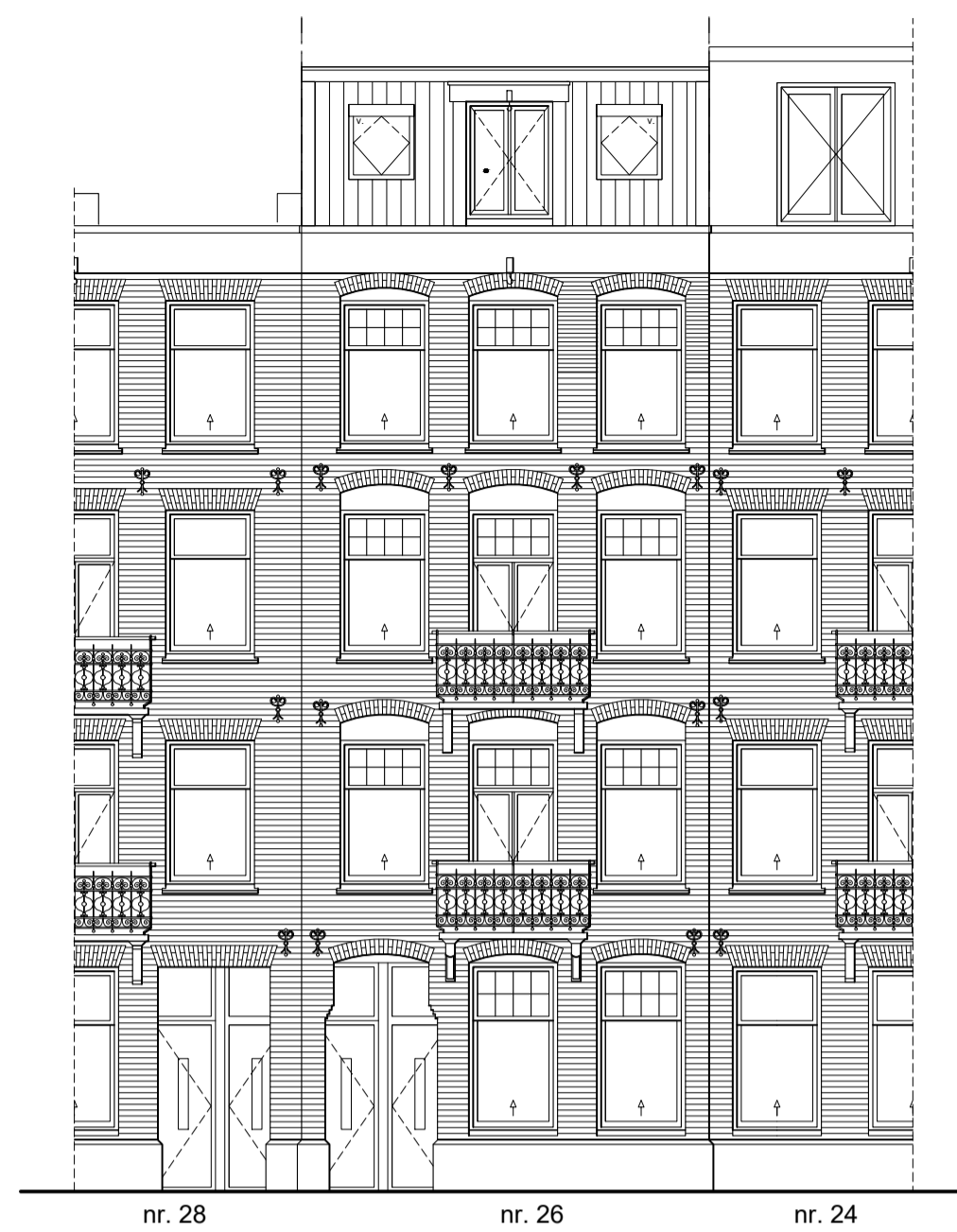
Voorgevel
