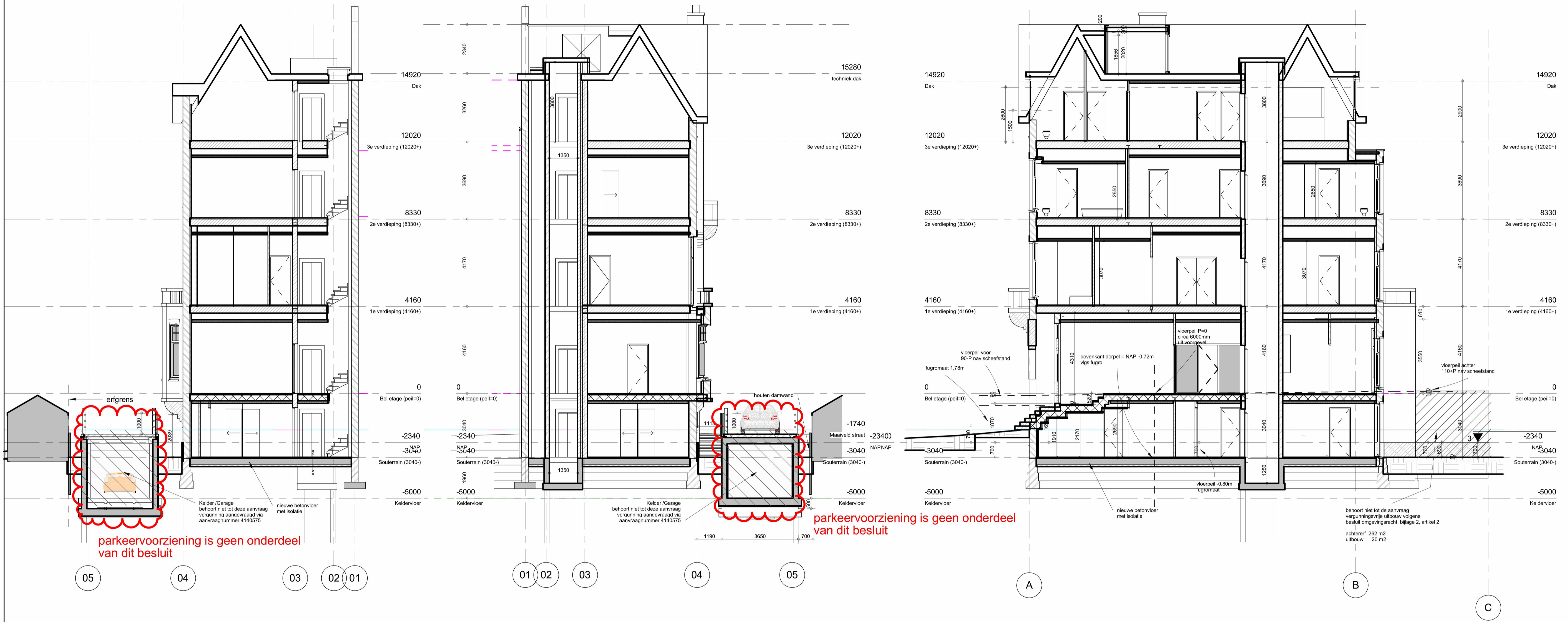
Doorsnede G-G 1 : 100
