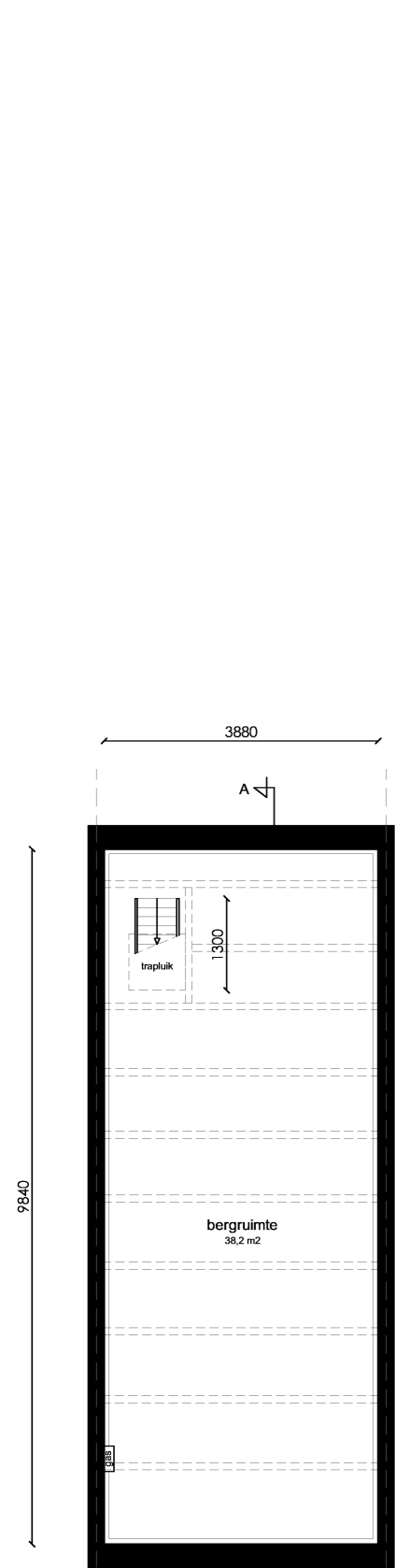
Kelder
