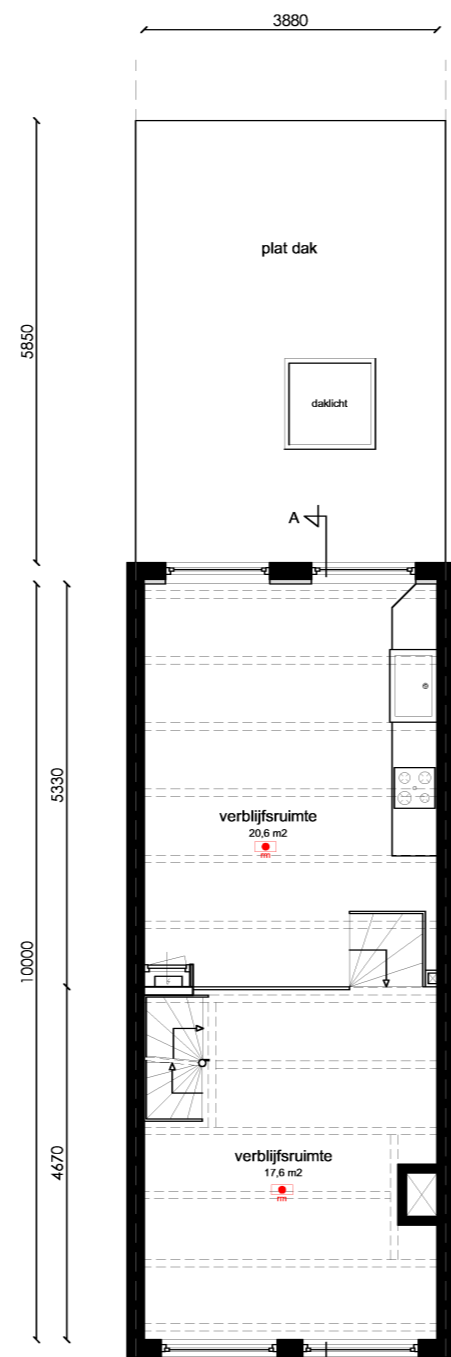
Eerste verdieping
