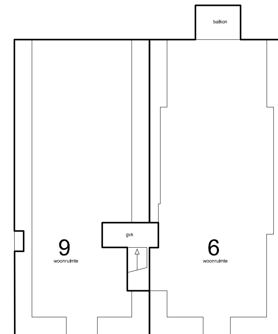
Kapverdieping schaal 1:100
