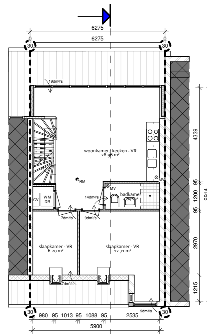
3e verdieping
