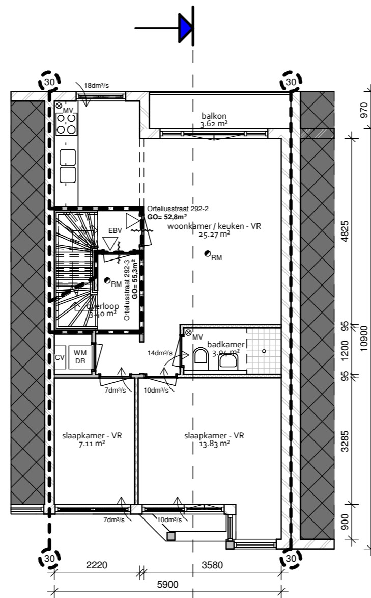
2e verdieping
