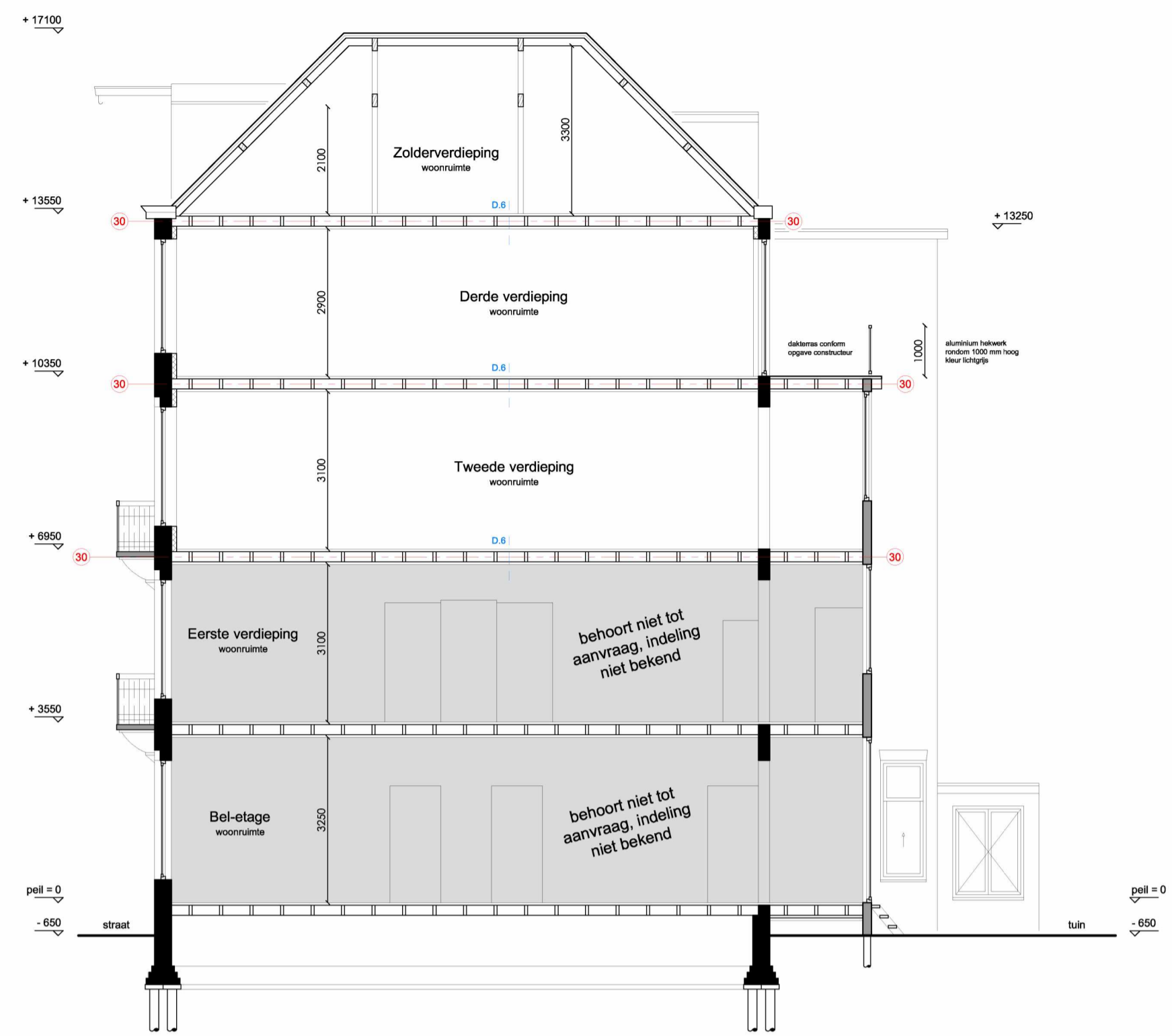
Doorsnede A-A
