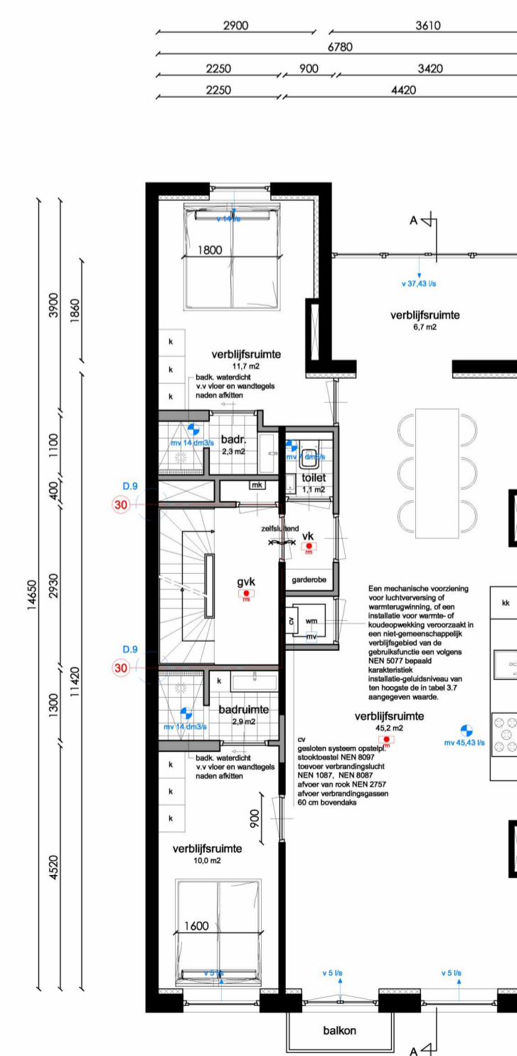
Tweede verdieping
