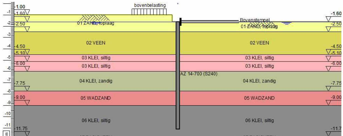
figuur 3: Bouwfase 1, ontgraving tot ca. NAP -1,6 m
