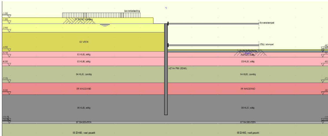
figuur 5: bouwfase 3, aanbrengen grondverbetering met een dikte van 0,30 m
