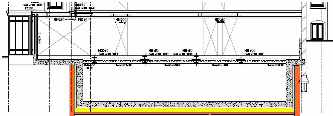
figuur 2: Doorsnede van de toekomstige keldervloer en bestaande funderingsmuren (bron: constructeur)
