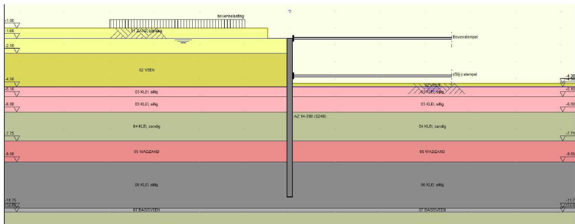
figuur 4: Bouwfase 2, maximale ontgraving tot ca. NAP -4,30 m
