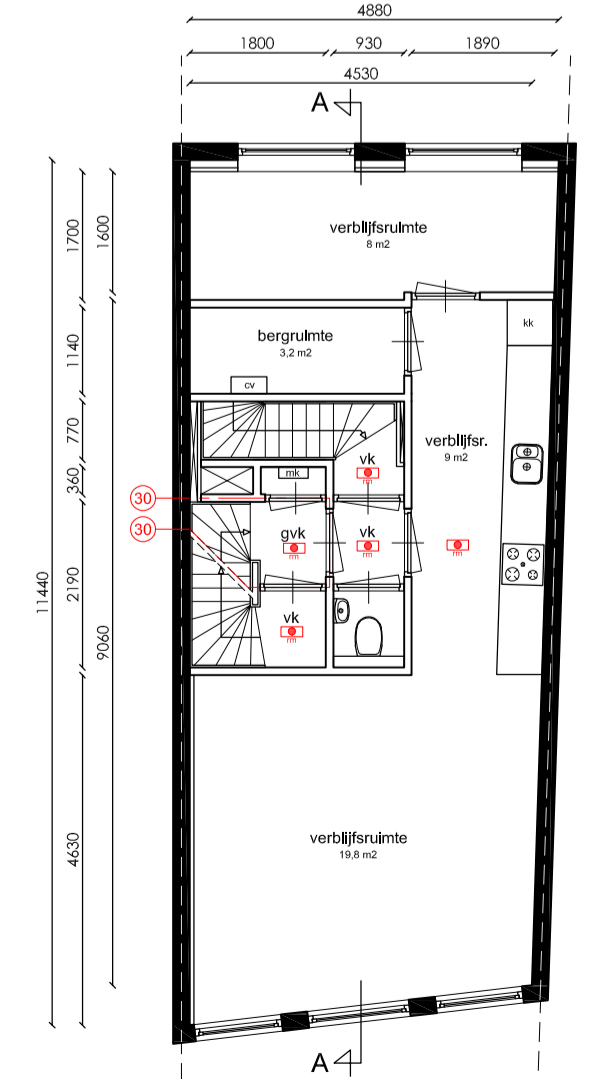
Derde verdieping
