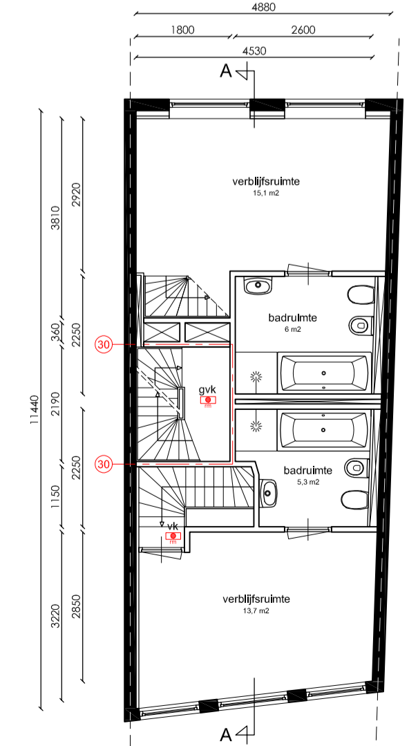
Tweede verdieping
