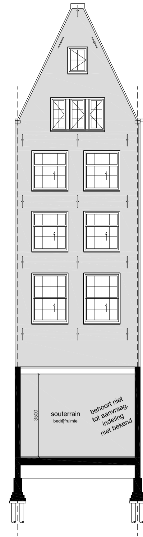
Achtergevel
