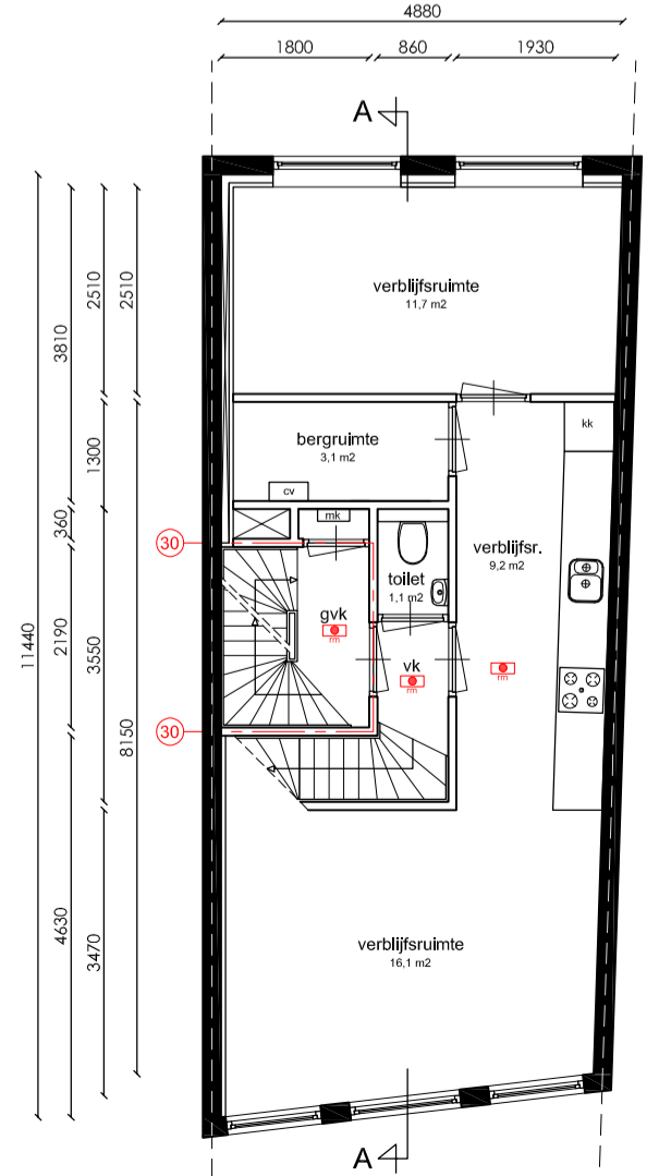
Eerste verdieping
