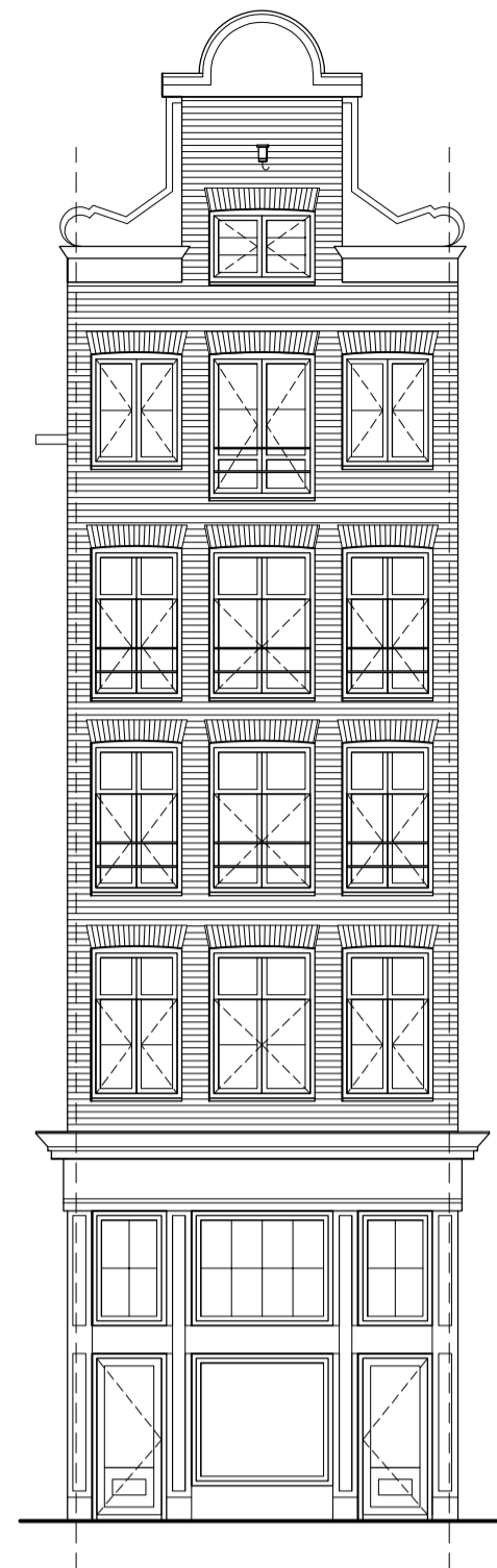
Voorgevel
