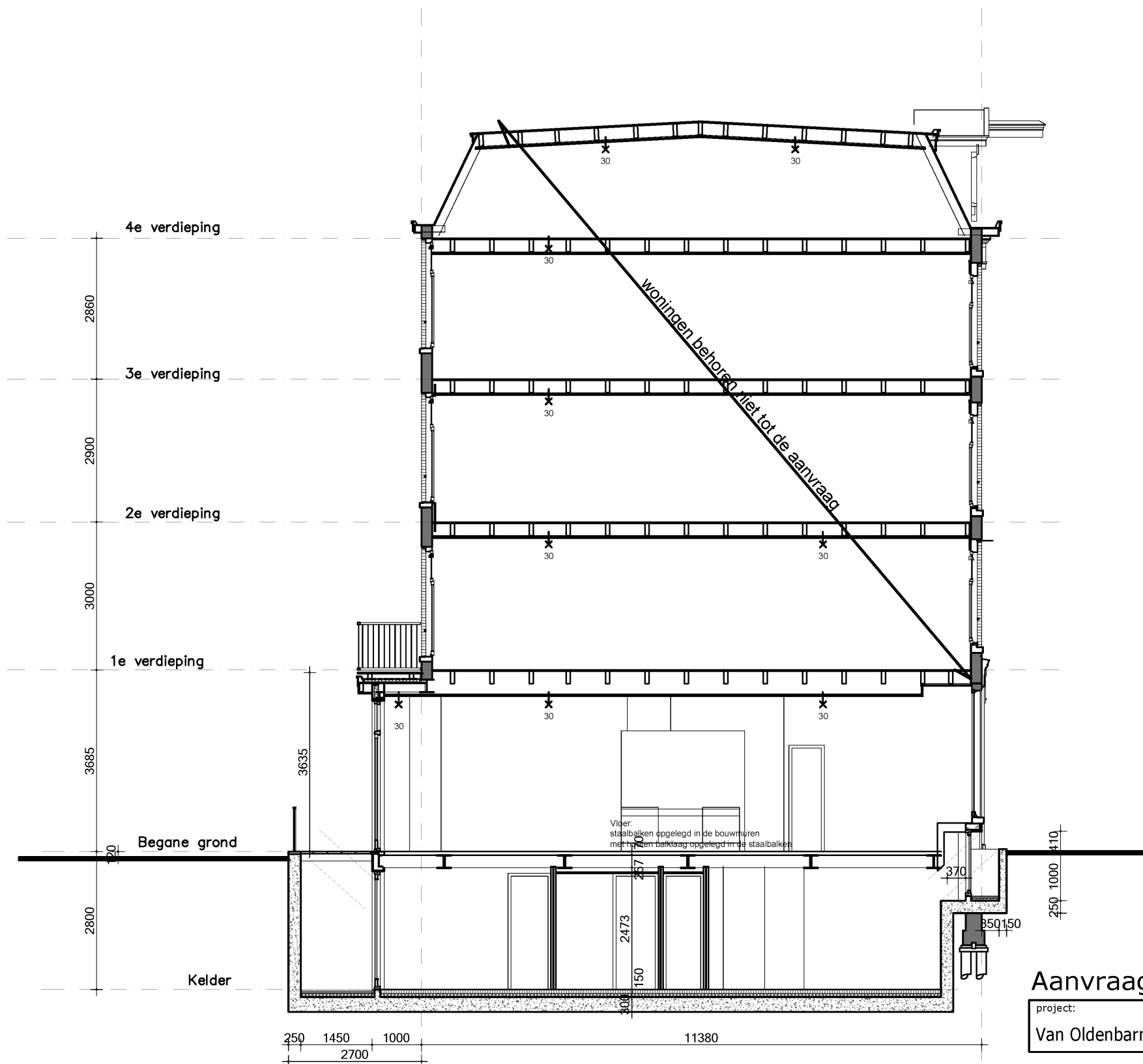
Doorsnede B-B
