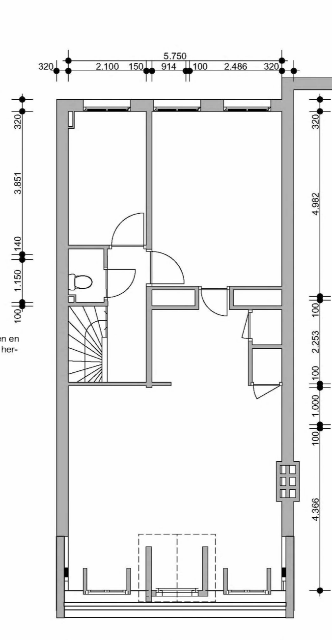
Derde verdieping
