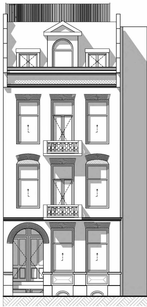
Voorgevel
