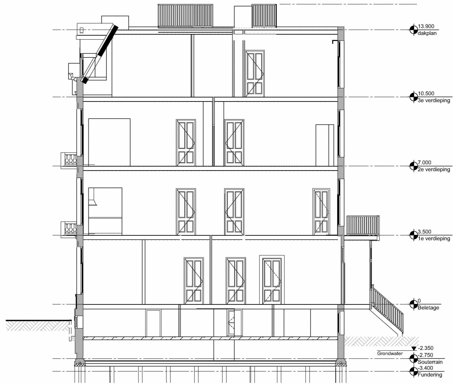
Doorsnede B - B
