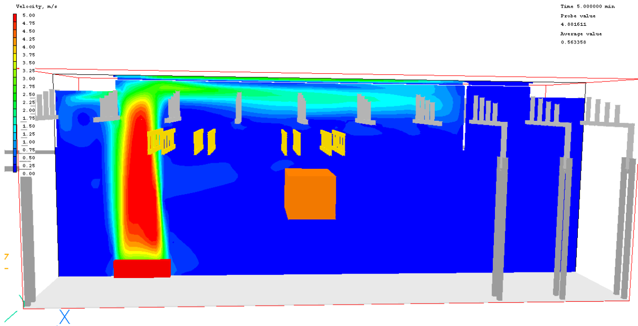
Figuur 101: Luchtsnelheden 5 minuten na aanvang brand, langsdoorsnede
