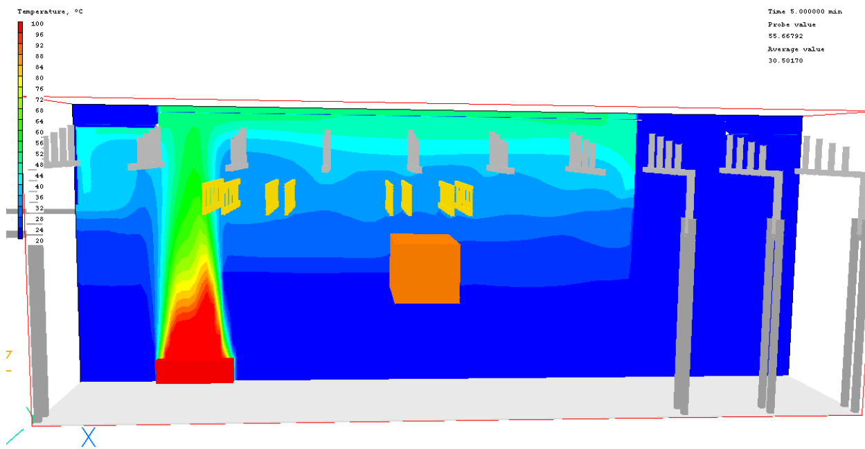
Figuur 103: Temperatuur 5 minuten na aanvang brand, langsdoorsnede
