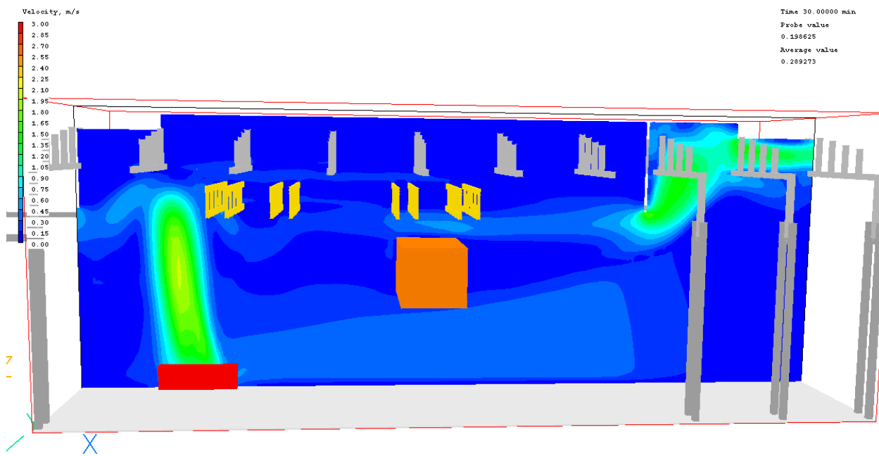
Figuur 121: Luchtsnelheden 30 minuten na aanvang brand, langsdoorsnede
