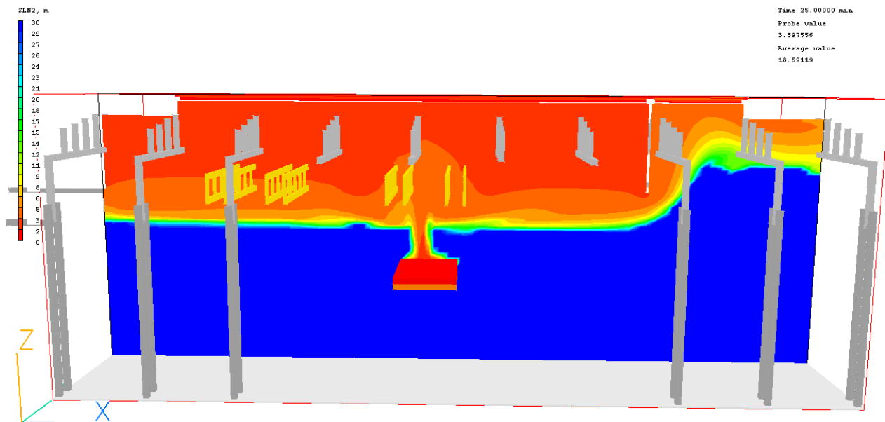
Figuur 218: Zichtlengte 25 minuten na aanvang brand, langsdoorsnede
