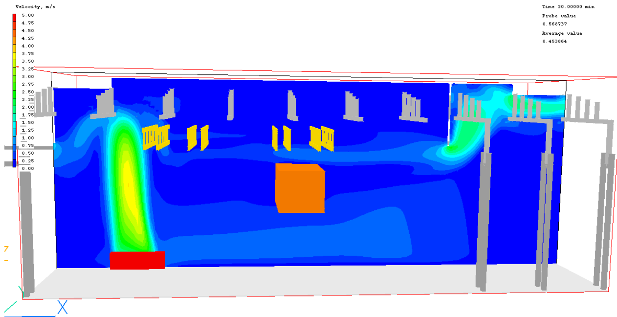
Figuur 113: Luchtsnelheden 20 minuten na aanvang brand, langsdoorsnede
