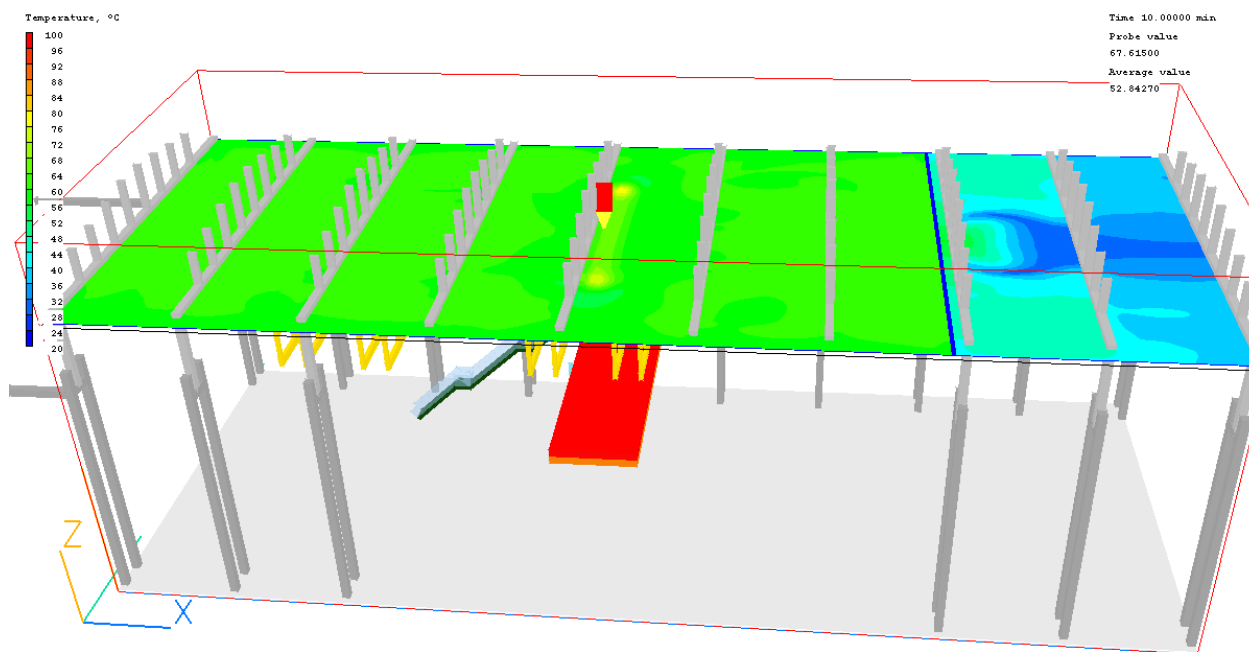
Figuur 208: Temperatuur 10 minuten na aanvang brand, doorsnede over draagbalken
