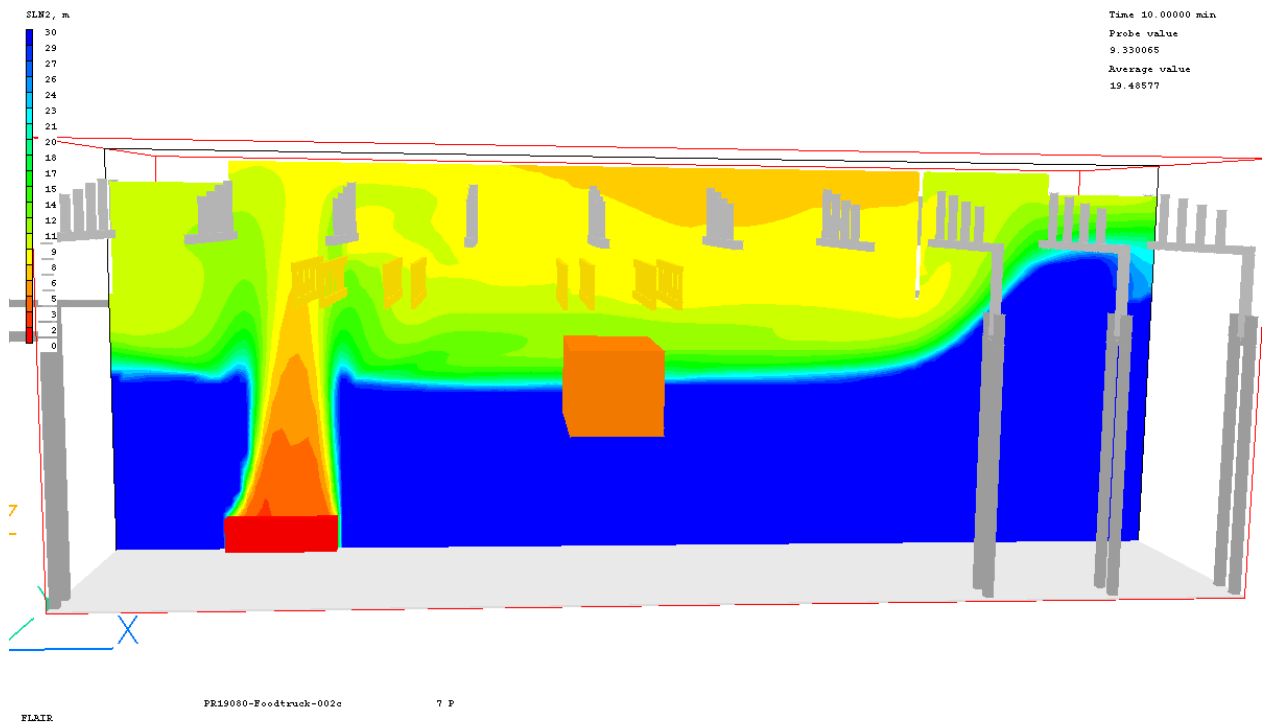
Figuur 106: Zichtlengte 10 minuten na aanvang brand, langsdoorsnede
