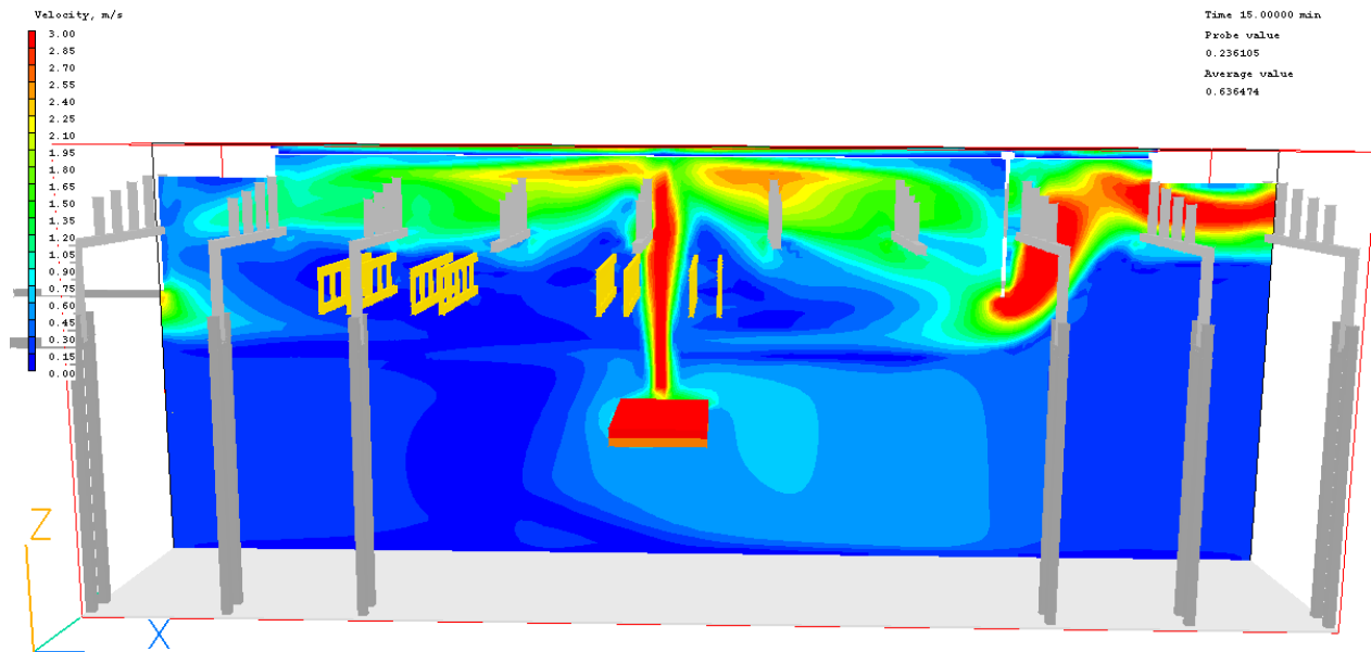
Figuur 209: Luchtsnelheden 15 minuten na aanvang brand, langsdoorsnede
