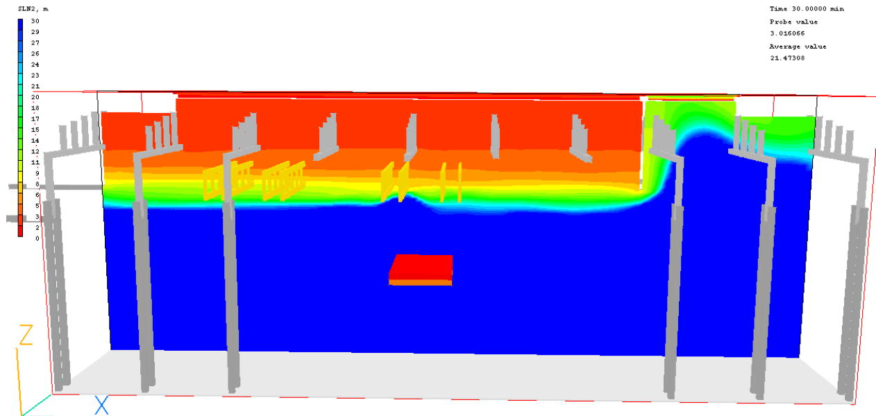
Figuur 222: Zichtlengte 30 minuten na aanvang brand, langsdoorsnede
