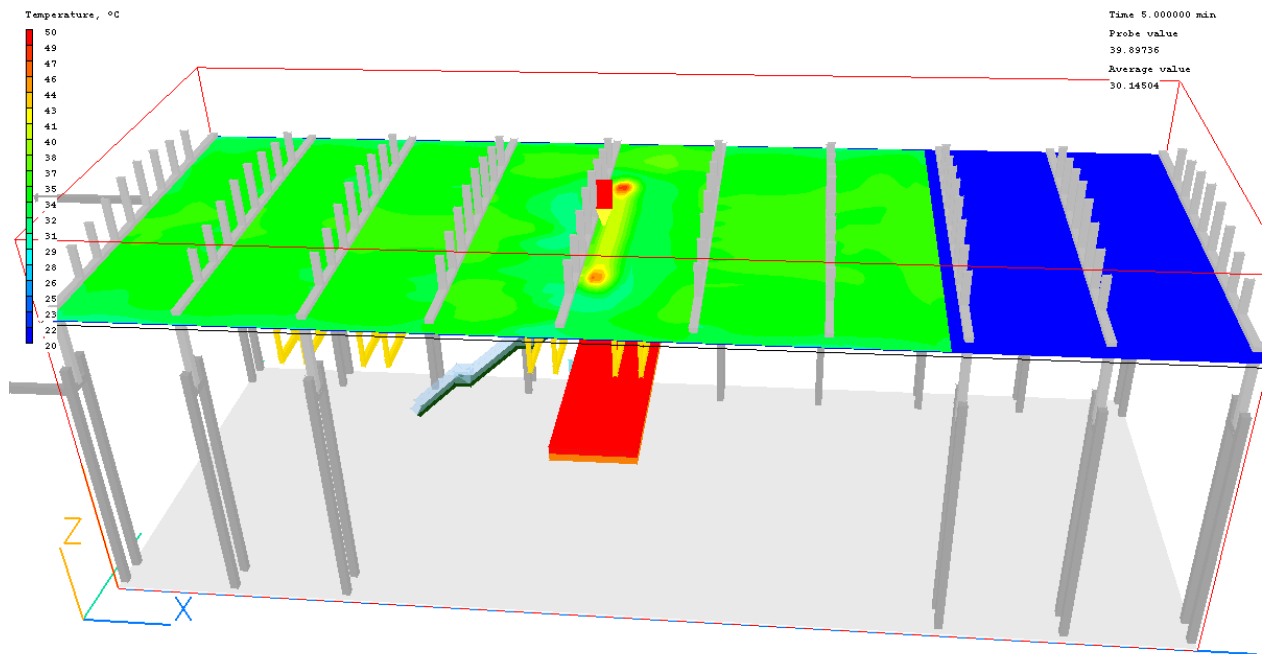
Figuur 204: Temperatuur 5 minuten na aanvang brand, doorsnede over draagbalken
