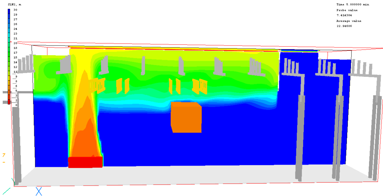
Figuur 102: Zichtlengte 5 minuten na aanvang brand, langsdoorsnede
