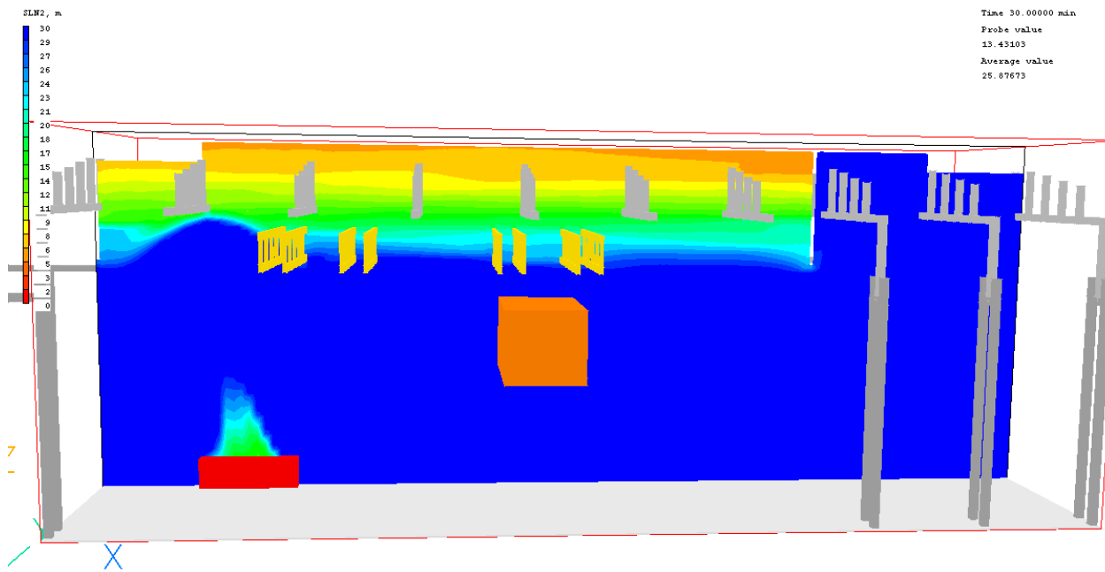
Figuur 122: Zichtlengte 30 minuten na aanvang brand, langsdoorsnede
