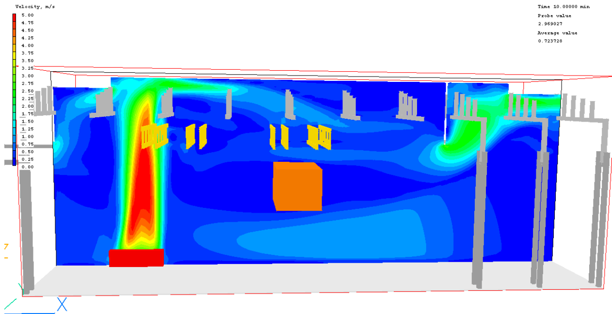
Figuur 105: Luchtsnelheden 10 minuten na aanvang brand, langsdoorsnede
