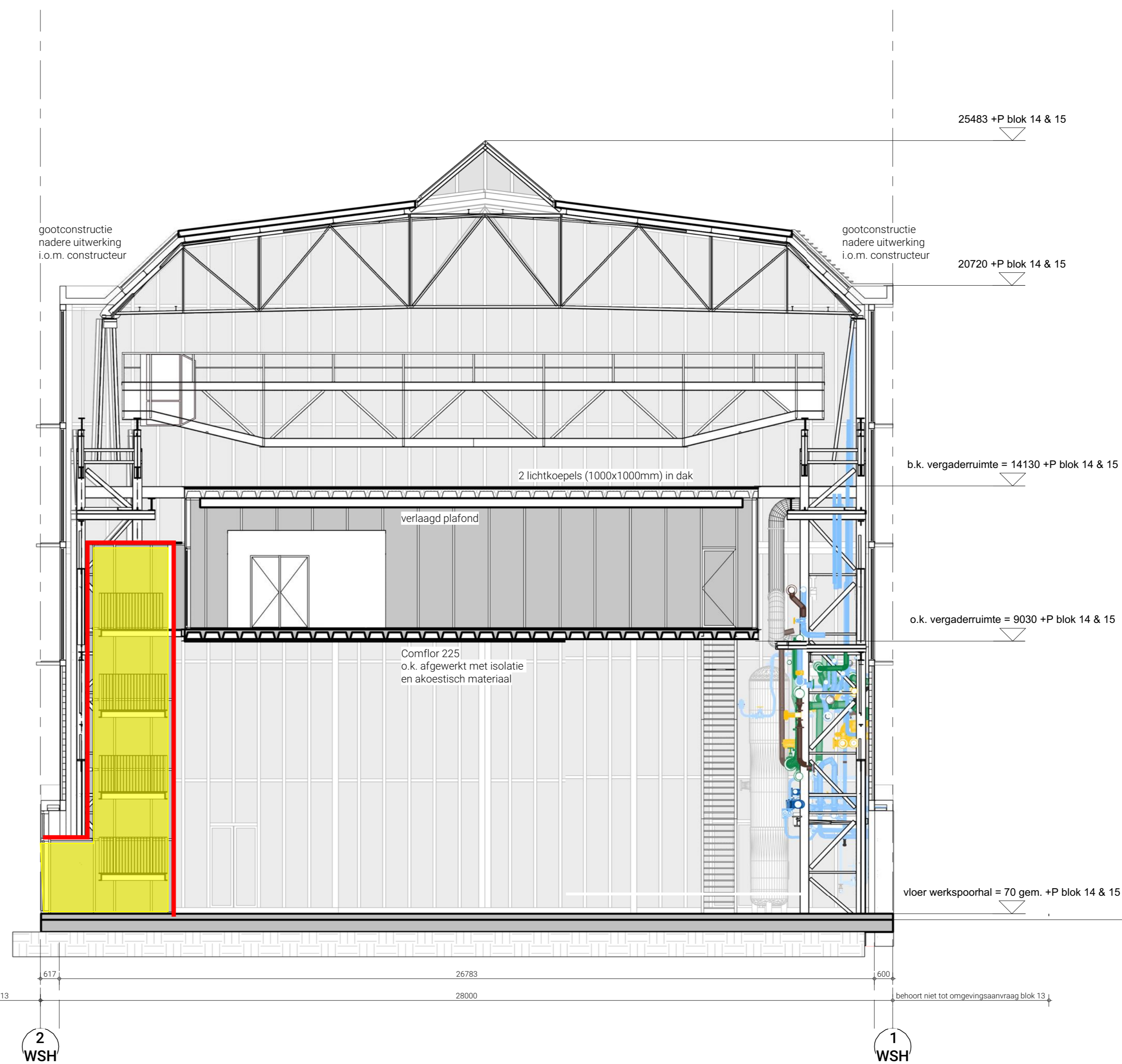
Drasn D1-D1 1:100
