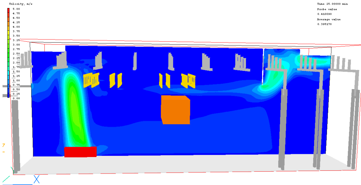
Figuur 117: Luchtsnelheden 25 minuten na aanvang brand, langsdoorsnede
