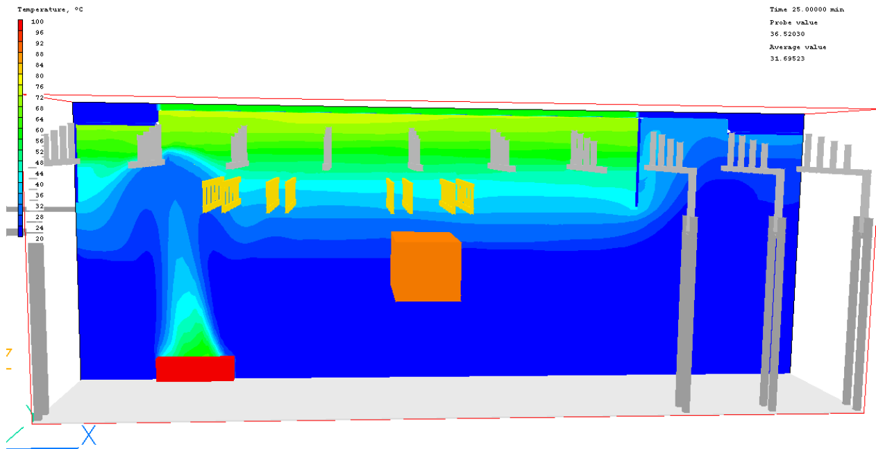
Figuur 119: Temperatuur 25 minuten na aanvang brand, langsdoorsnede
