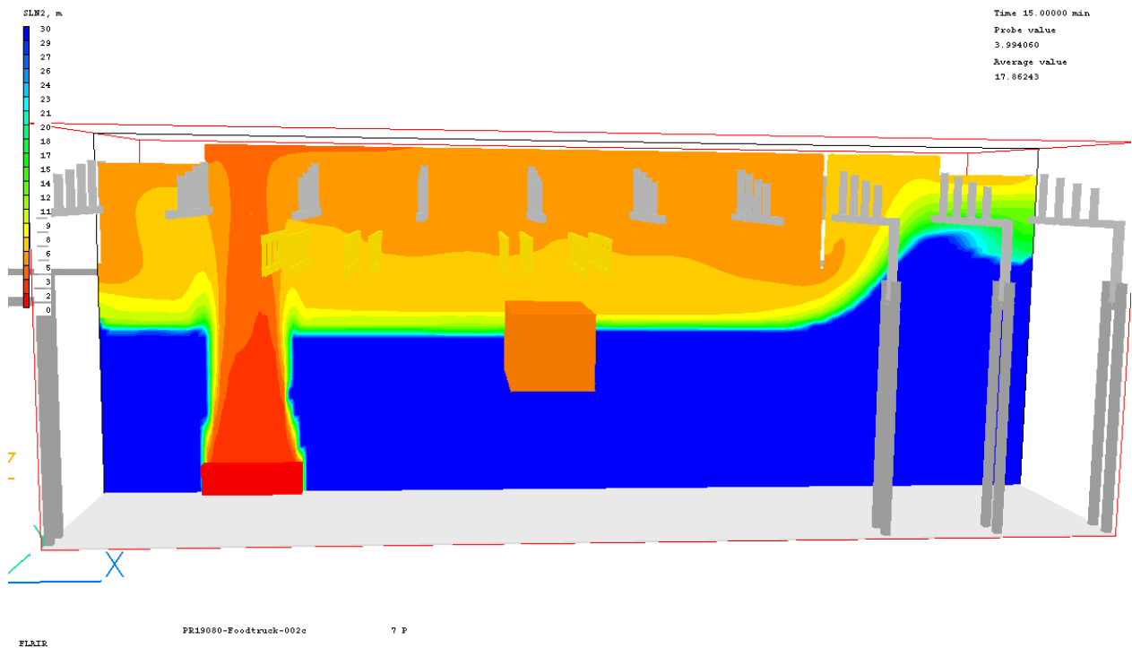
Figuur 110: Zichtlengte 15 minuten na aanvang brand, langsdoorsnede
