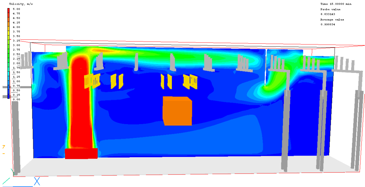
Figuur 109: Luchtsnelheden 15 minuten na aanvang brand, langsdoorsnede
