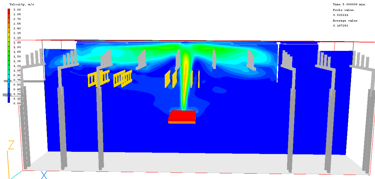
Figuur 201: Luchtsnelheden 5 minuten na aanvang brand, langsdoorsnede
