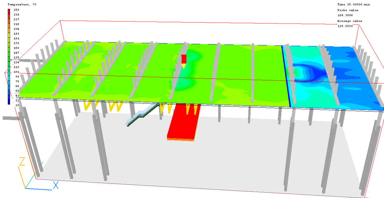
Figuur 220: Temperatuur 25 minuten na aanvang brand, doorsnede over draagbalken
