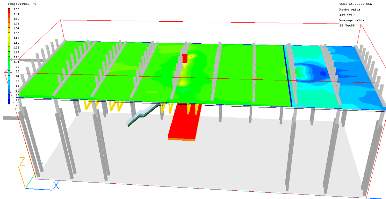
Figuur 212: Temperatuur 15 minuten na aanvang brand, doorsnede over draagbalken
