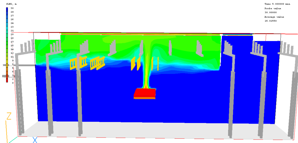
Figuur 202: Zichtlengte 5 minuten na aanvang brand, langsdoorsnede
