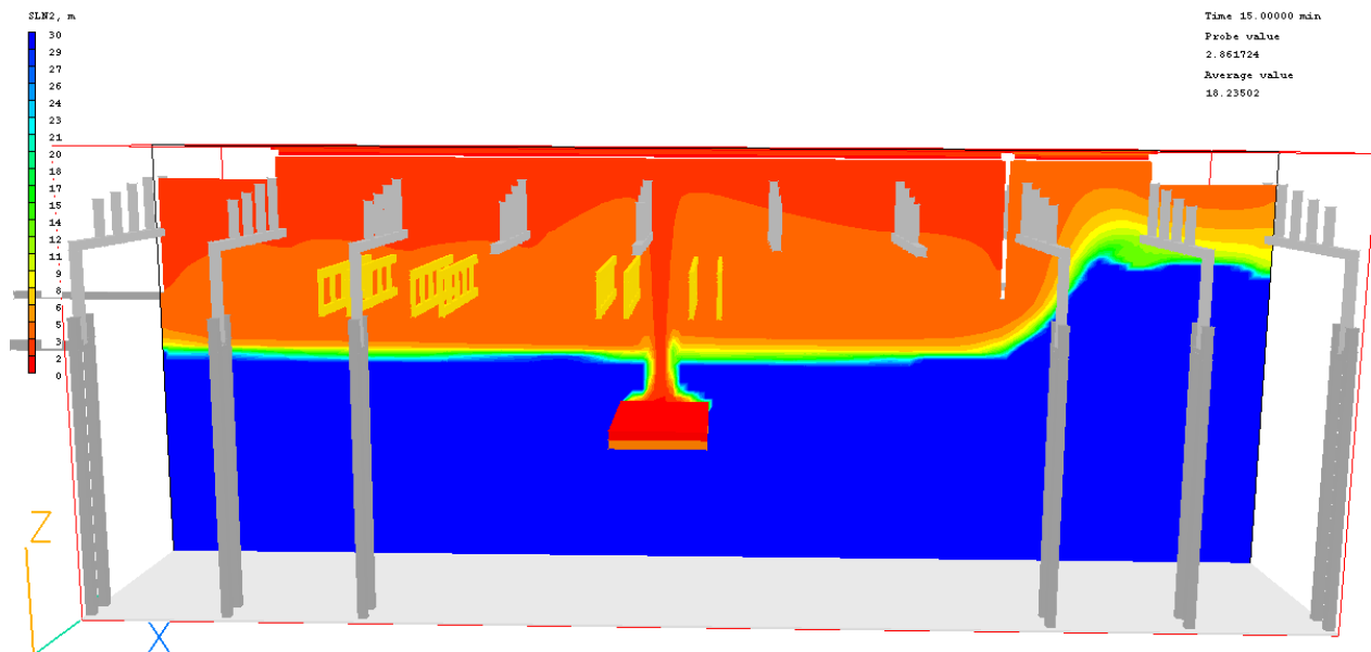
Figuur 210: Zichtlengte 15 minuten na aanvang brand, langsdoorsnede
