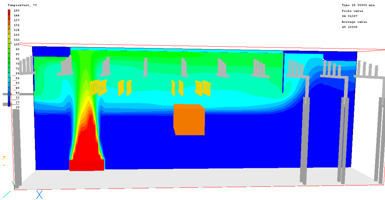
Figuur 111: Temperatuur 15 minuten na aanvang brand, langsdoorsnede
