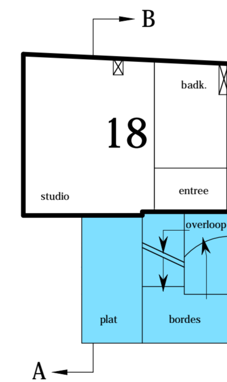
TUSSENVERDIEPING 1 : 100
