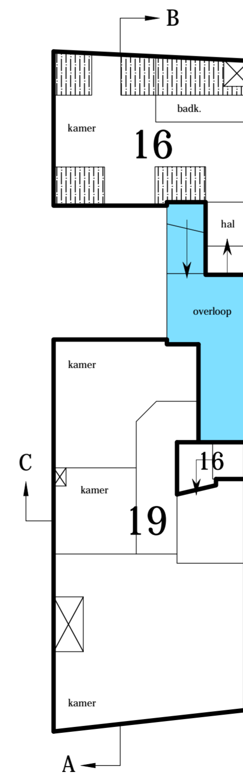
2e VERDIEPING ~ 1 : 100
