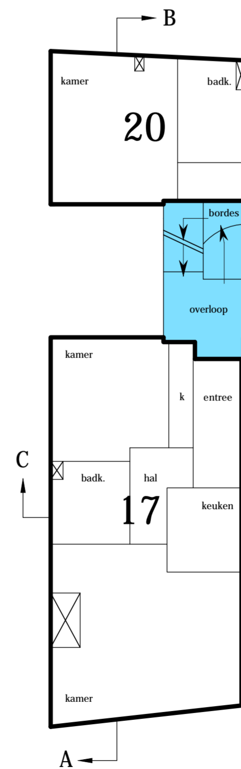
1e VERDIEPING ~ 1 : 100
