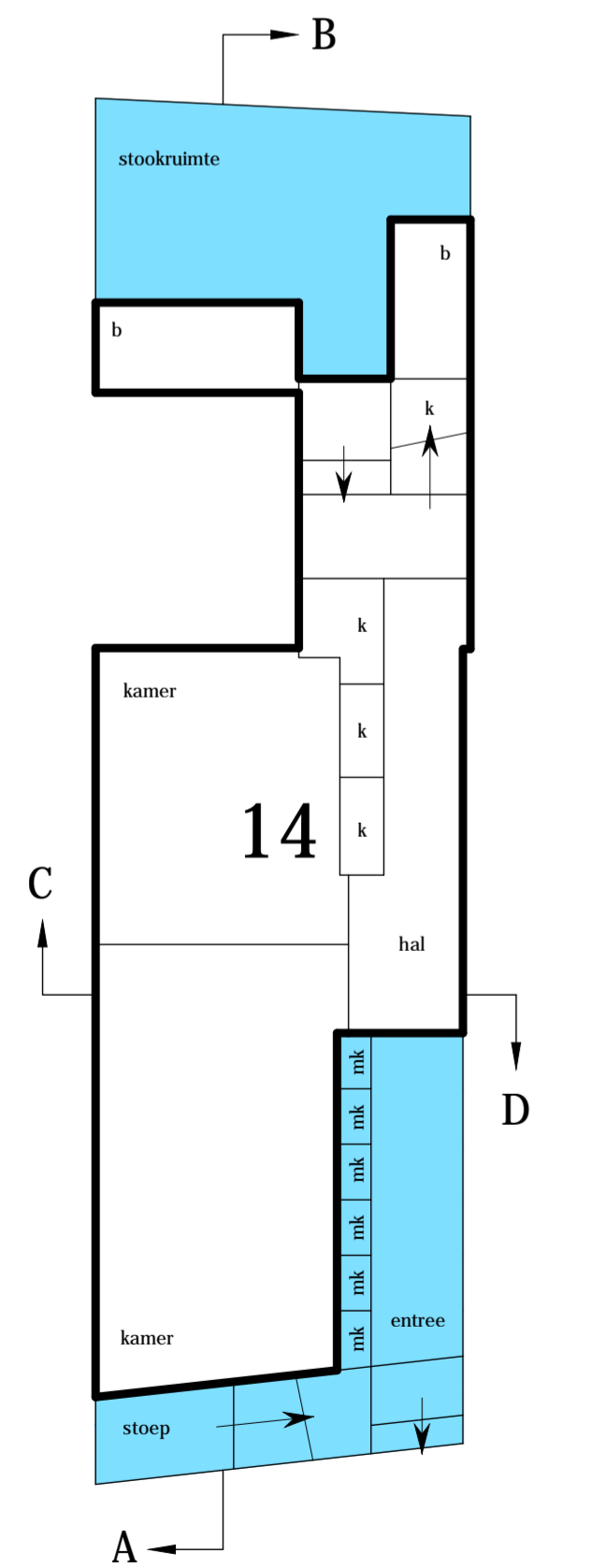
SOUTERRAIN ~ 1 : 100
