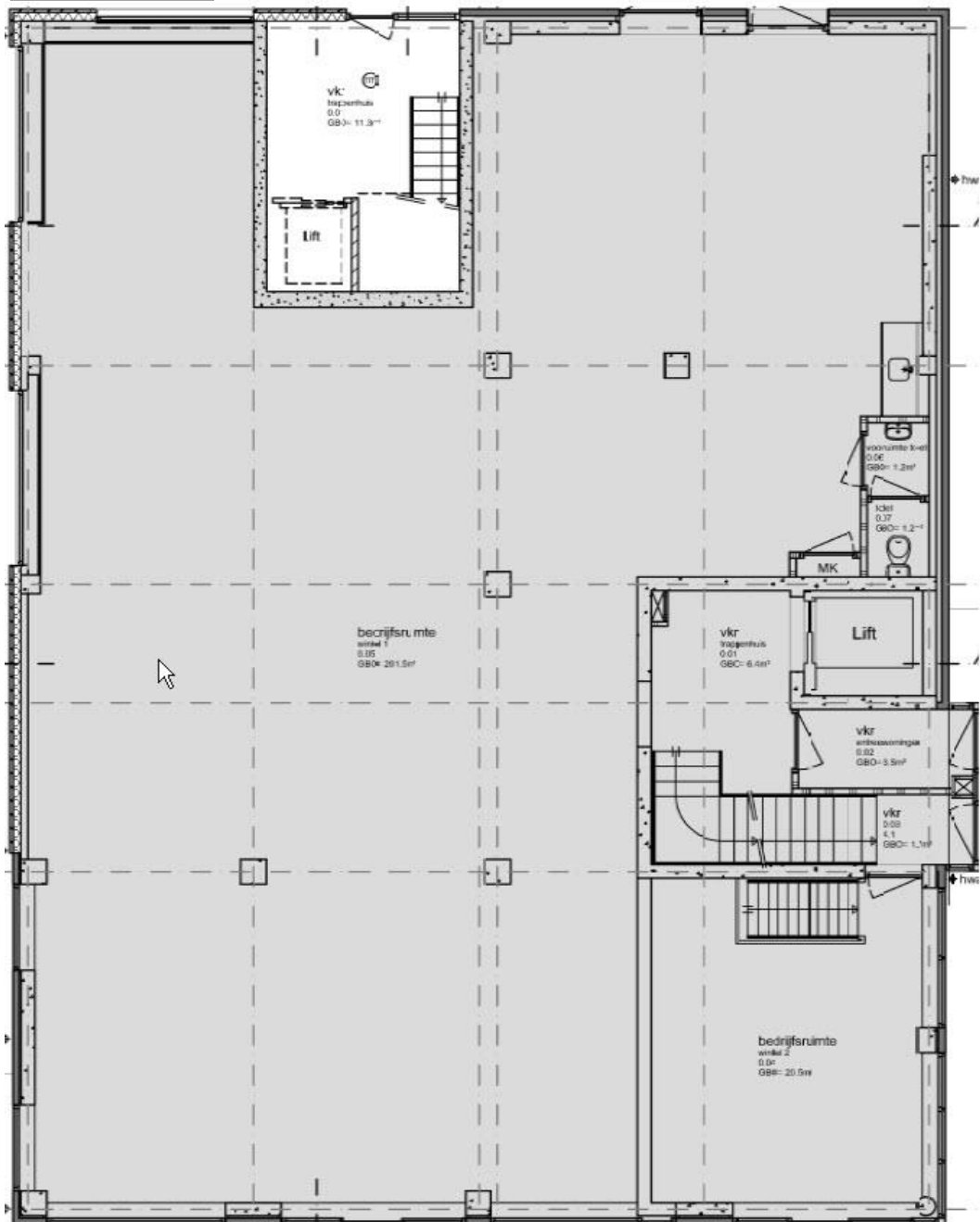
Begane grond
