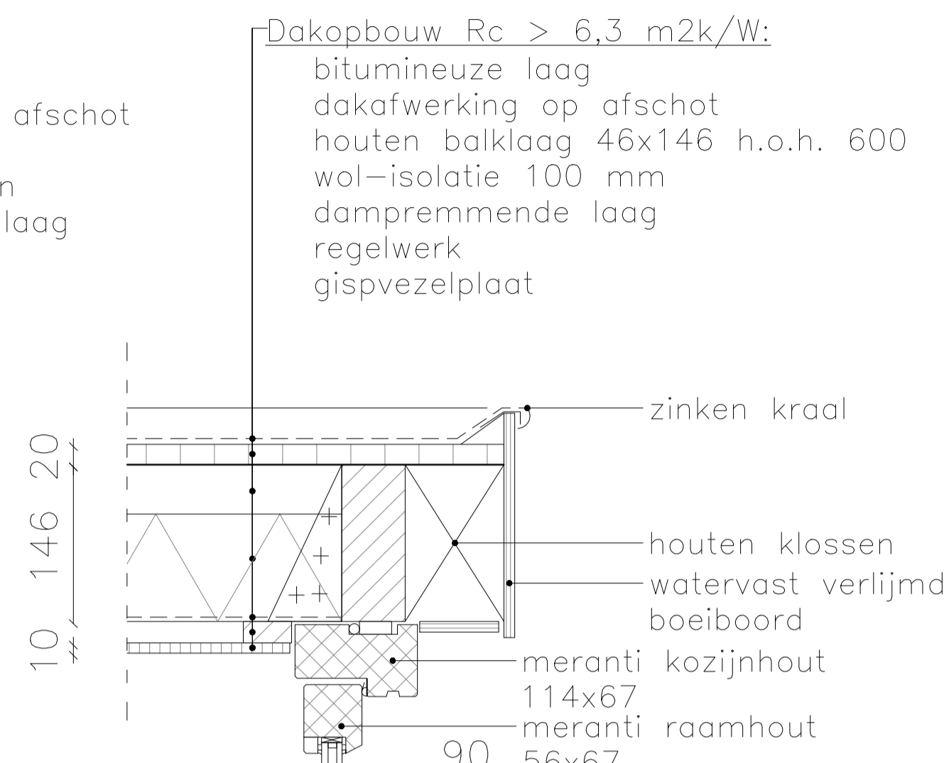
Detail 02 bovenaansluiting dakkapel kozijn
