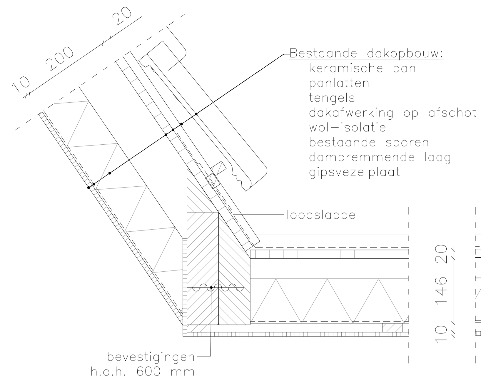
Detail 02 bovenaansluiting dakkapel kozijn
