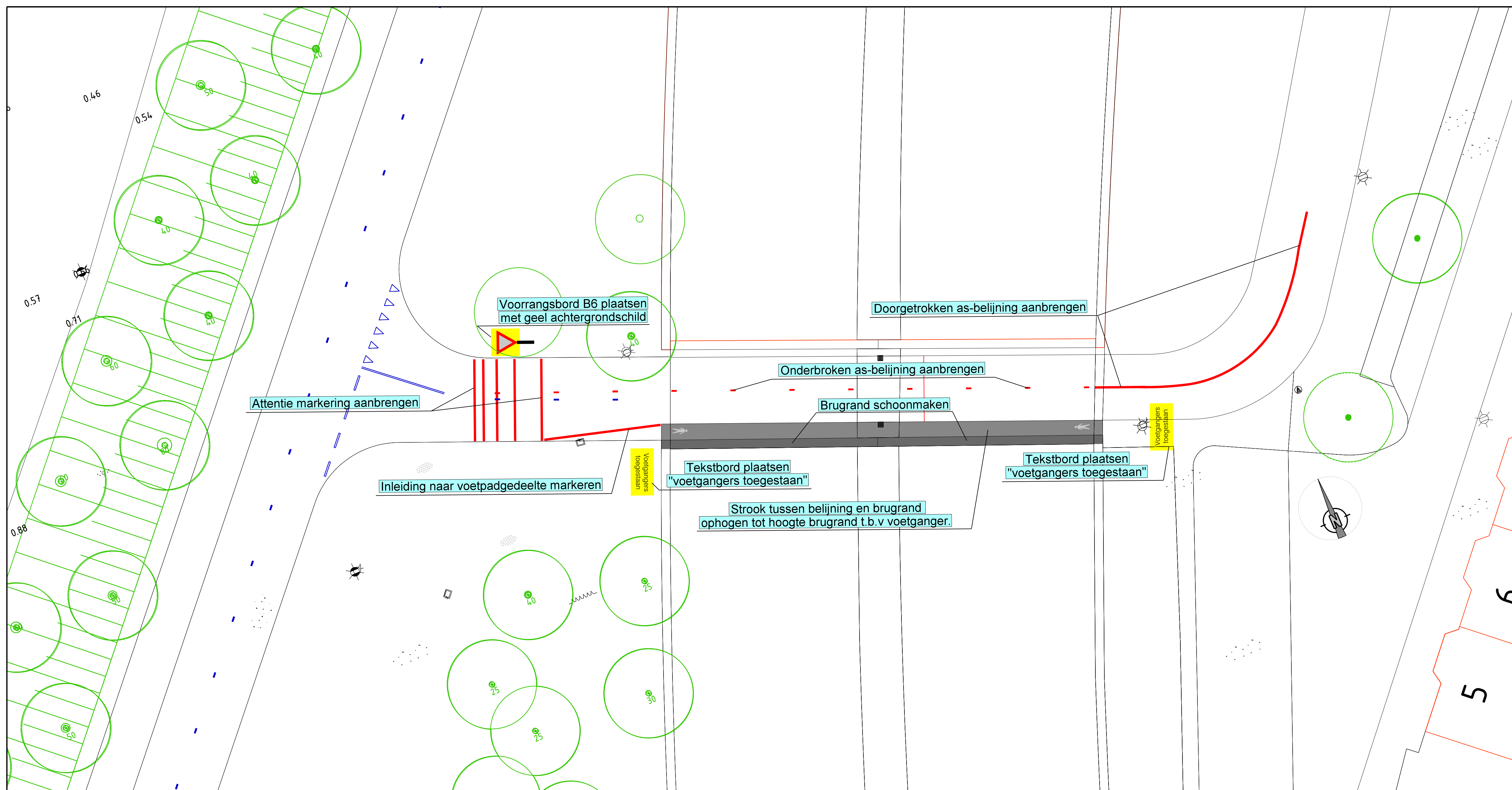
Aansluiting fietspad
