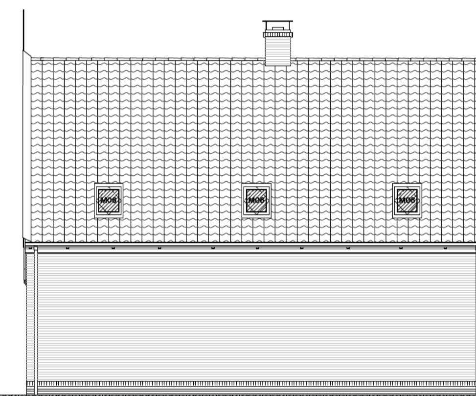
Rechterzijgevel
