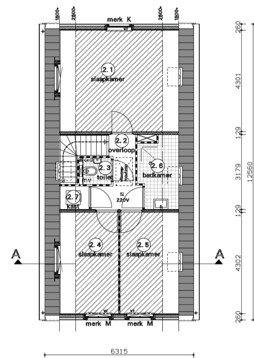
verdieping
