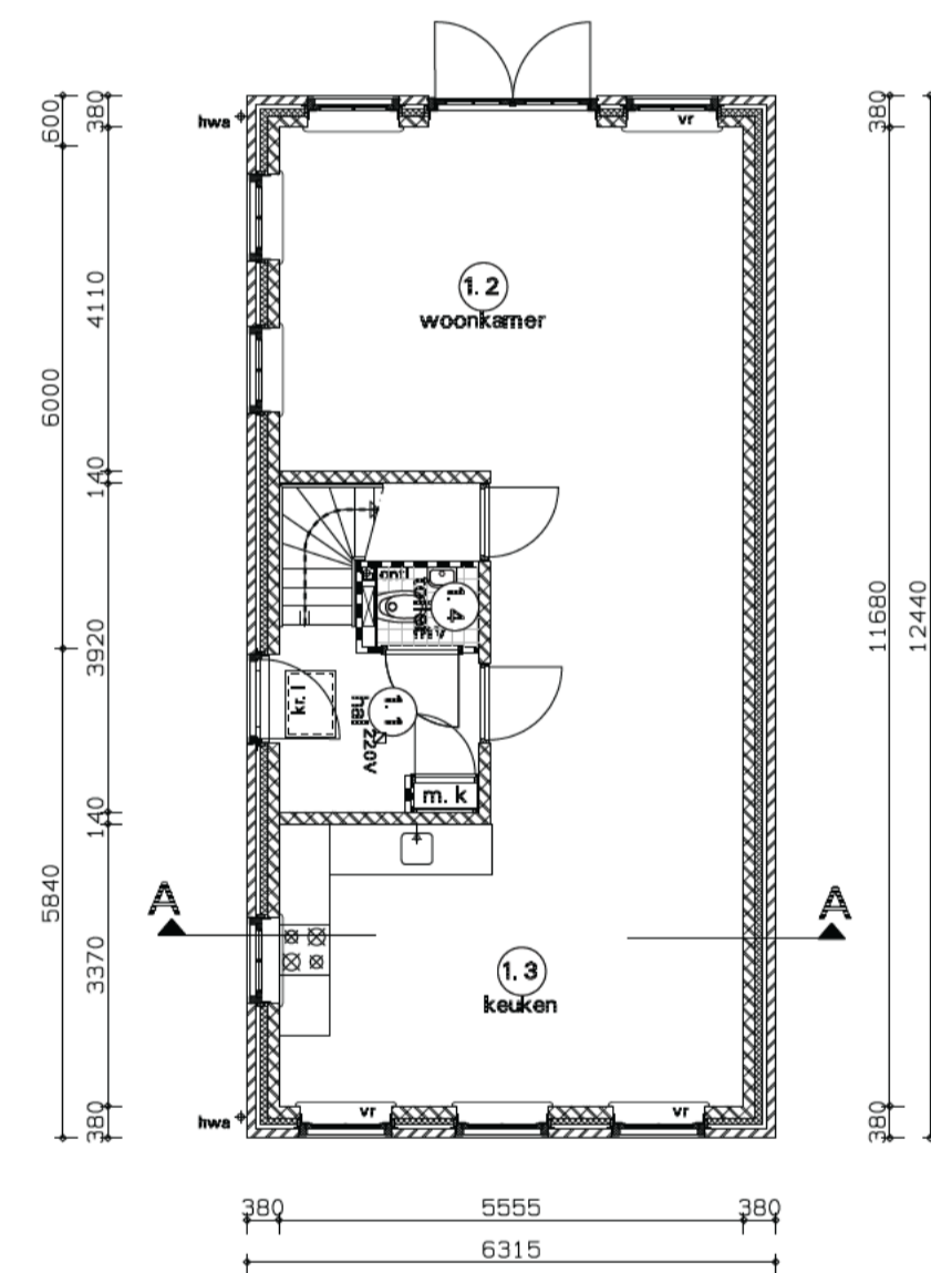
begane grond
